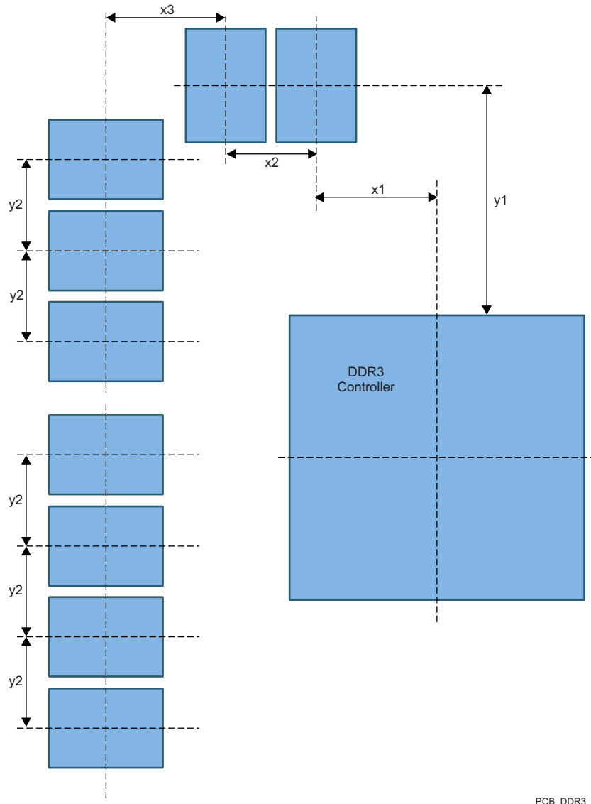
图 7-4. Placement Specifications
