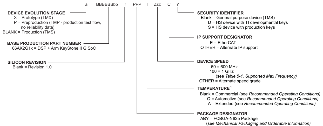
图 8-1. Device Nomenclature
