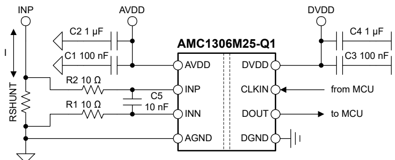
图 9-1. Decoupling of the AMC1306M25-Q1
