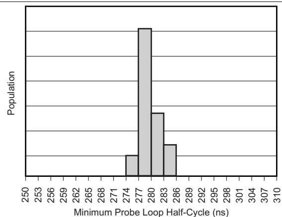
图 32. Oscillator Production Distribution
