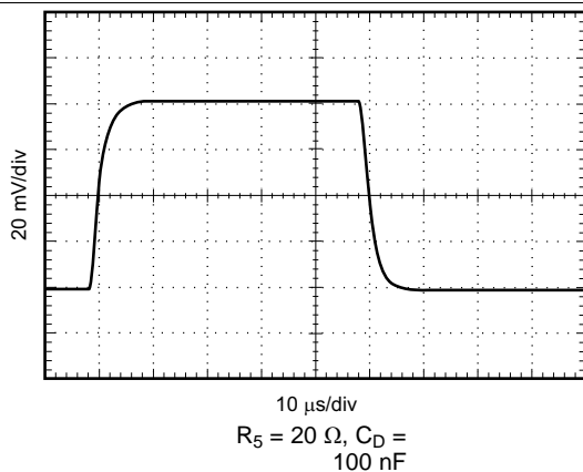
图 44. 图 44 Performance ( V_{OUT} )
