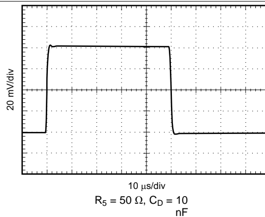
图 45. 图 45 Performance ( V_{OUT} )
