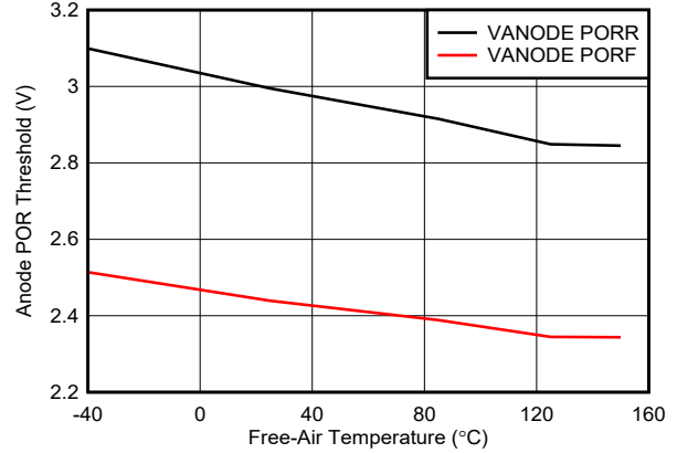
图 6-14. V_{ANODE} POR Threshold vs Temperature
