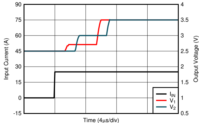
图 9-7. 对足以产生 1V 输出摆幅的输入电流阶跃的瞬态响应
