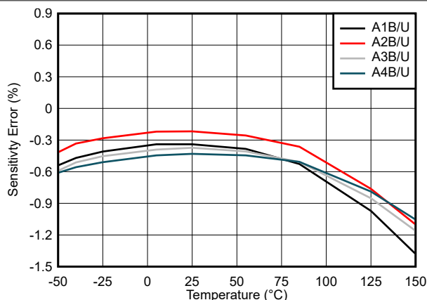
图 7-1. TMCS1108-Q1 灵敏度误差与温度间的关系
