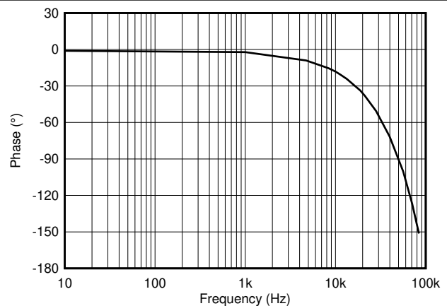
图 9-5. 归一化相位，所有型号
