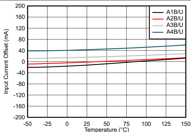
图 7-2. TMCS1108-Q1 输入失调电流与温度间的关系
