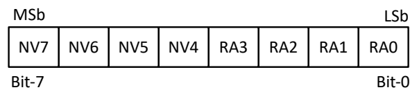
图 8-6. 电阻地址
