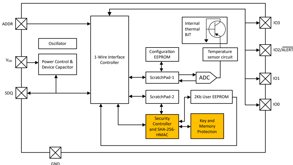
图 8-1. 功能方框图
