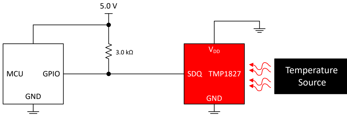
图 9-1. 总线供电应用
