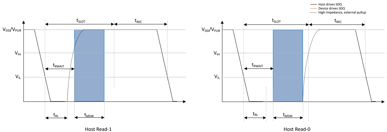
图 7-3. 读取时序图
