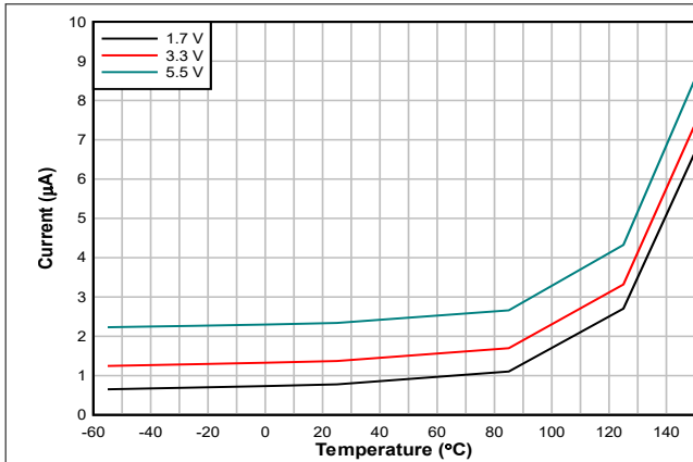
图 7-9. 关断电流与温度间的关系
