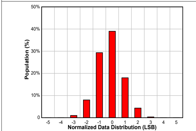
图 7-11. 转换时间为 5.5ms 和取平均值功能开启时的数据分布情况 (16 位格式)
