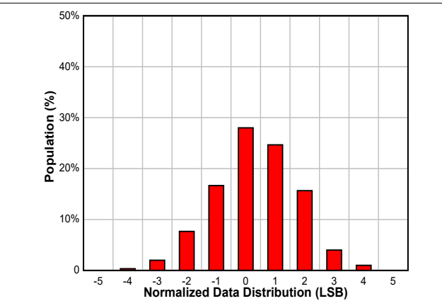
图 7-12. 转换时间为 3ms 和取平均值功能开启时的数据分布情况 (16 位格式)
