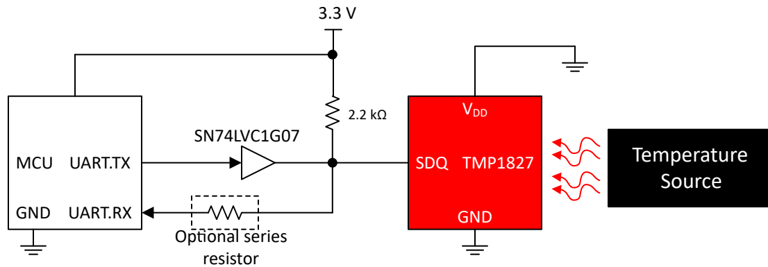
图 9-3. 使用 UART 进行连接 TMP1827
