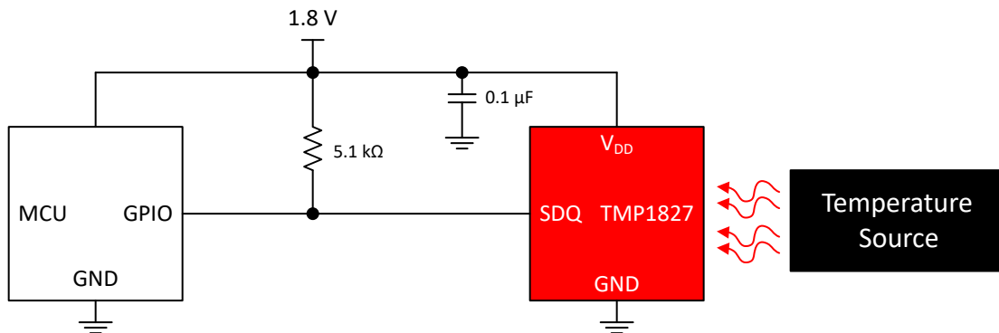
图 9-2. 电源供电类应用
