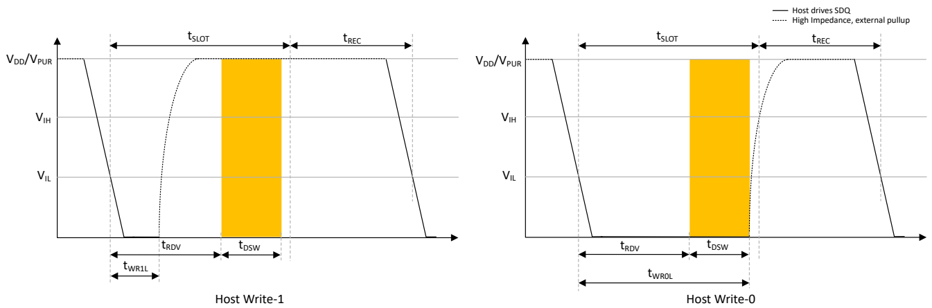
图 7-2. 写入时序图
