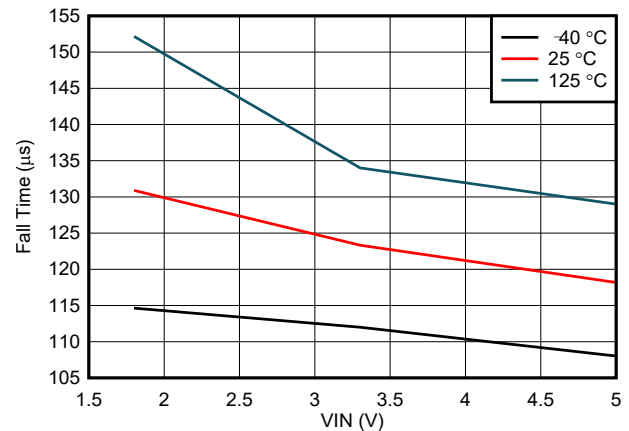
图 6-6. Fall Time vs Input Voltage
