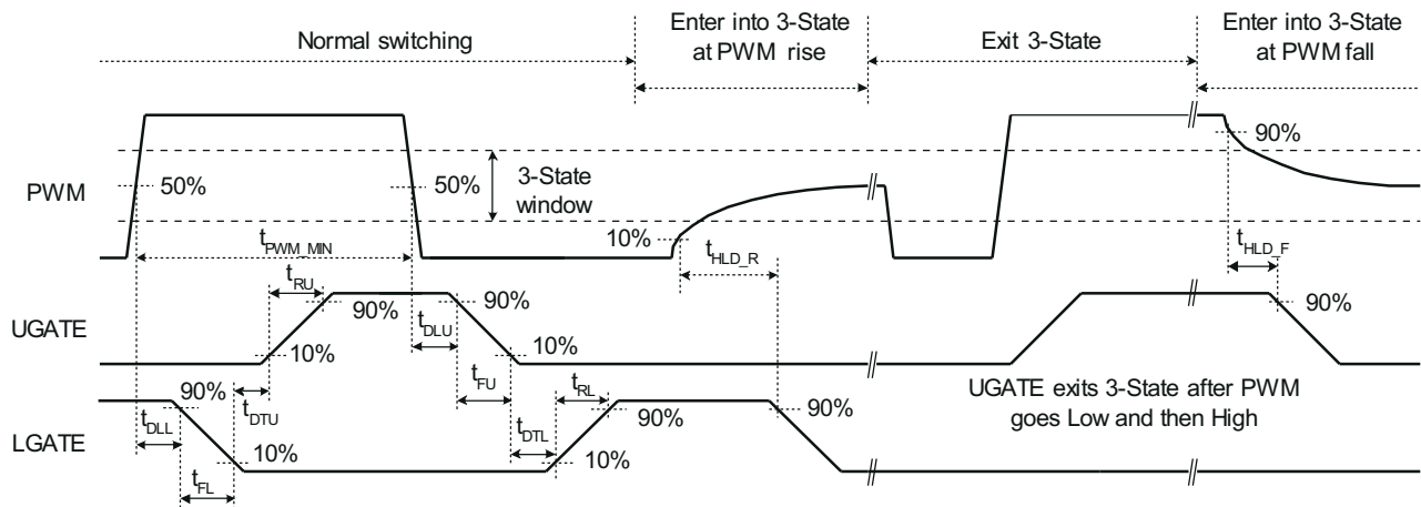
图 6-1. Timing Diagram
