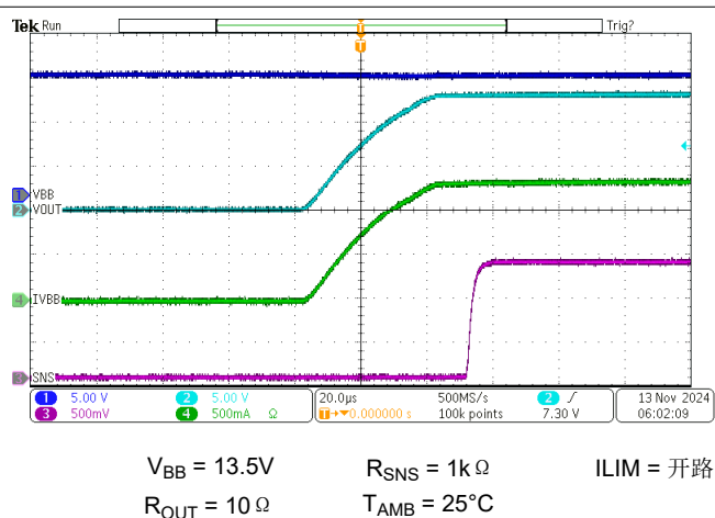
图 6-13. 开关导通
