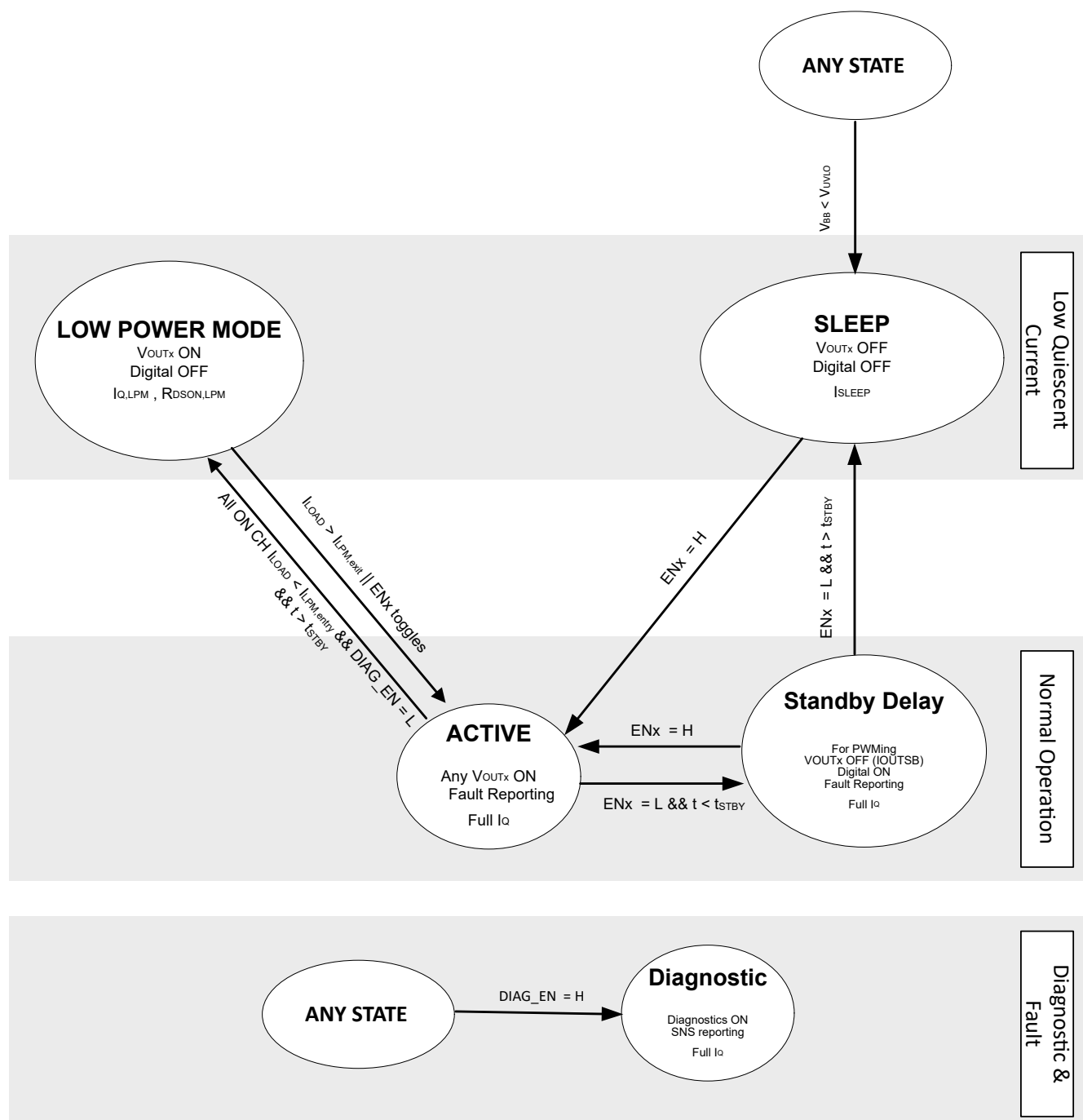
图 7-24. 状态图
