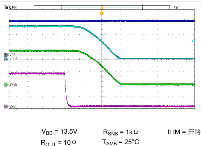
图 6-14. 开关关断
