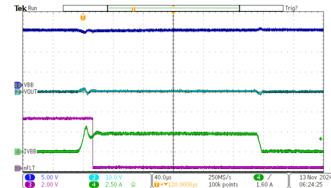
图 6-16. ILIM 开路时的永久短路行为
