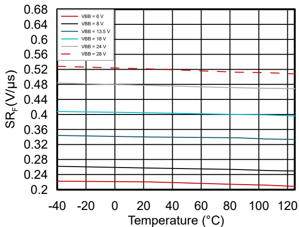
图 6-10. 在 V_{BB} 电压范围内 SR_F 与温度间的关系
