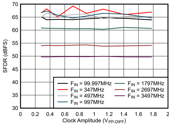
图 5-33. SFDR vs Clock Amplitude
