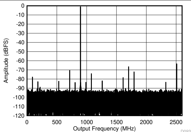
图 5-18. 双通道模式：897MHz 时的单音 FFT
