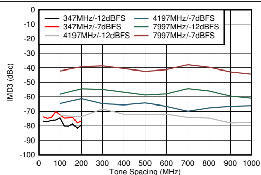
图 5-108. 双通道模式：IMD3 与频间间隔间的关系
