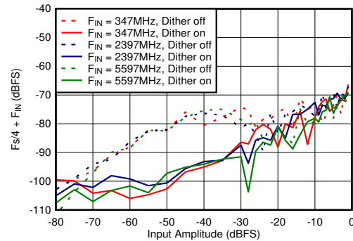
图 5-68. DES 模式： F_s/2 - F_{\text{IN}} 与输入振幅和抖动间的关系
