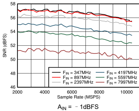
图 5-29. DES 模式：SNR 与采样率和输入频率间的关系
