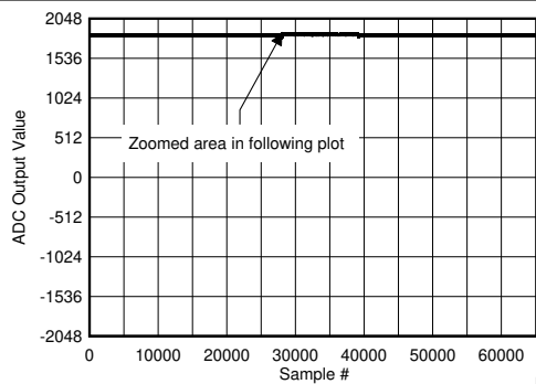
图 5-146. 后台校准内核转换 (直流信号)
