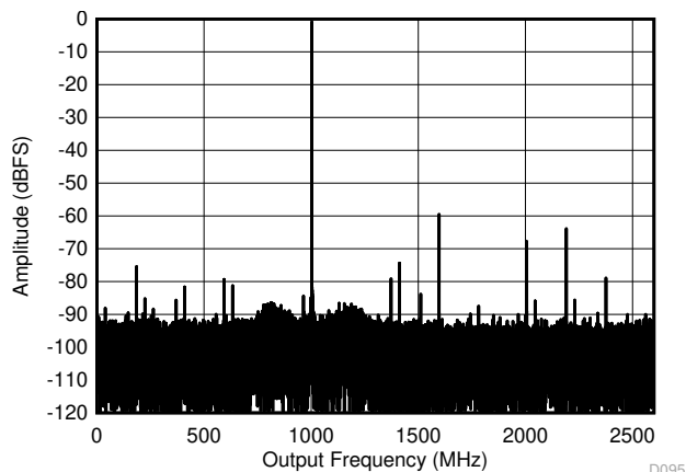
图 5-20. 双通道模式：4197MHz 时的单音 FFT
