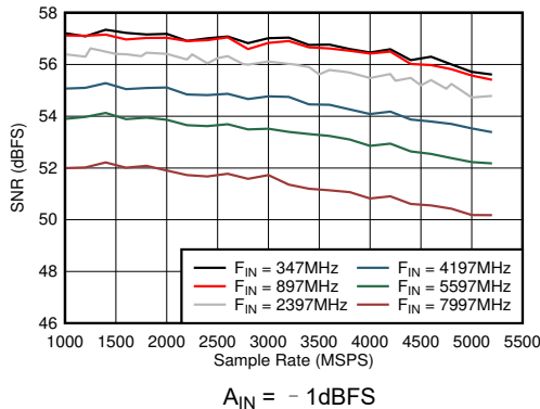
图 5-45. 双通道模式：SNR 与采样率和输入频率间的关系
