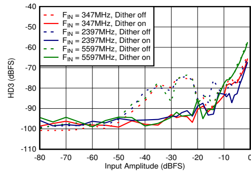
图 5-66. DES 模式：HD3 与输入振幅和抖动间的关系
