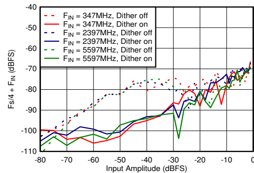
图 5-70. DES 模式： F_s/4 + F_{\text{IN}} 与输入振幅和抖动间的关系
