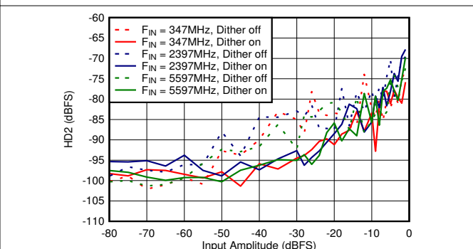
图 6-64. DES Mode: HD2 vs Input Amplitude and Dither
