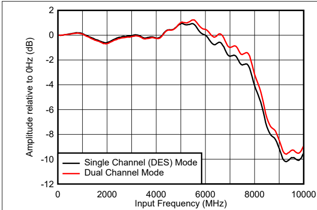
图 6-1. Input Amplitude vs Input Frequency
