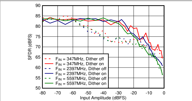
图 6-62. DES Mode: SFDR vs Input Amplitude and Dither
