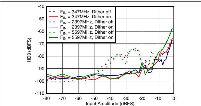
图 6-66. DES Mode: HD3 vs Input Amplitude and Dither
