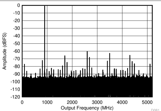
图 6-6. DES Mode: Single Tone FFT at 897 MHz
