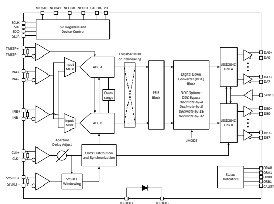
ADC12DJ5200-SP 方框图
