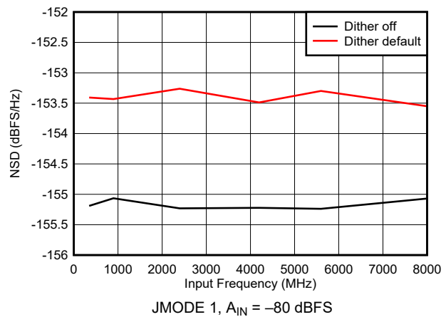
图 6-36. DES Mode: NSD vs Input Frequency
