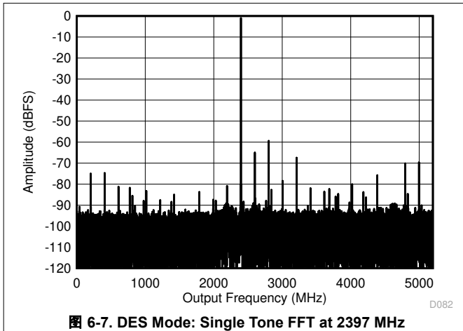
图 6-7. DES Mode: Single Tone FFT at 2397 MHz
