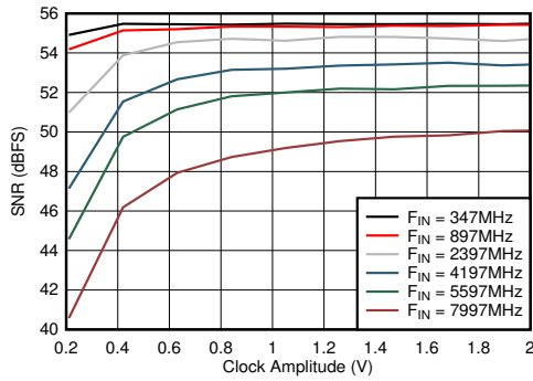
图 5-81. DES Mode: SNR vs Clock Amplitude
