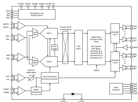
ADC12DJ5200RF 方框图
