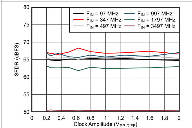
图 5-41. SFDR vs Clock Amplitude
