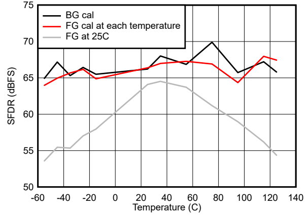
图 5-44. SFDR vs Temperature
