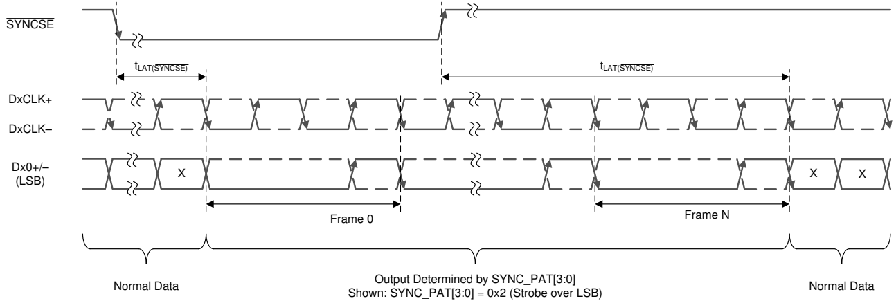
图 5-8. SYNCSE Timing Diagram
