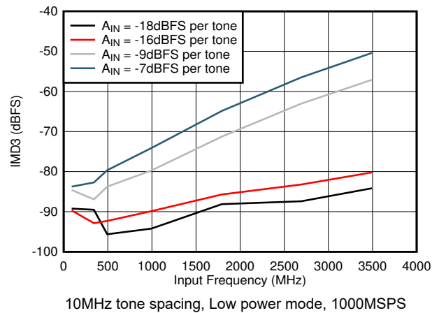
图 6-76. IMD3 vs F_{IN}
