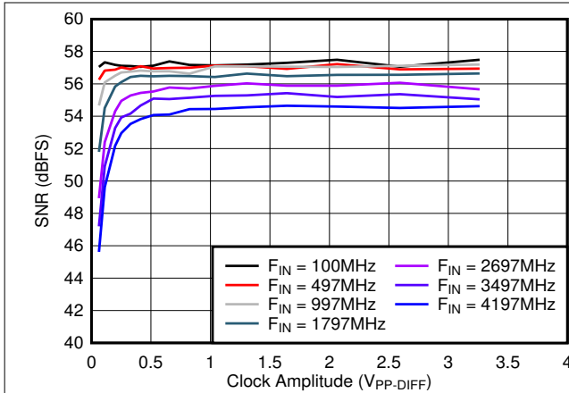
图 6-37. SNR vs A_{CLK}
