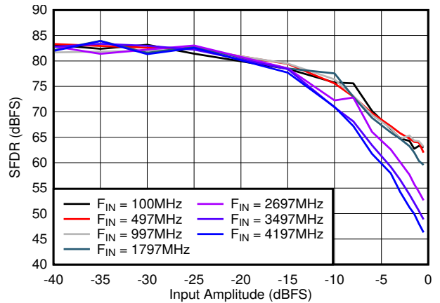
图 6-32. SFDR vs A_{IN}
