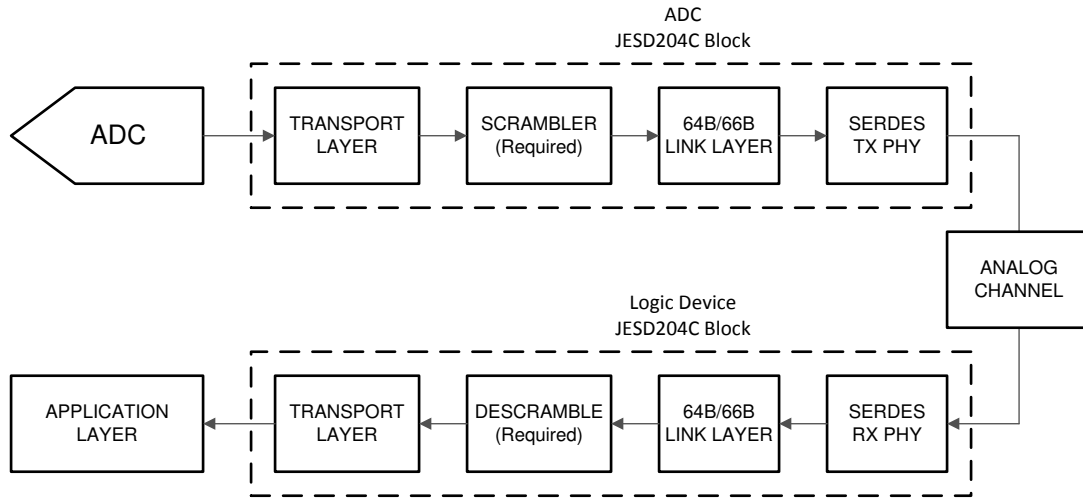
图 6-6. Simplified 64B/66B Encoded JESD204C Interface Diagram
