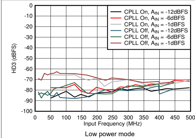
图 5-59. HD3 vs A_{IN} and C-PLL
