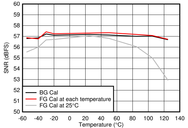
图 5-64. SNR vs Temperature
