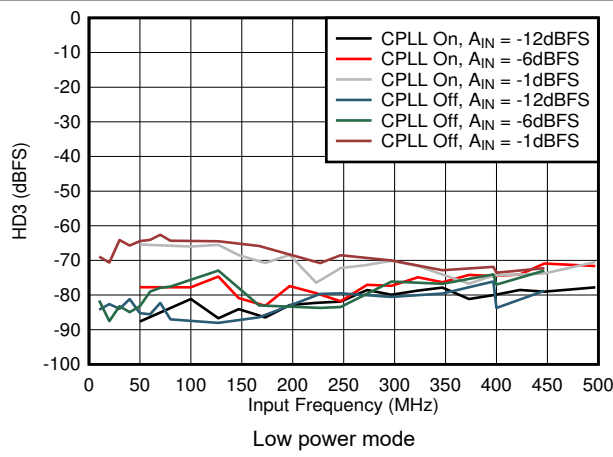
图 5-59. HD3 vs A_{IN} and C-PLL
