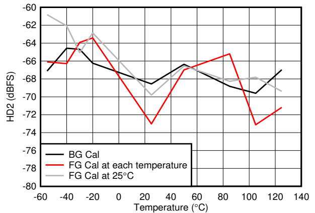
图 5-66. HD2 vs Temperature
