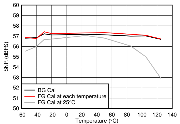
图 5-64. SNR vs Temperature
