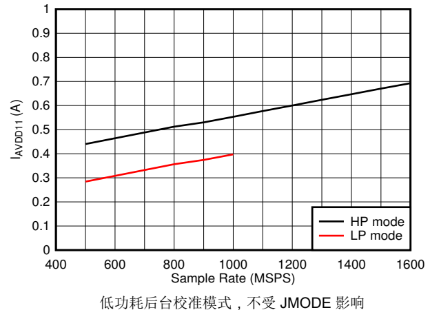
图 5-84. 四通道, I_{VA11} 与 F_S 间的关系
