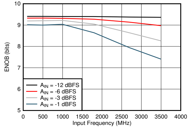
图 5-20. ENOB 与输入频率间的关系
