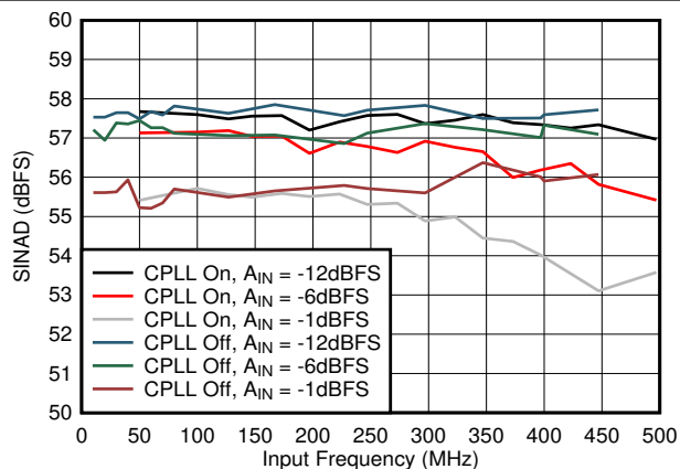
图 5-56. SINAD 与 A_{IN} 以及 C-PLL 间的关系
