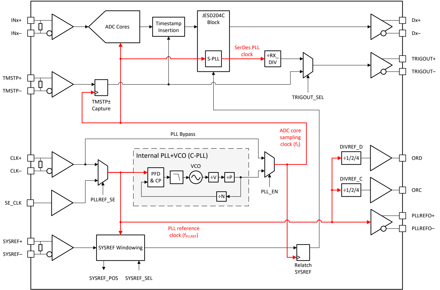
图 6-3. 时钟子系统
