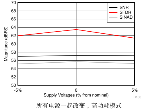
图 5-60. SNR、SFDR 和 SINAD 与电源电压间的关系
