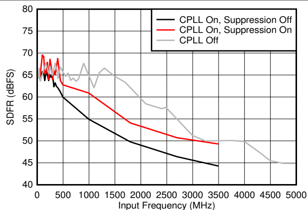
图 5-40. SFDR 与 F_{IN} 以及 C-PLL 模式间的关系
