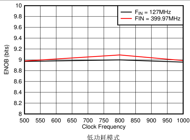
图 5-31. ENOB 与采样率间的关系
