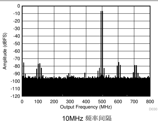
图 5-69. 498MHz 时的双音 FFT
