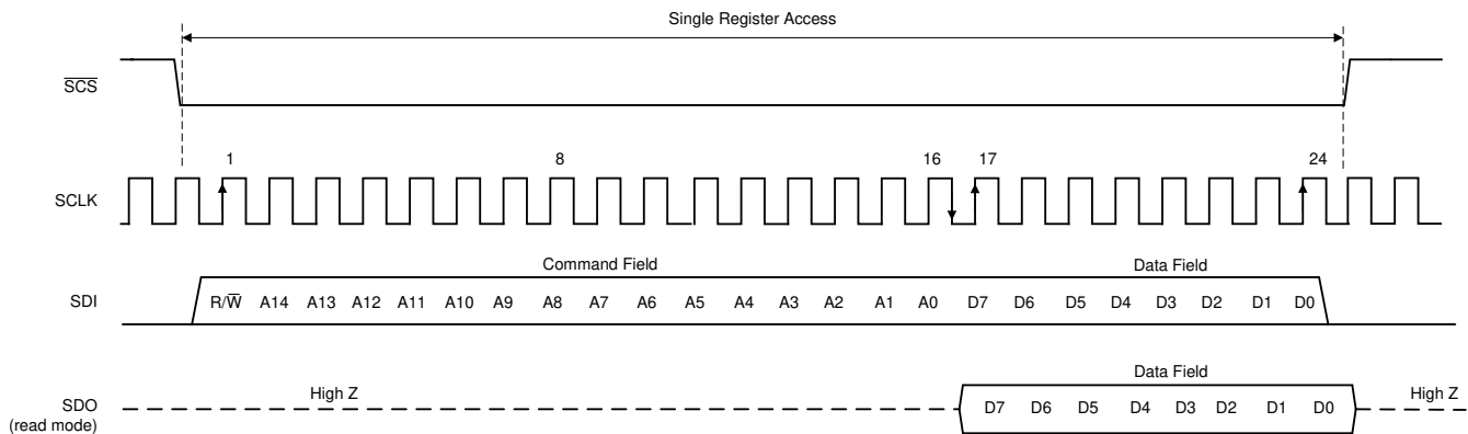
图 6-16. 串行接口协议：单读取/写入
