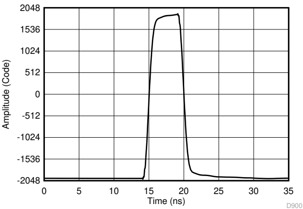
图 7-2. 使用测量等效 32GSPS 时所用的子采样技术测量脉冲
