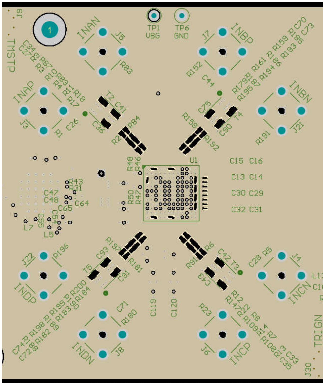
图 7-6. GND1 开孔可优化元件焊盘的阻抗
