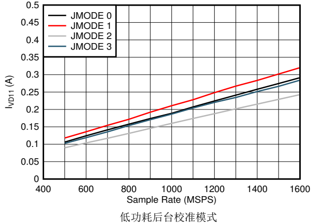
图 5-105. 单通道, I_{VD11} 与 F_S 以及 JMODE 0 - 3 间的关系
