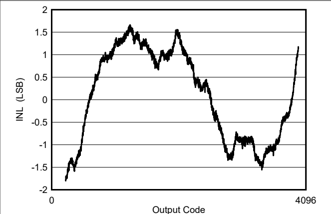
图 5-2. INL vs Code
