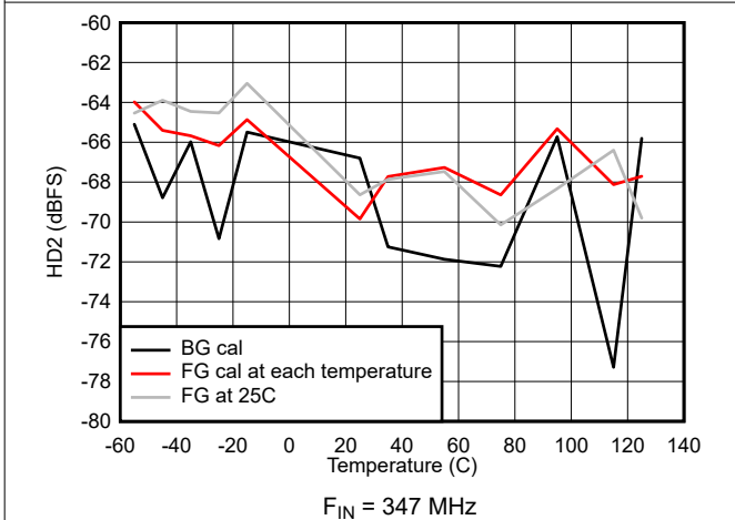
图 5-45. HD2 vs Temperature
