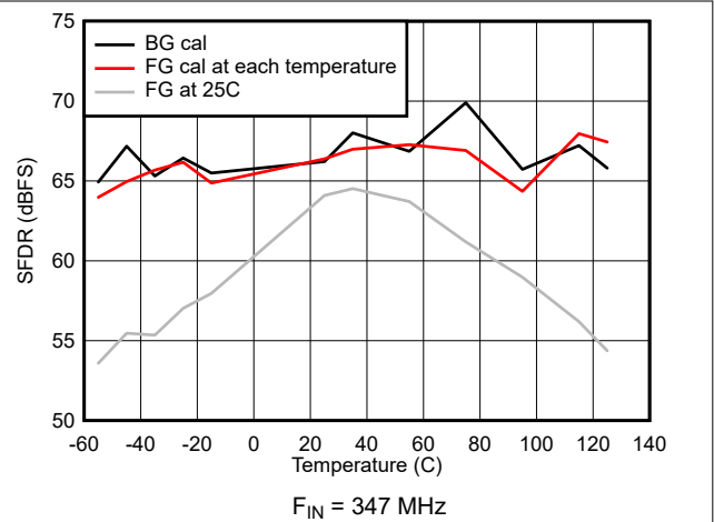
图 5-44. SFDR vs Temperature
