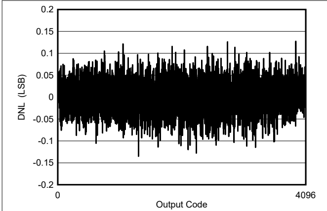
图 5-1. DNL vs Code
