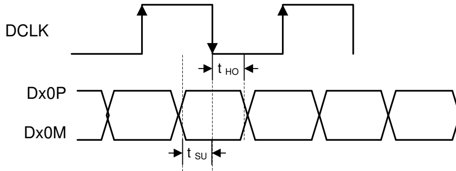
图 7-3. Setup and Hold Time
