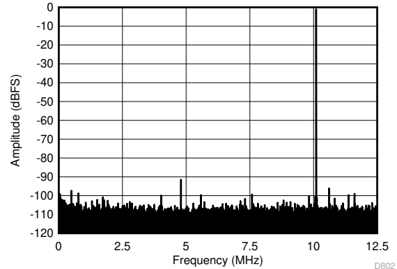
图 6-2. FFT for 10-MHz Input Signal (Dither Off)
