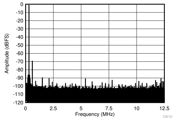
图 6-8. FFT for 270-MHz Input Signal (Dither Off)
