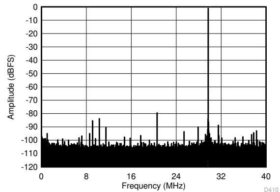
图 6-68. FFT for 270-MHz Input Signal (Dither Off)
