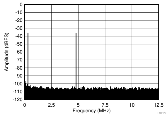
图 6-10. FFT for 450-MHz Input Signal (Dither Off)
