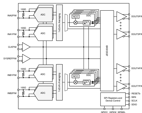
方框图
