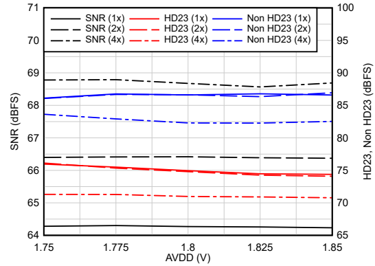
图 6-40. AC Performance vs AVDD18
