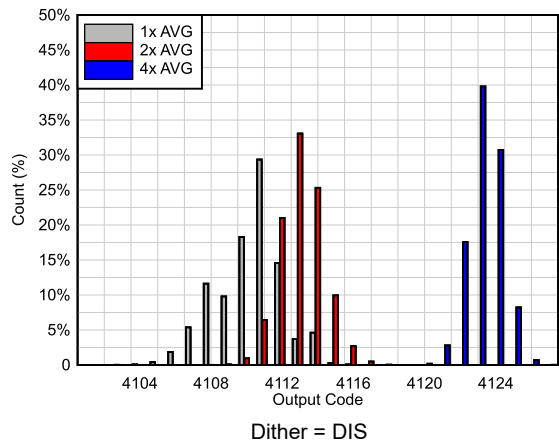
图 6-45. DC Offset Histogram
