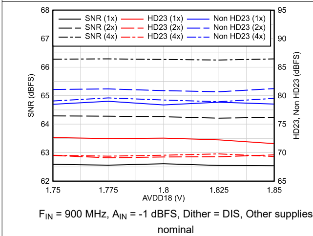
图 6-37. AC Performance vs AVDD18
