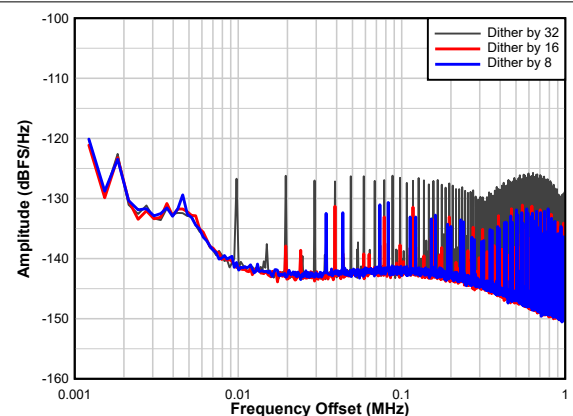
图 7-9. Dither vs Dither Divider Setting
