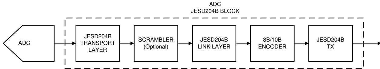
图 7-41. JESD204B Block Diagram
