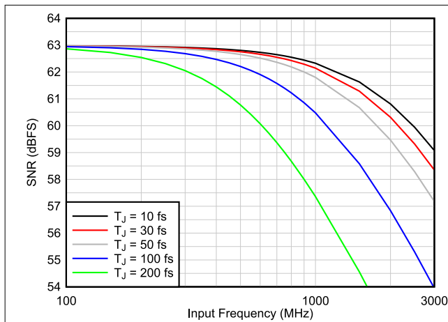
图 7-2. SNR vs T Jitter vs F IN (1x AVG)
