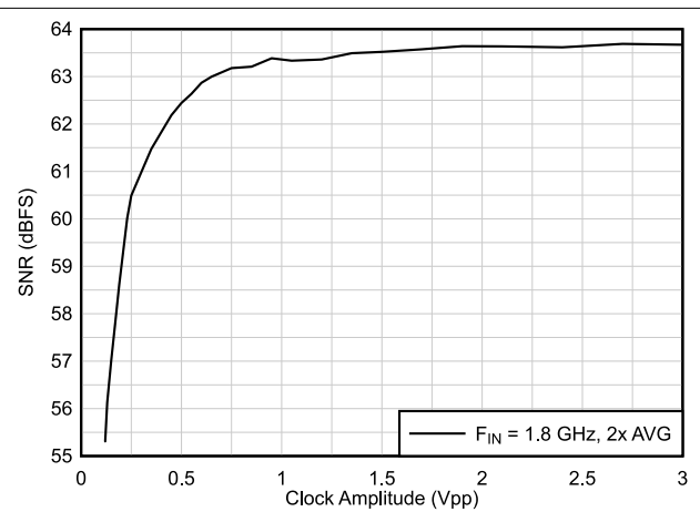
图 7-3. SNR vs Clock Amplitude
