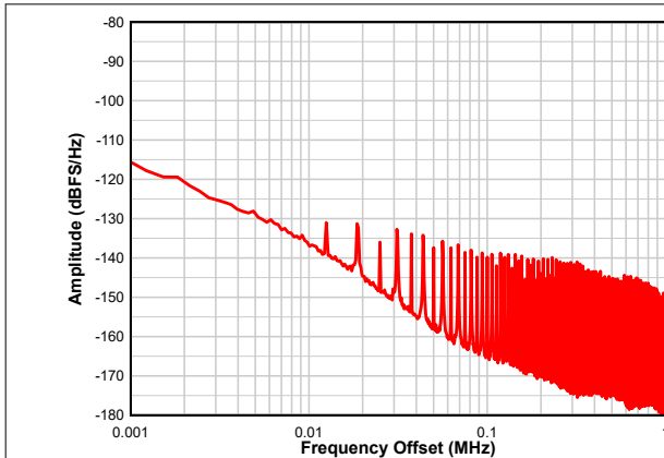
图 6-8. Dither Close-Up
