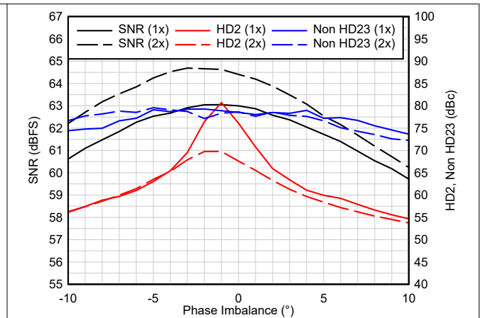
图 6-4. Phase Imbalance - 2.6 GSPS
