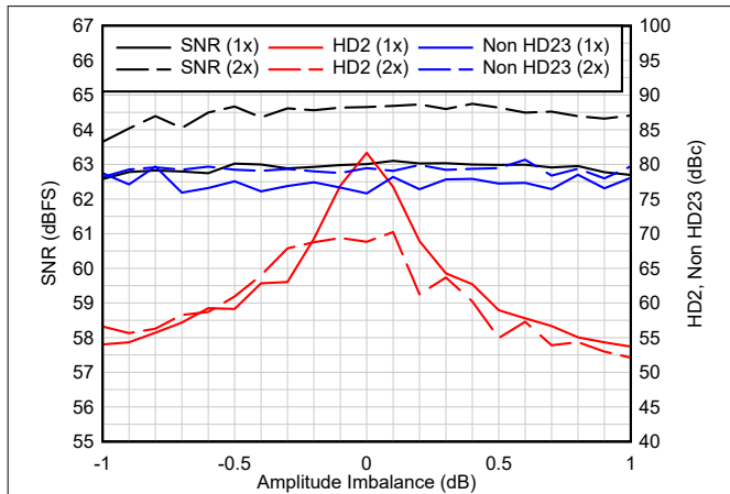
图 6-3. Amplitude Imbalance - 2.6 GSPS
