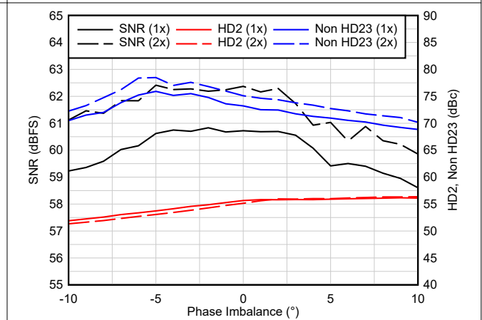
图 6-6. Phase Imbalance - 3.0 GSPS
