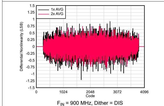
图 5-39. DNL vs Code
