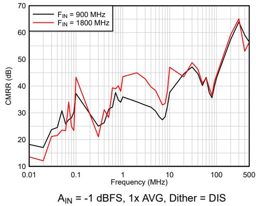
图 5-41. CMRR
