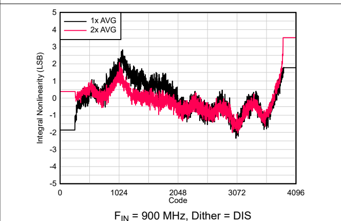
图 5-38. INL vs Code
