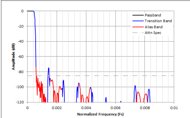
图 8-41. /1024 复数抽取滤波器响应
