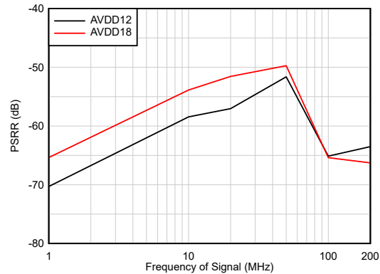
图 9-9. 电源抑制比 (PSRR) 与频率间的关系
