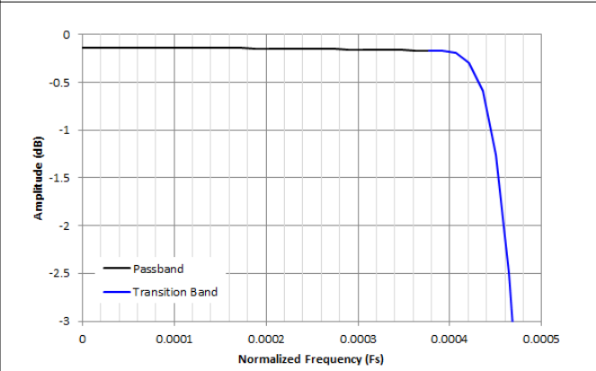
图 8-42. /1024 抽取通带纹波响应
