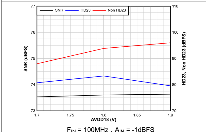
图 6-47. 交流性能与 AVDD18 间的关系
