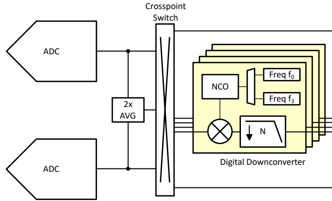
内部数字下变频器
