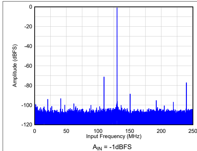
图 9-4. FFT1 : DDC 旁路
