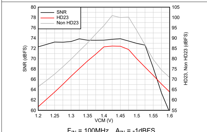
图 6-49. 交流性能与 VCM 间的关系
