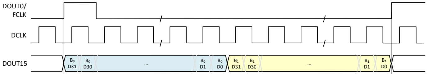
图 8-57. 示例 2 的 SLVDS 帧组装
