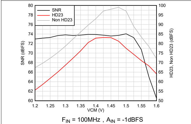
图 6-21. 交流性能与 VCM 间的关系
