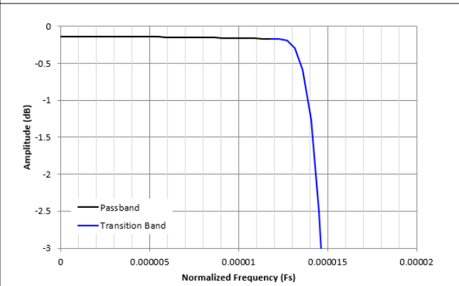
图 8-52. /32768 抽取通带纹波响应
