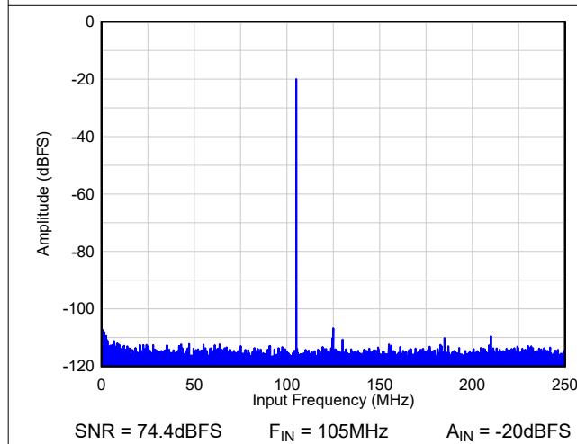
图 8-73. FFT - 无 AVG
