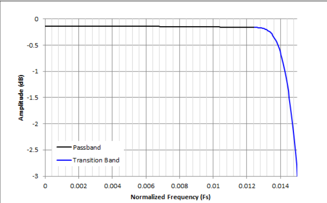
图 8-32. /32 抽取通带纹波响应
