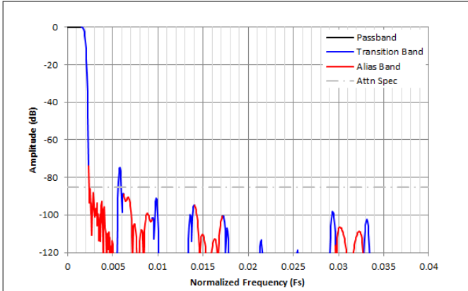
图 8-37. /256 复数抽取滤波器响应
