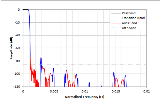
图 8-39. /512 复数抽取滤波器响应
