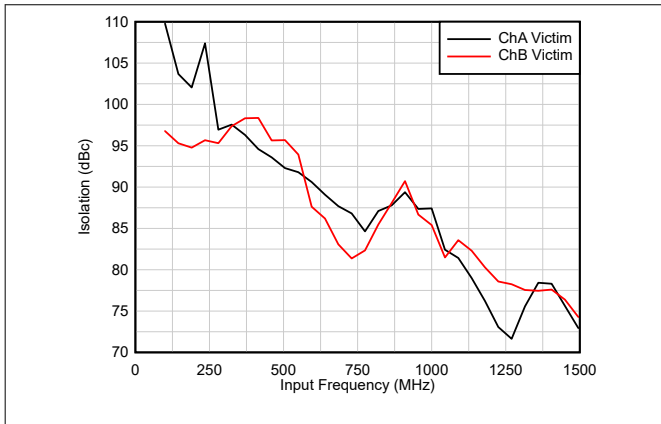
图 6-45. 隔离与 F_{IN} 间的关系
