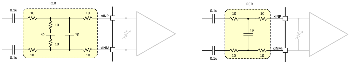
图 8-7. F_{IN} < 500\text{MHz} (左) 和 F_{IN} > 500\text{MHz} (右) 的外部 RCR
