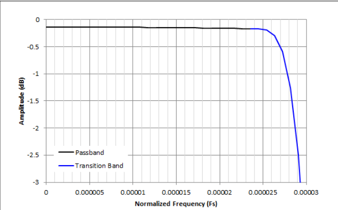
图 8-50. /16384 抽取通带纹波响应
