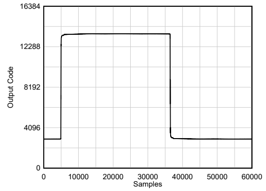
图 6-26. 脉冲响应
