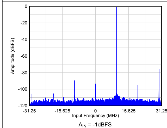
图 9-6. FFT3 : /8 抽取
