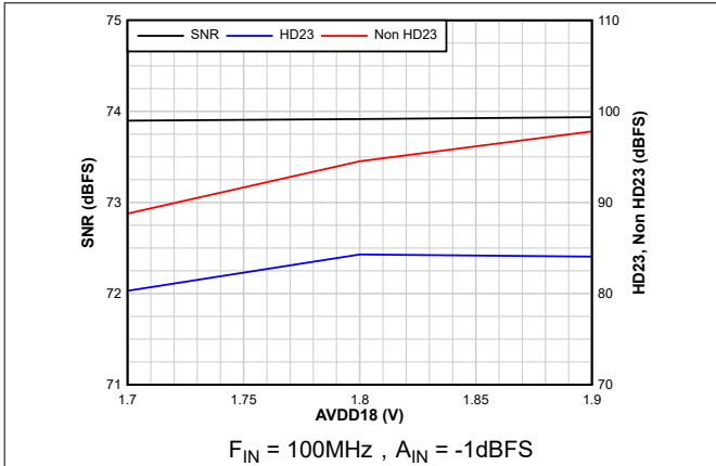
图 6-19. 交流性能与 AVDD18 间的关系
