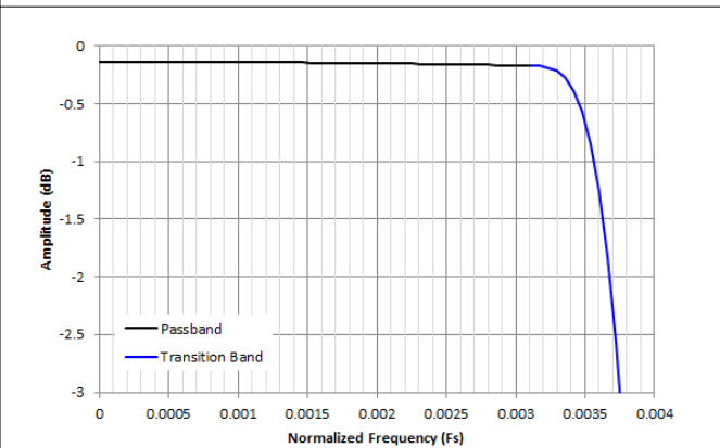
图 8-36. /128 抽取通带纹波响应
