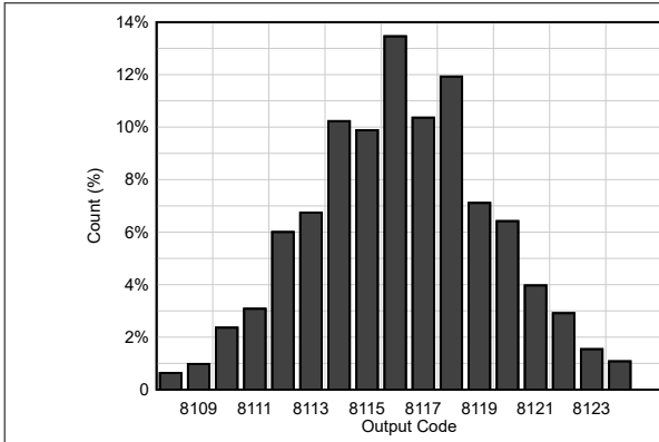
图 6-25. 直流偏移直方图
