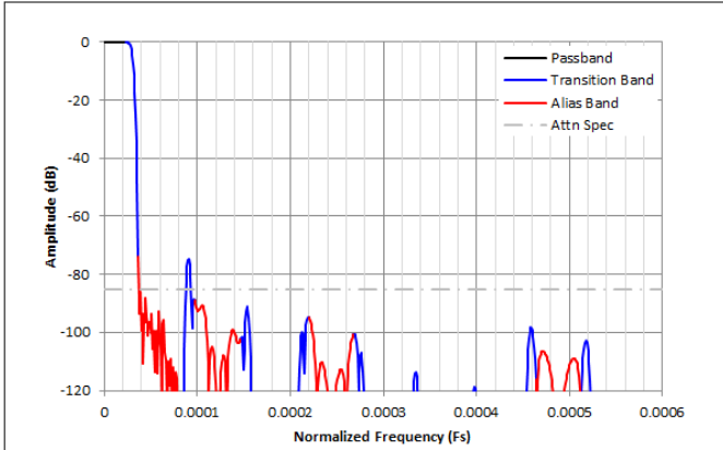
图 8-49. /16384 复数抽取滤波器响应
