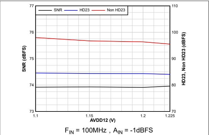
图 6-20. 交流性能与 AVDD12 间的关系
