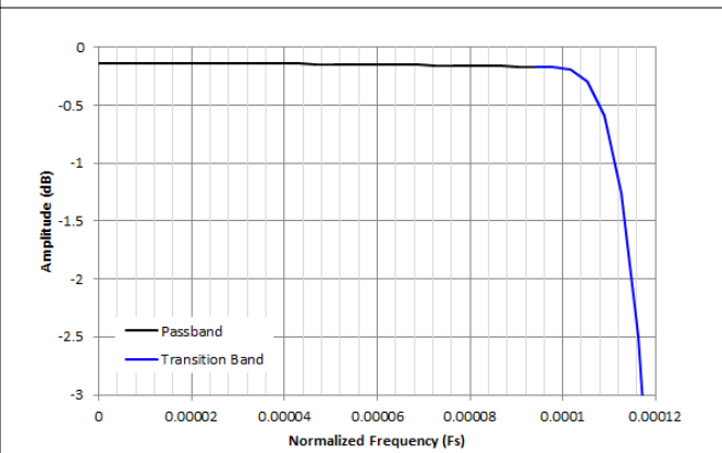
图 8-46. /4096 抽取通带纹波响应
