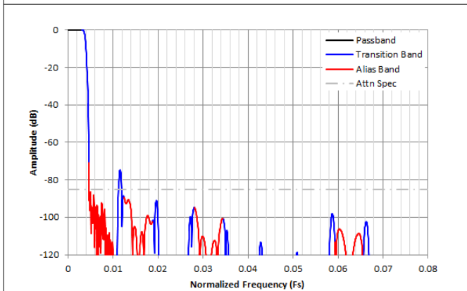
图 8-35. /128 复数抽取滤波器响应
