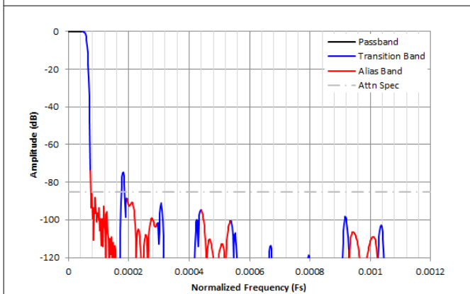
图 8-47. /8192 复数抽取滤波器响应
