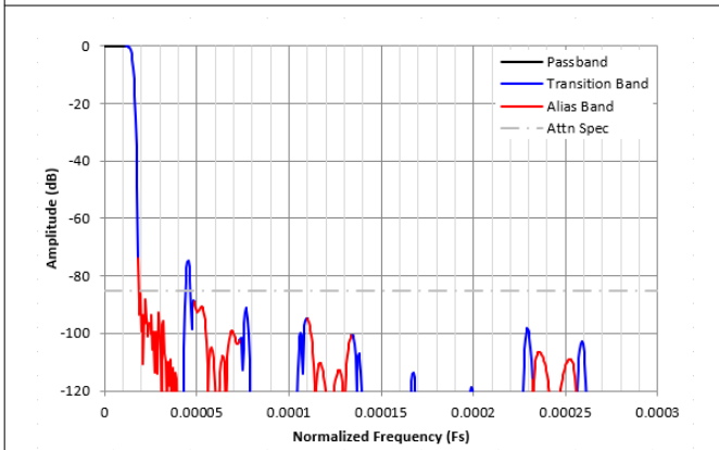
图 8-51. /32768 复数抽取滤波器响应
