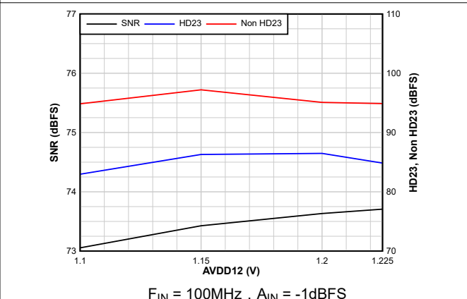
图 6-48. 交流性能与 AVDD12 间的关系
