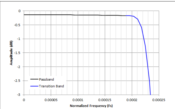
图 8-44. /2048 抽取通带纹波响应
