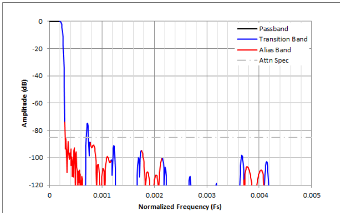
图 8-43. /2048 复数抽取滤波器响应
