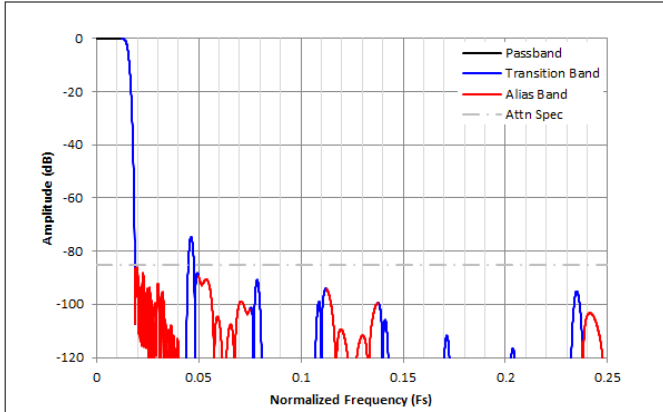
图 8-31. /32 复数抽取滤波器响应
