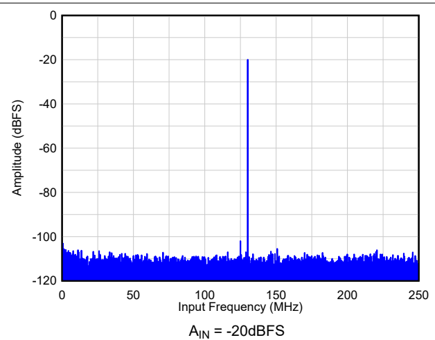
图 9-5. FFT2 : DDC 旁路
