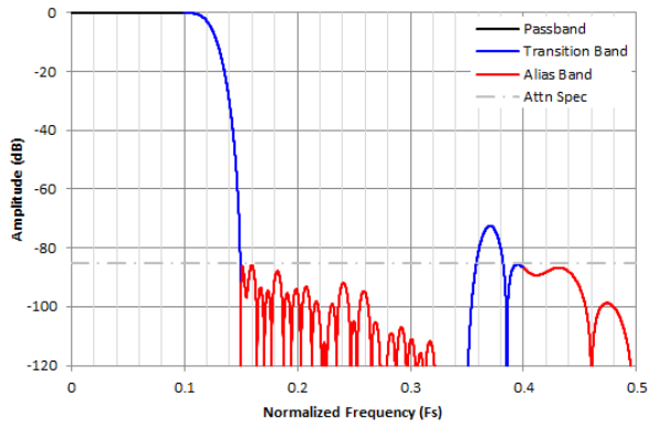
图 8-25. /4 复数抽取滤波器响应
