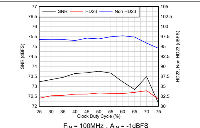
图 6-46. 交流性能与时钟占空比间的关系
