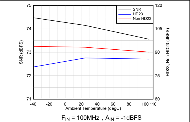
图 6-22. 交流性能与温度间的关系
