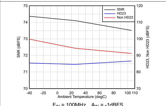
图 6-50. 交流性能与温度间的关系
