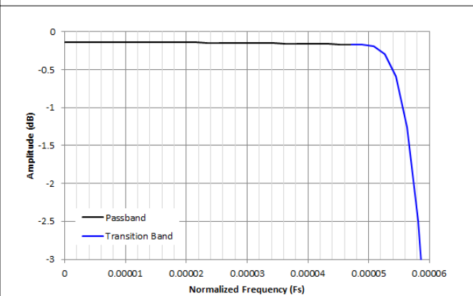
图 8-48. /8192 抽取通带纹波响应
