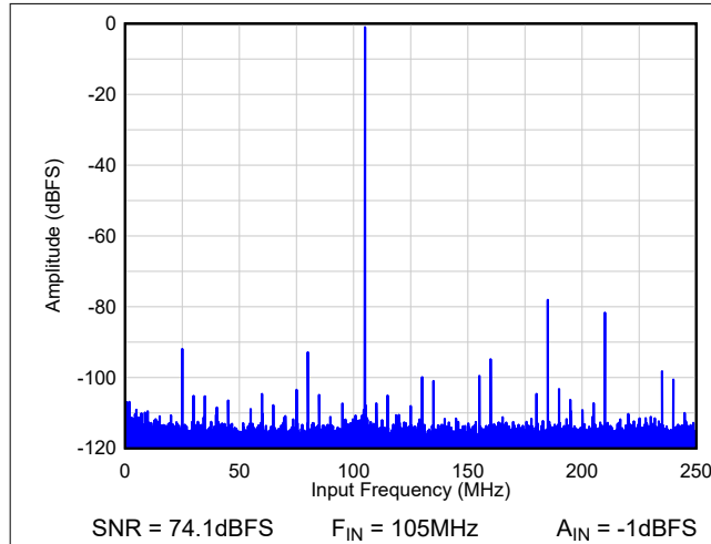
图 8-71. FFT - 无 AVG
