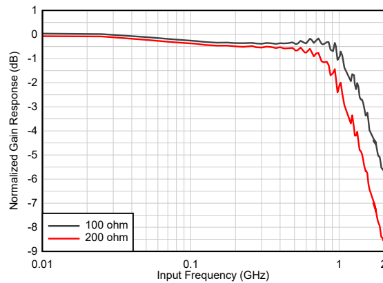
图 8-6. 100 Ω 和 200 Ω 内部端接的全功率输入带宽
