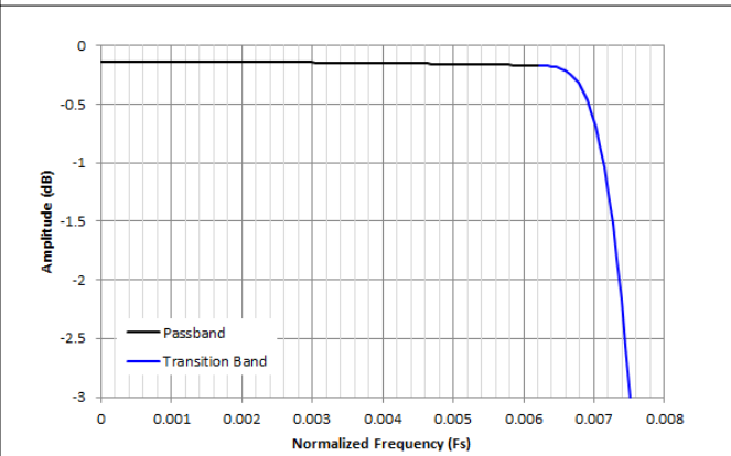
图 8-34. /64 复数抽取通带纹波响应
