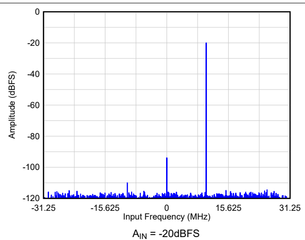
图 9-7. FFT4 : /8 抽取
