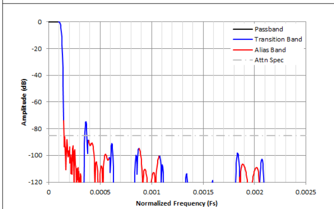
图 8-45. /4096 复数抽取滤波器响应
