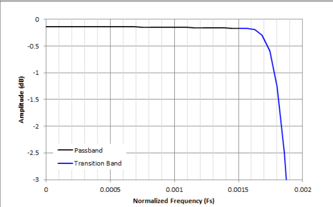
图 8-39. /256 抽取通带纹波响应
