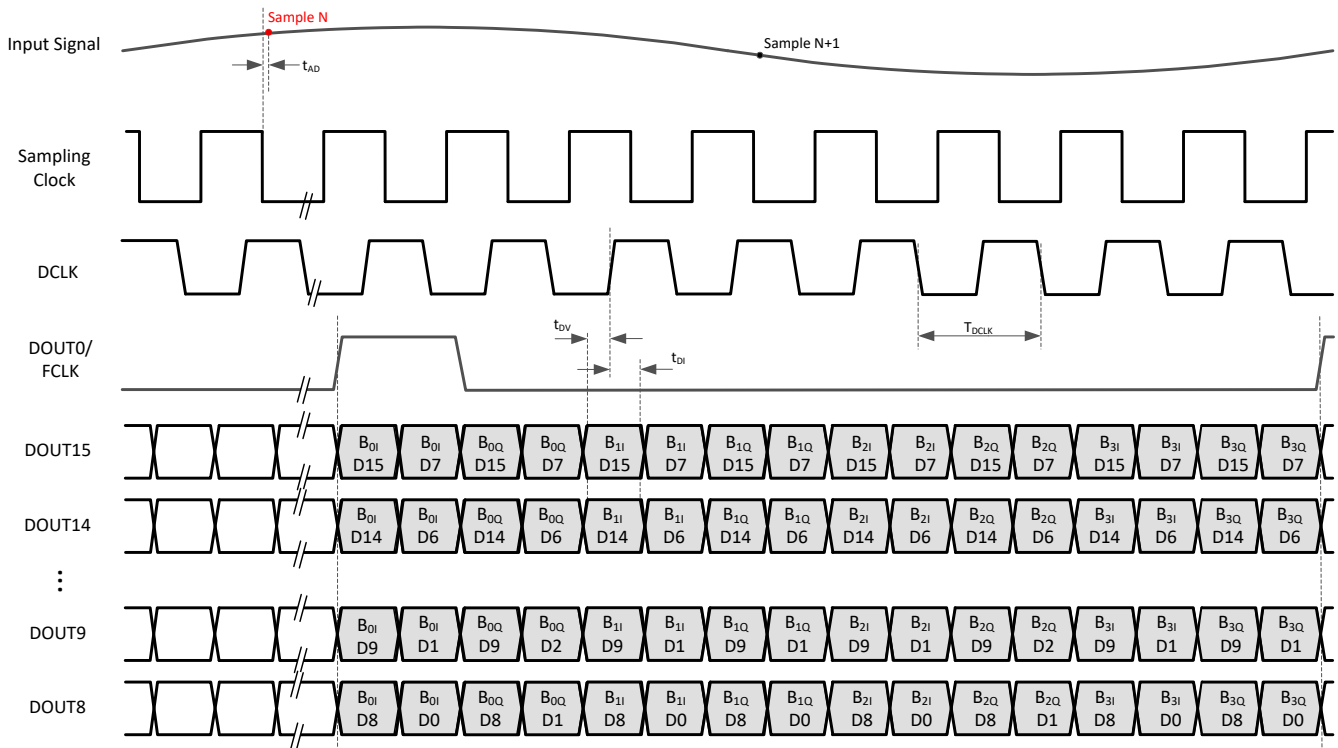
图 7-2. 时序图：串行 LVDS (示例：四频带、16 位、/8 复数抽取)
