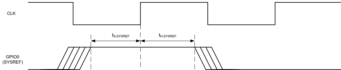
图 8-16. 时序：外部同步输入
