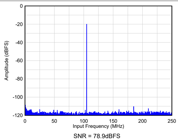
图 8-75. FFT - 2x AVG ( F_{IN} = 105\text{MHz} , A_{IN} = -20\text{dBFS} )
