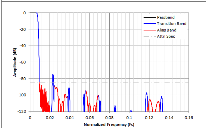
图 8-34. /64 复数抽取滤波器响应
