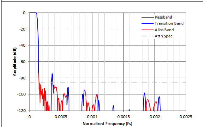
图 8-46. /4096 复数抽取滤波器响应
