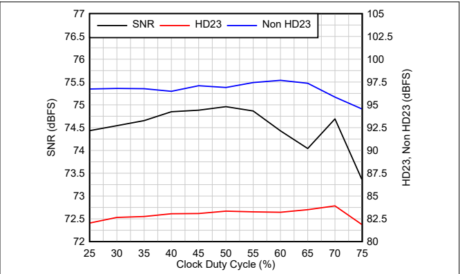
图 6-46. 交流性能与时钟占空比间的关系
