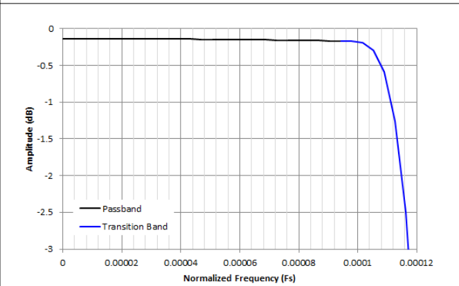
图 8-47. /4096 抽取通带纹波响应
