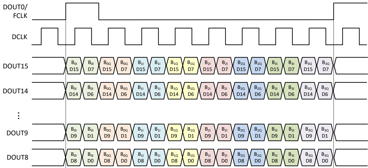
图 8-60. 示例 4 的 SLVDS 帧组装
