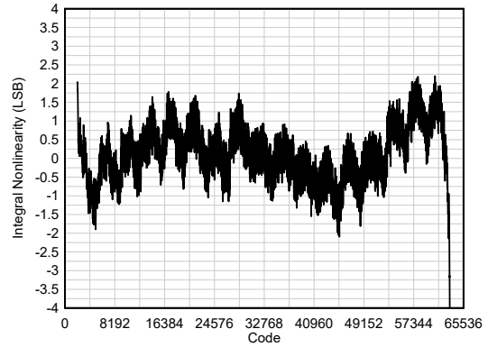
图 6-52. INL
