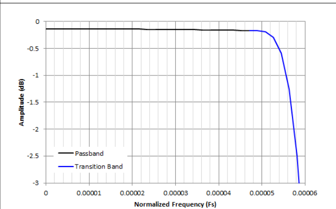
图 8-49. /8192 抽取通带纹波响应
