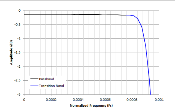
图 8-41. /512 抽取通带纹波响应
