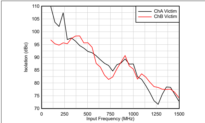
图 6-45. 隔离与 F_{IN} 间的关系
