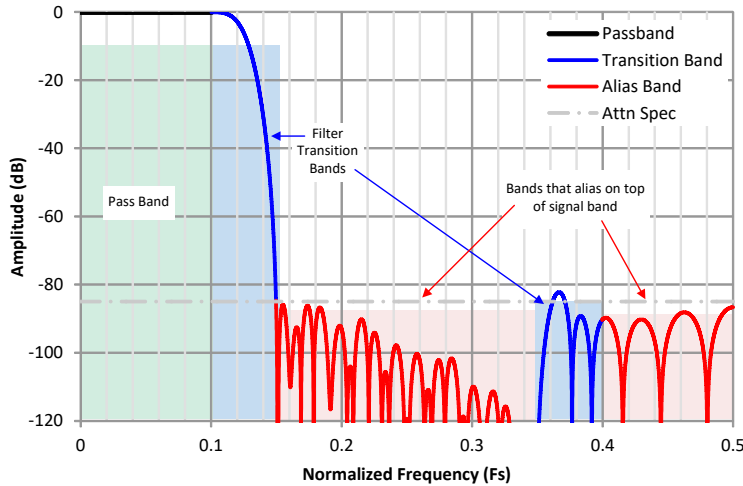
图 8-23. 抽取滤波器图的解释
