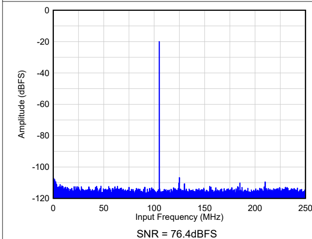
图 8-74. FFT - 无 AVG ( F_{IN} = 105\text{MHz} , A_{IN} = -20\text{dBFS} )
