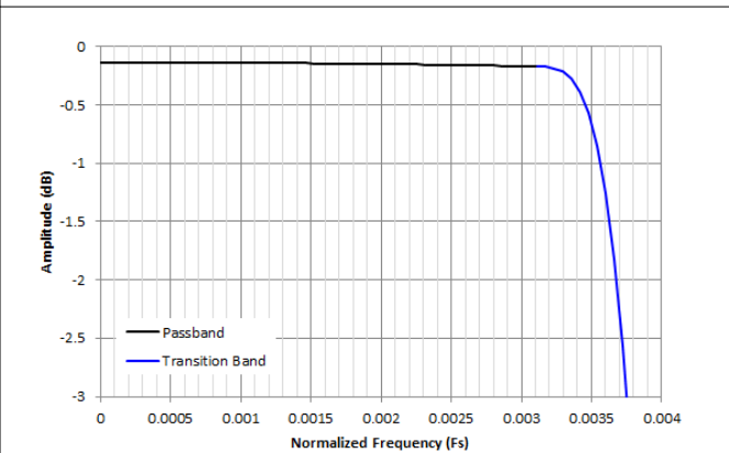
图 8-37. /128 抽取通带纹波响应
