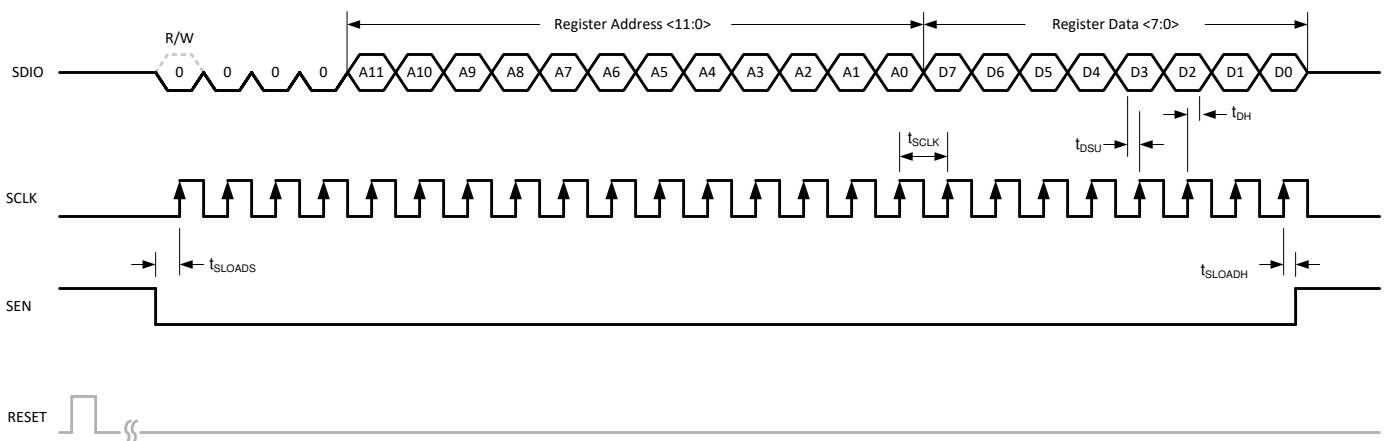
图 8-76. 串行寄存器写入时序图
