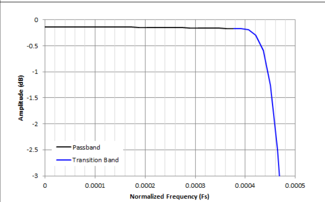
图 8-43. /1024 抽取通带纹波响应
