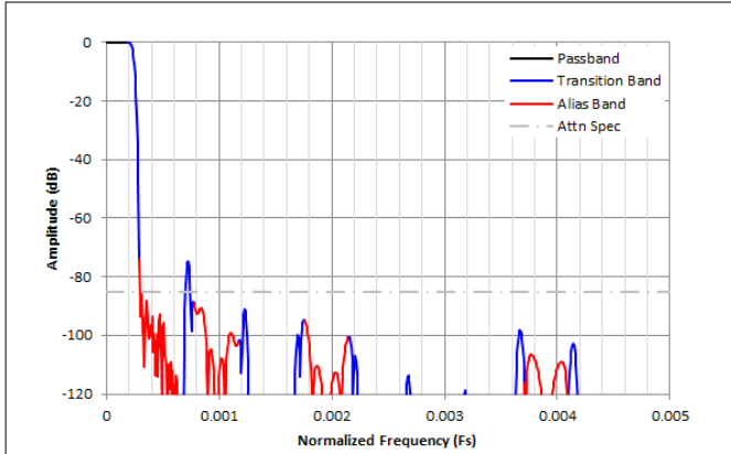
图 8-44. /2048 复数抽取滤波器响应
