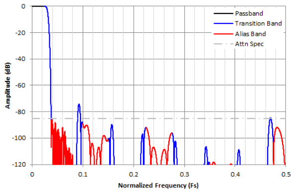
图 8-30. /16 复数抽取滤波器响应
