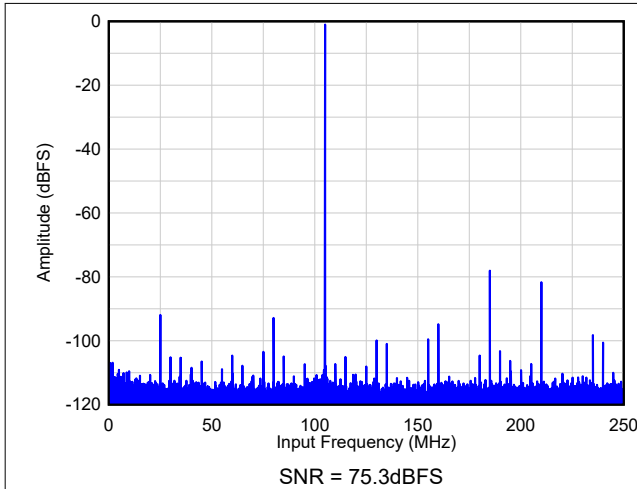
图 8-72. FFT - 无 AVG ( F_{IN} = 105\text{MHz} , A_{IN} = -1\text{dBFS} )
