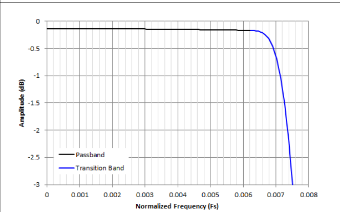
图 8-35. /64 复数抽取通带纹波响应
