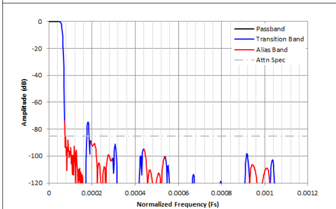
图 8-48. /8192 复数抽取滤波器响应
