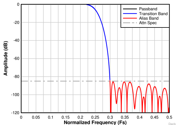
图 7-27. 2 倍复杂抽取率频率响应
