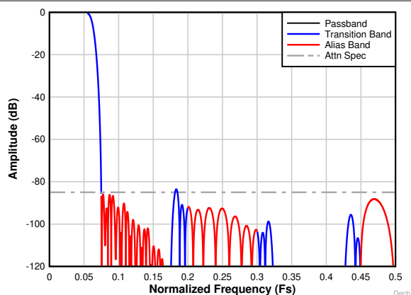
图 7-31. 8 倍复杂抽取率频率响应
