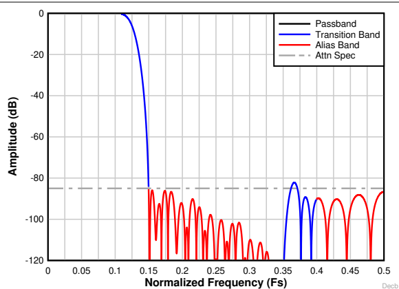
图 7-29. 4 倍复杂抽取率频率响应
