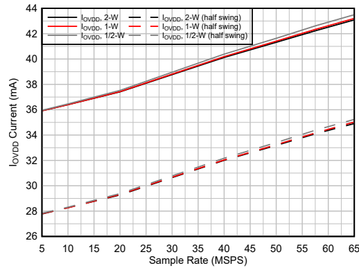
F_{IN} = 5\text{MHz} , 32 倍复数抽取率
