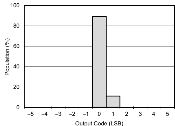
输出数据直方图 (256 项读数, 2.5SPS, 增益 = 1)
