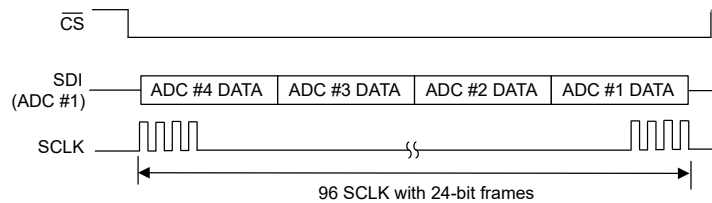
图 7-43. 24 位数据输入序列
