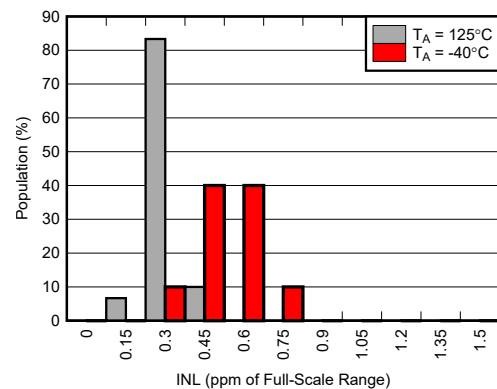
图 5-72. INL 分布图
