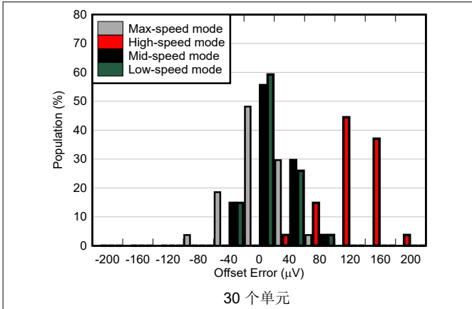
图 5-49. 偏移误差分布图
