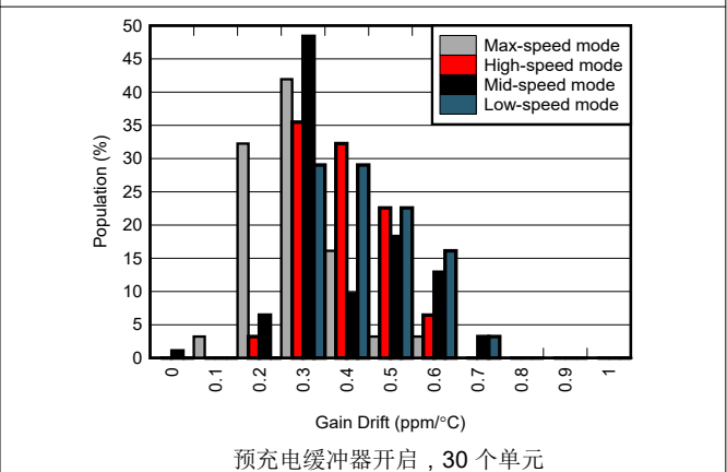
图 5-54. 增益漂移分布图
