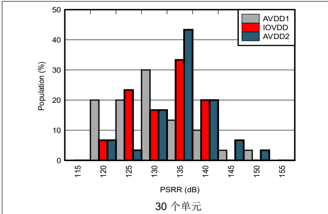
图 5-85. 直流 PSRR 分布图
