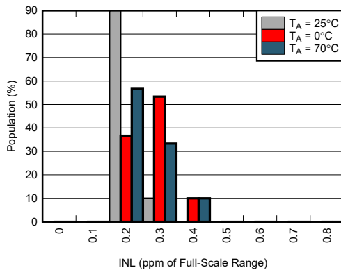
图 5-69. INL 分布图
