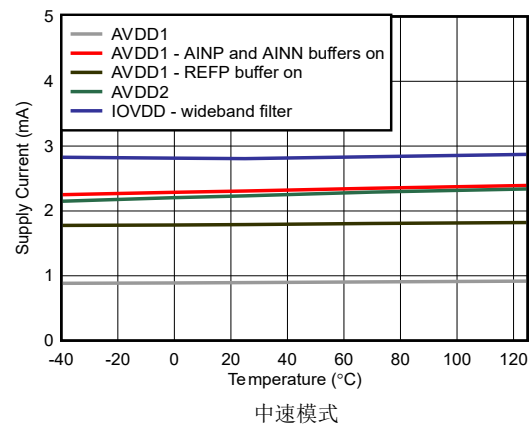
图 5-90. 电源电流与温度间的关系
