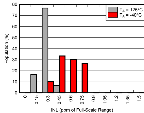
图 5-70. INL 分布图
