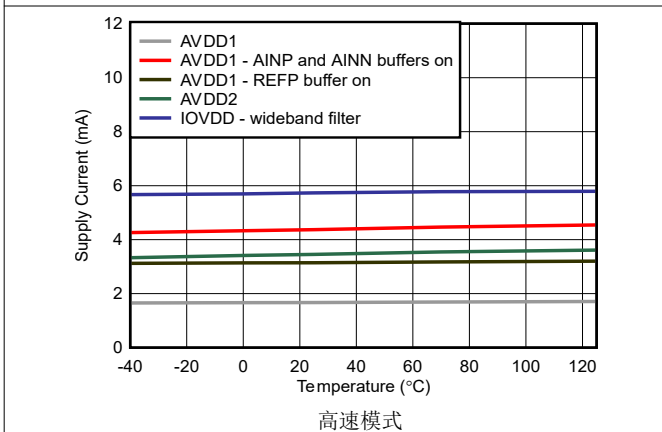
图 5-89. 电源电流与温度间的关系
