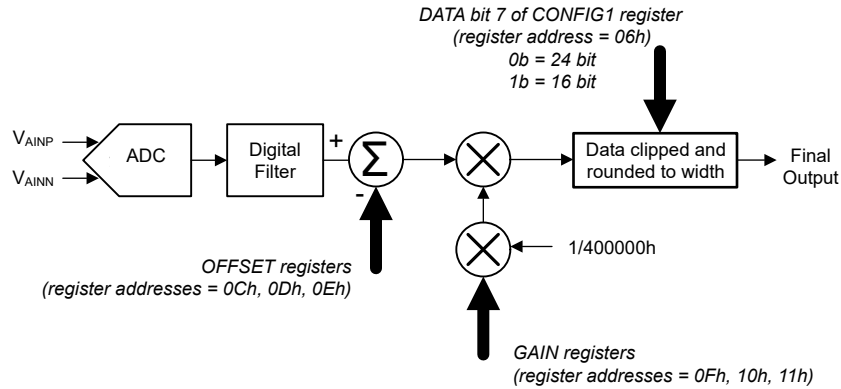
图 7-34. 校准方框图
