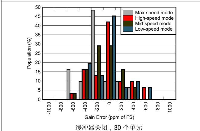
图 5-53. 增益误差分布图
