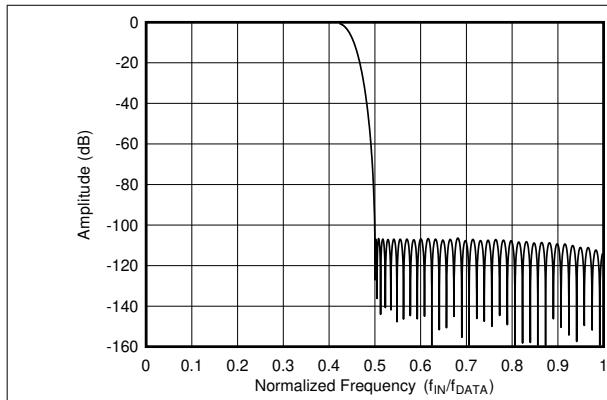
图 7-16. 宽带滤波器频率响应
