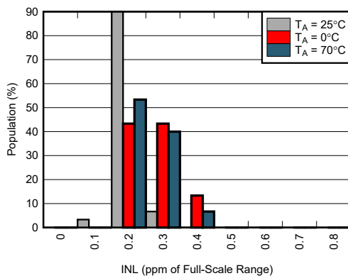
图 5-71. INL 分布图
