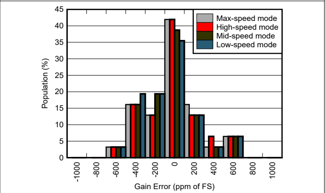
缓冲器开启，30 个单元
