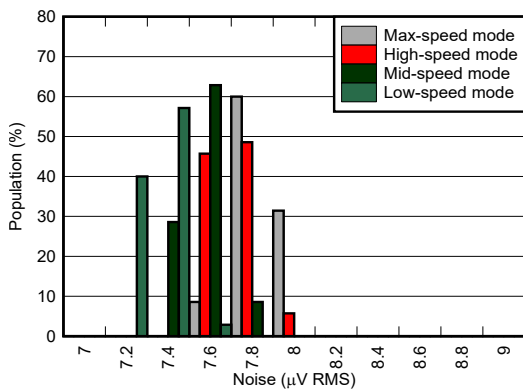
宽带滤波器, OSR = 64, 30 个单元
