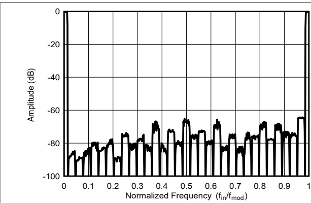
图 7-17. 宽带滤波器阻带衰减
