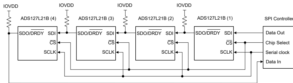
图 7-42. 菊花链连接
