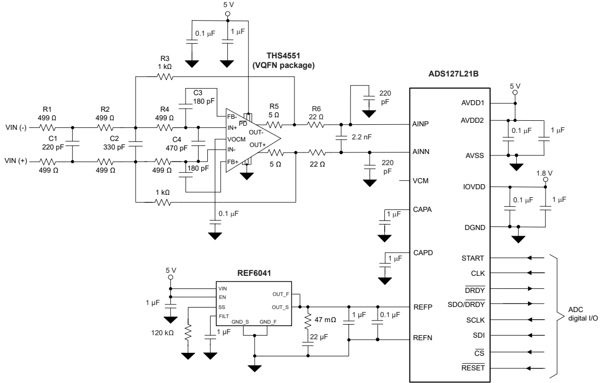
图 9-8. ADS127L21B 电路图
