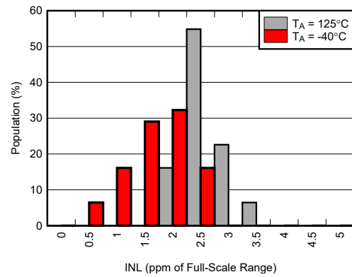
图 5-68. INL 分布图
