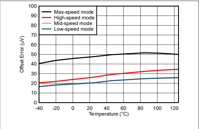
图 5-50. 偏移误差与温度间的关系
