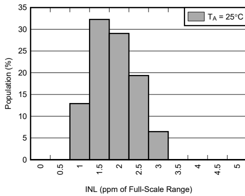
图 5-67. INL 分布图
