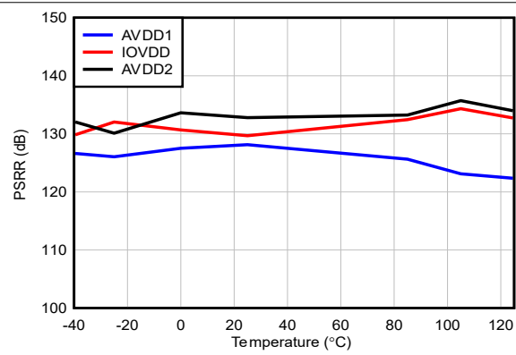
图 5-86. 直流 PSRR 与温度间的关系
