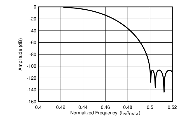
图 7-15. 宽带滤波器过渡带
