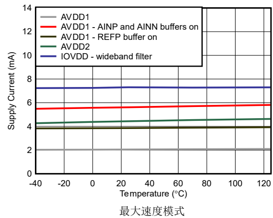
图 5-88. 电源电流与温度间的关系
