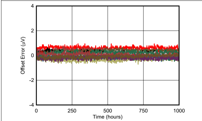
30 个单元，在 t = 0 时校准的偏移
