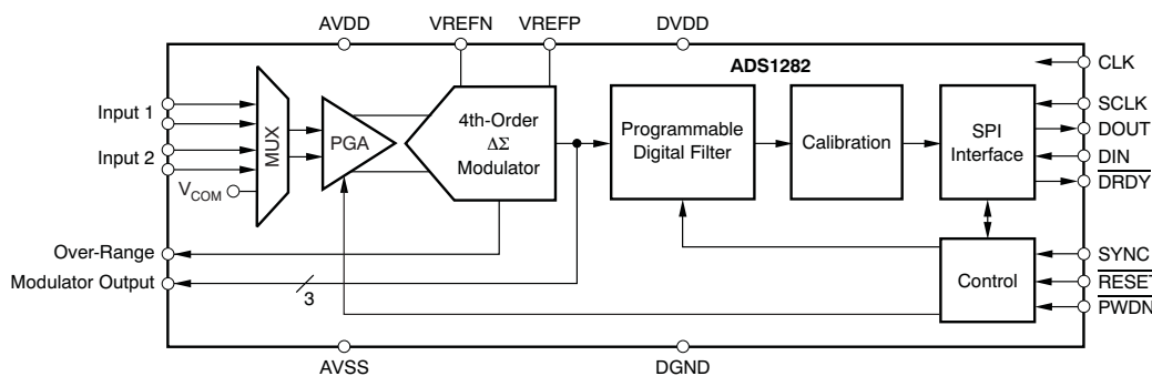
简化原理图
