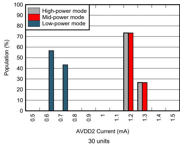
图 6-64. AVDD2 Current Distribution
