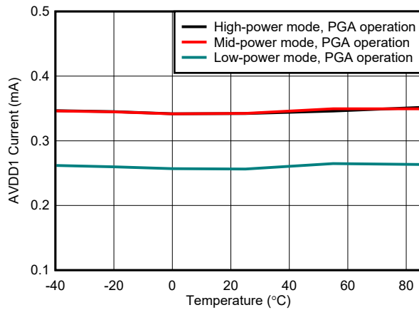
图 6-63. AVDD1 Current vs Temperature
