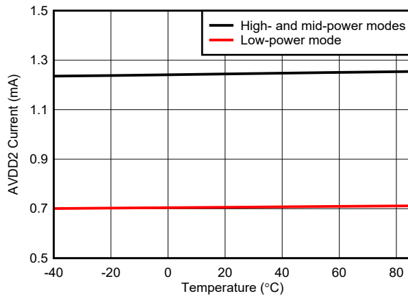
图 6-65. AVDD2 Current vs Temperature
