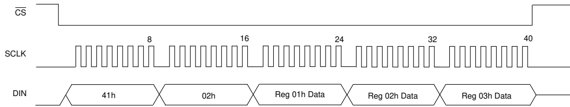
图 8-27. Write Register Data
