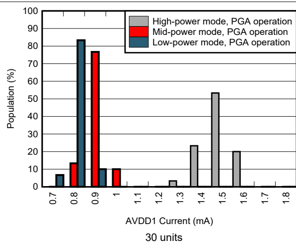
图 6-60. AVDD1 Current Distribution
