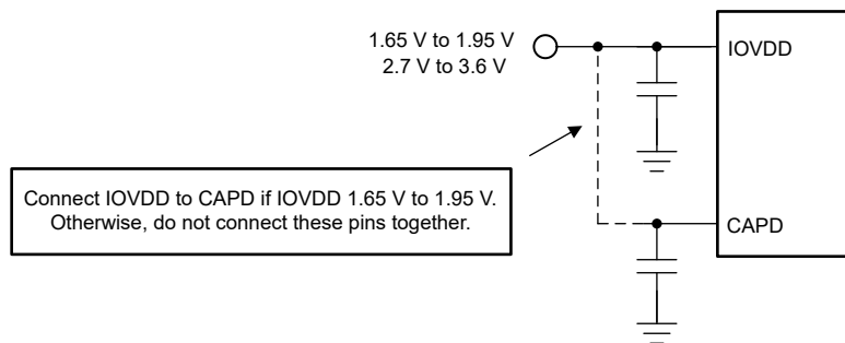
图 8-9. IOVDD Power-Supply Connection
