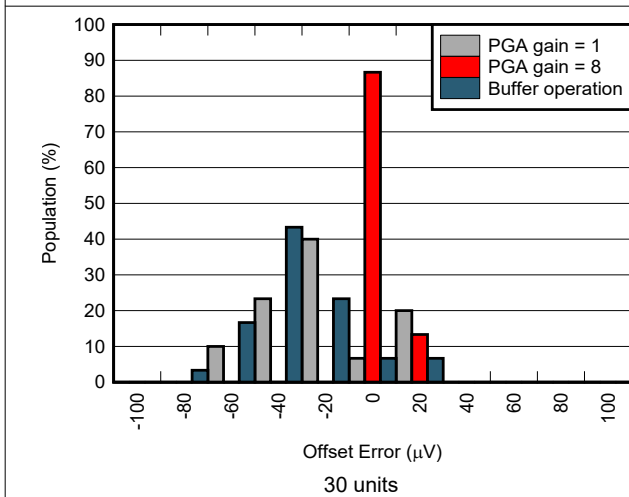
图 6-39. Offset Error Distribution
