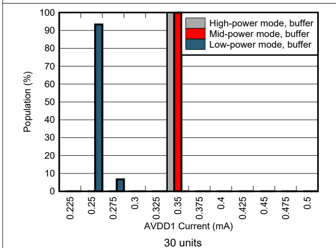
图 6-61. AVDD1 Current Distribution
