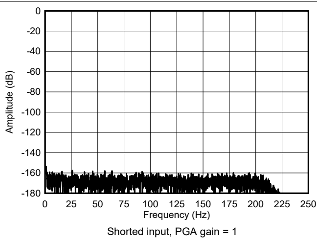
图 6-9. High-Power Mode FFT Spectrum
