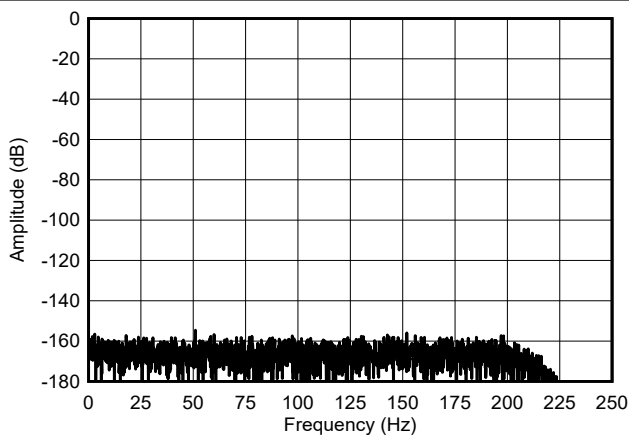
图 6-25. Mid-Power Mode FFT Spectrum
