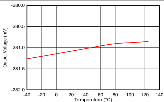
图 5-29. 测试 DACy 输出电压与温度间的关系
