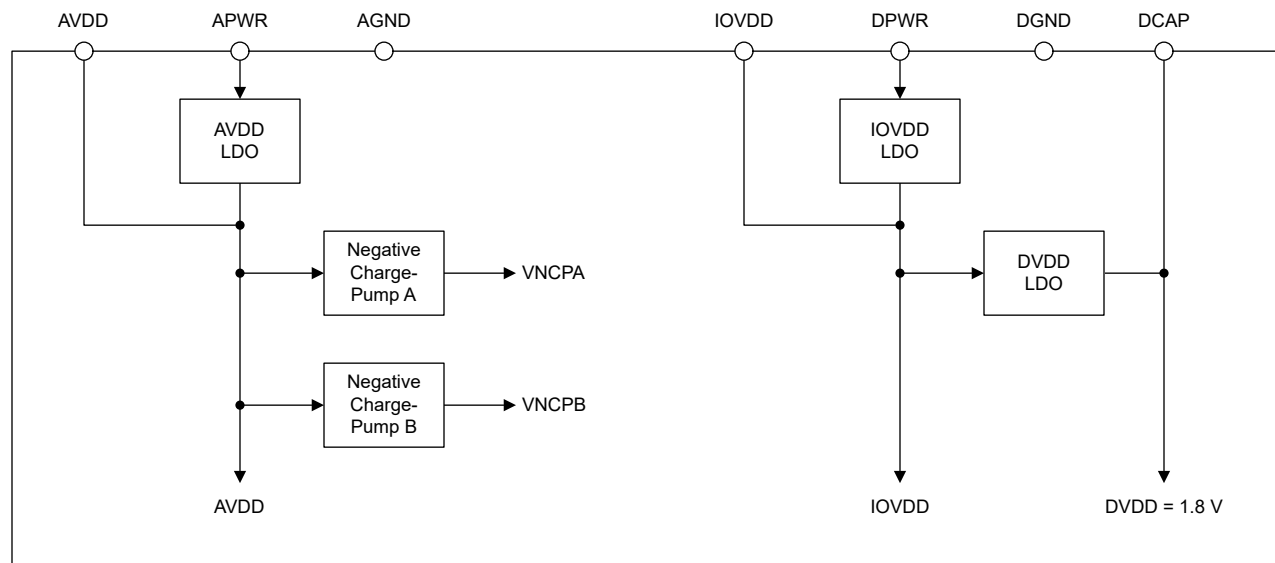
图 9-4. 电源架构
