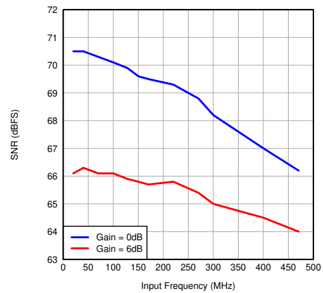
图 7-75. SNR vs Input Frequency
