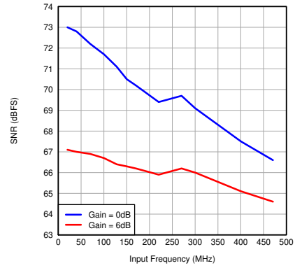
图 7-13. SNR vs Input Frequency (CMOS)
