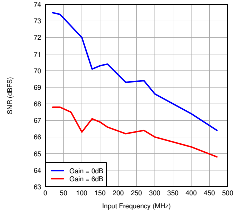
图 7-55. SNR vs Input Frequency (CMOS)
