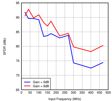
图 7-53. SFDR vs Input Frequency
