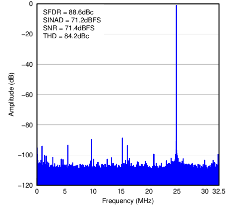
图 7-49. FFT for 170-MHz Input Signal
