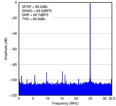
图 7-105. FFT for 170-MHz Input Signal
