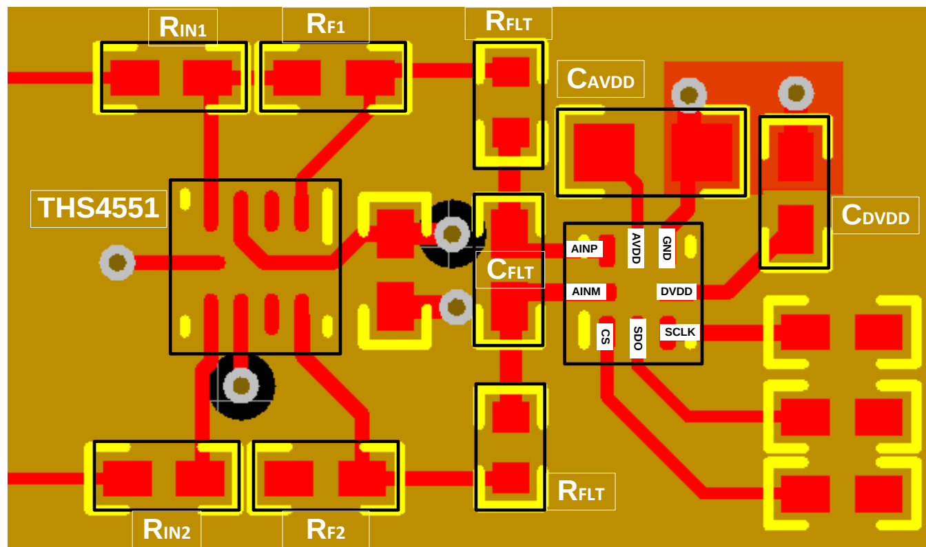
图 48. Example Layout
