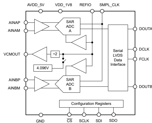
器件方框图
