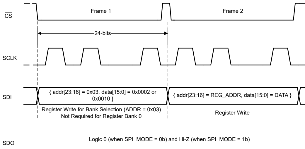
图 6-9. 寄存器写入
