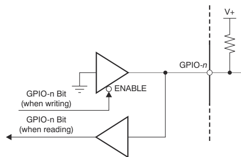
图 7-17. GPIO Pins
