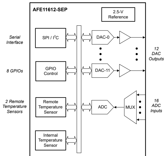
简化原理图
