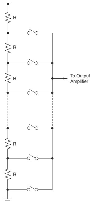
图 7-10. Resistor String
