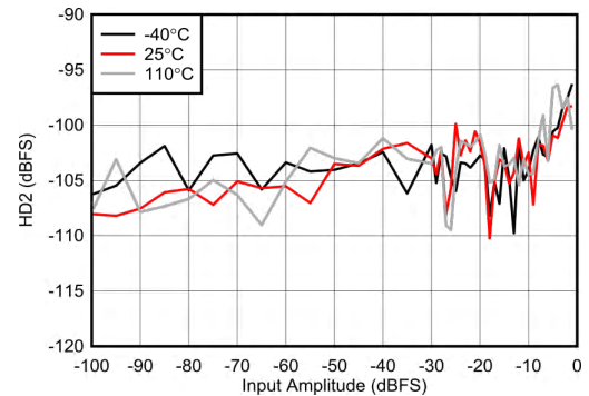
图 6-221. RX HD2 vs Input Amplitude at 6.851GHz
