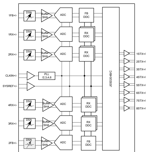
功能方框图
