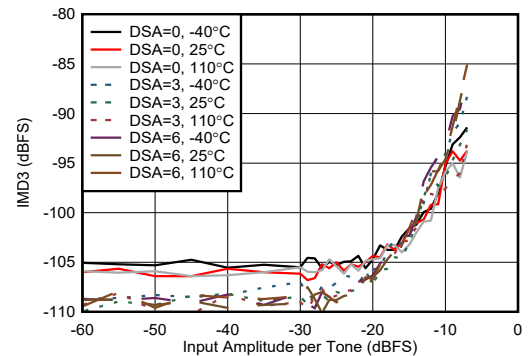
图 6-217. RX IMD3 vs Input Amplitude at 6.851GHz
