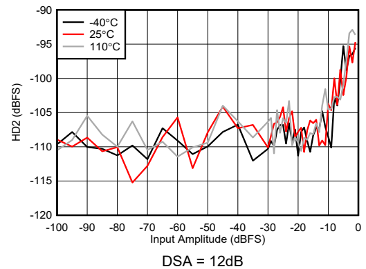
图 6-223. RX HD2 vs Input Amplitude at 6.851GHz
