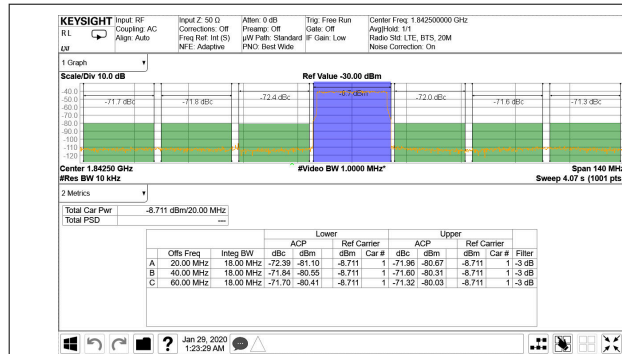
图 4-68. TX 20-MHz LTE Output Spectrum at 1.8425GHz
