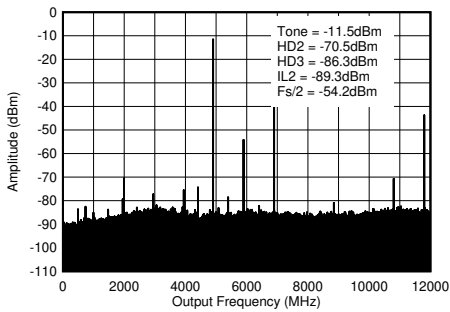
f_{\text{DAC}} = 11796.48\text{MSPS} ，交错模式，4.9GHz 匹配，包括 PCB 和电缆损耗。ILn = f_s/n \pm f_{\text{OUT}}
