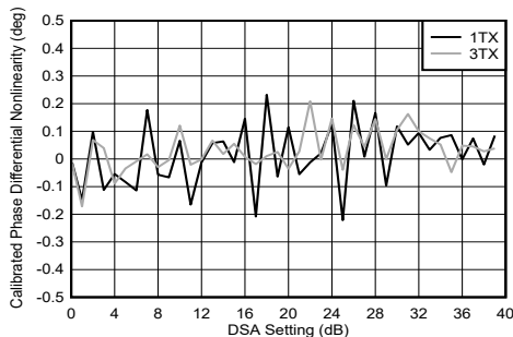
图 5-196. 8.11GHz 条件下 TX DSA 已校准相位微分非线性
