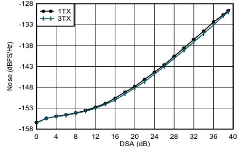
图 5-168. 2.6GHz 条件下 TX 输出噪声与通道和衰减间的关系
