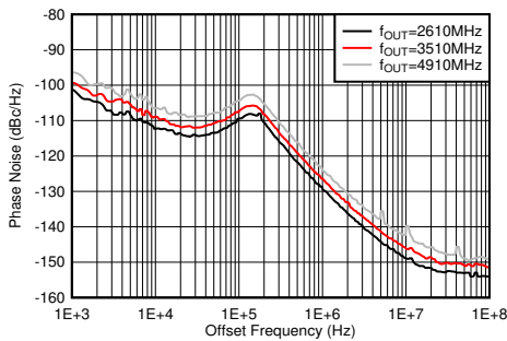
PLL 启用, f_{VCO} = 8847.36\text{MHz} , f_{REF} = 491.52\text{MSPS} , 在 TX 输出端测量 图 5-502. 110°C 条件下 9GHz VCO 相位噪声与偏移频率和 f_{OUT} 间的关系
