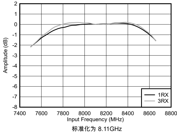
图 5-422. RX 振幅与频率和通道间的关系
