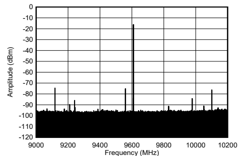
图 5-268. 9.61GHz 和 -6dBFS (1.2 GHz 带宽) 条件下 TX 单音频谱
