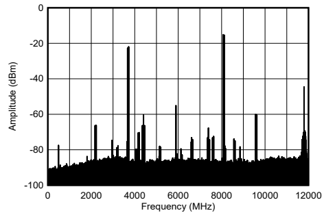
图 5-209. 8.1GHz 条件下 TX 双音输出频谱
