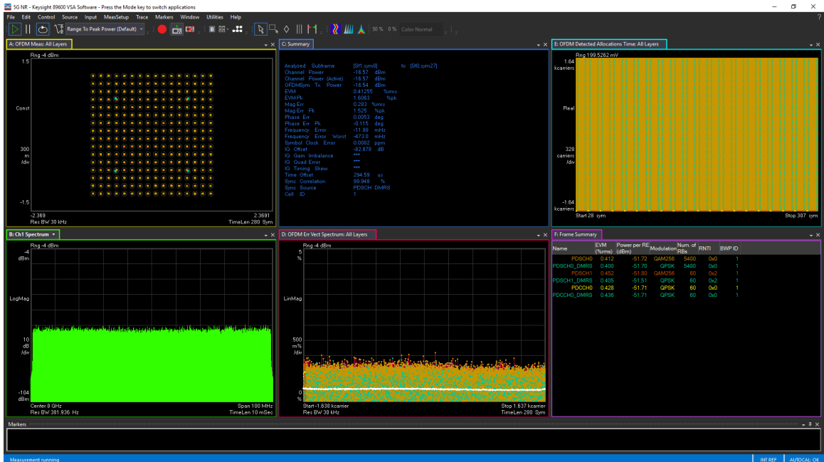
图 5-230. 8.11GHz 条件下 TX 100MHz NR EVM
