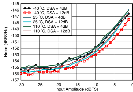
图 5-406. 4.9GHz 条件下 RX 噪声频谱密度与输入振幅和温度间的关系
