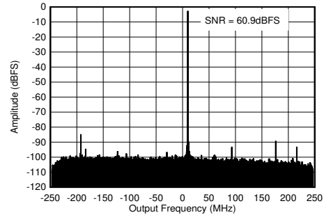
图 5-327. 1.75GHz 条件下的 RX 输出 FFT
