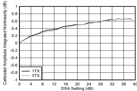
图 5-192. 8.11GHz 条件下 TX DSA 已校准振幅积分非线性
