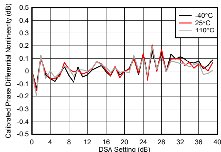
图 5-198. 8.11GHz 条件下 TX DSA 已校准相位微分非线性
