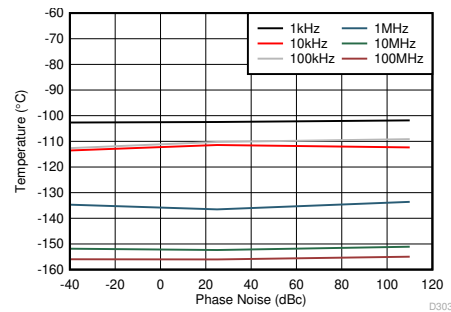
PLL 启用, f_{VCO} = 8847.36\text{MHz} , f_{REF} = 491.52\text{MSPS} , 最小 LPF 带宽, 在 TX 输出端测量 图 5-503. f_{OUT} = 2.6\text{GHz} 时 9GHz VCO 相位噪声与温度和偏移频率间的关系
