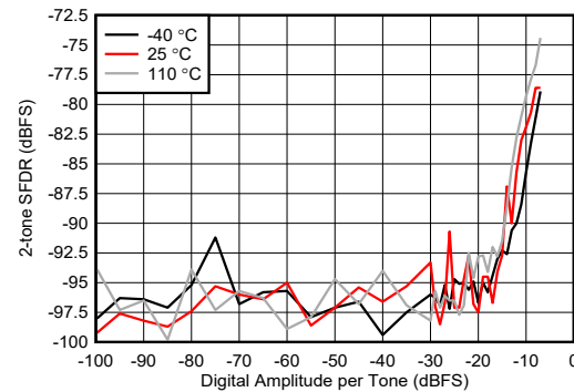
图 5-439. 8.11GHz 条件下 RX 双音 SFDR 与数字振幅间的关系
