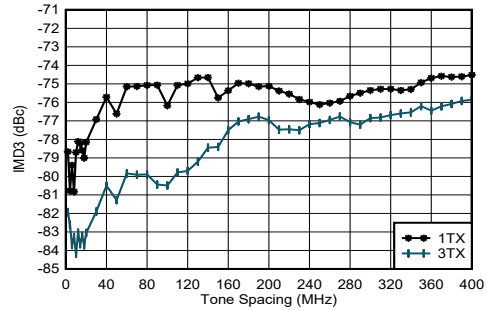
f_{\text{DAC}} = 11796.48\text{MSPS} ，交错模式， f_{\text{CENTER}} = 0.85\text{GHz} ，在 0.8GHz 条件下匹配，单音幅度为 -13\text{dBFS}
