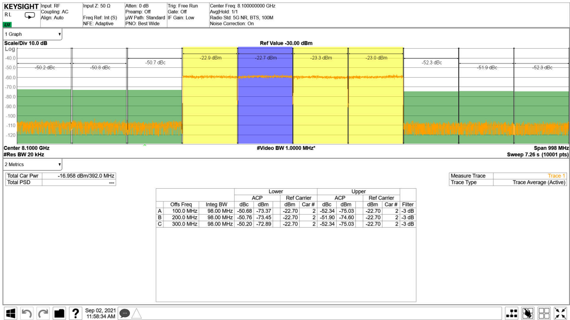
图 5-231. 8.1GHz 条件下 TX 4x100MHz NR 输出频谱
