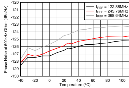
图 5-493. f_{OUT} = 2.6\text{GHz} 时 10GHz VCO 相位噪声 (600kHz 条件下) 与温度和 f_{REF} 间的关系
