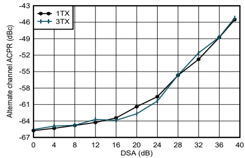
图 5-227. 8.11GHz 条件下 TX NR100MHz alt-ACPR 与 DSA 设置间的关系
