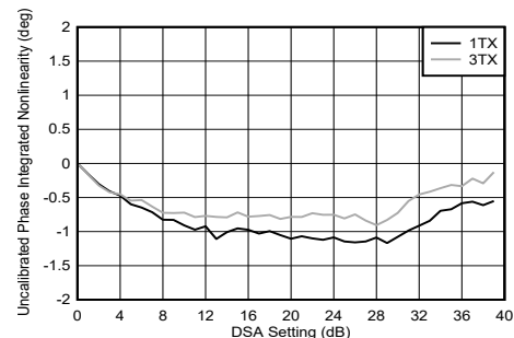
图 5-199. 8.11GHz 条件下 TX DSA 未校准相位积分非线性
