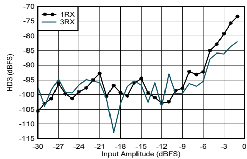
图 5-310. 0.8GHz 条件下 RX HD3 与输入电平和通道间的关系
