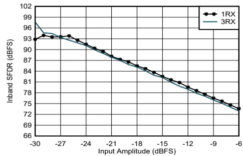
图 5-418. 4.9GHz 条件下 RX 带内 SFDR ( \pm 400\text{MHz} ) 与输入幅度和通道间的关系
