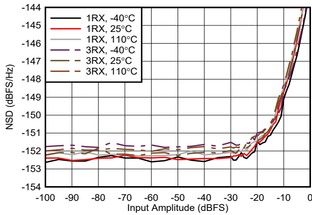
图 5-458. 9.6GHz 条件下 RX NSD 与数字振幅间的关系
