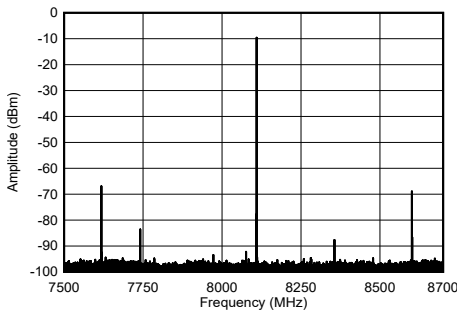
图 5-204. 8.11GHz 条件下 TX 单音输出频谱
