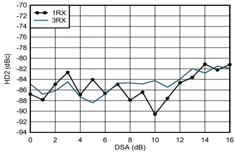
图 5-411. 4.9GHz 条件下 RX HD2 与 DSA 设置和通道间的关系
