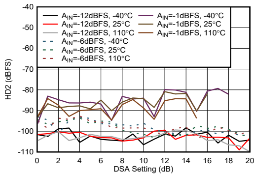
图 5-436. 8.11GHz 条件下 RX HD2 与 DSA 设置间的关系
