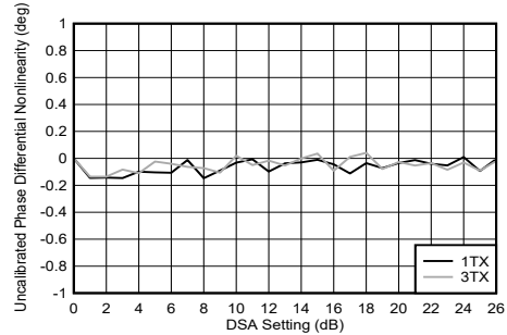
图 5-244. TX DSA 未校准相位微分非线性
