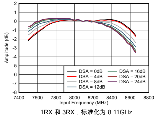
图 5-423. RX 振幅与频率和 DSA 设置间的关系
