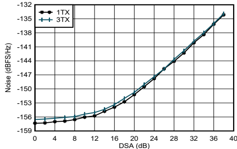
f_{\text{DAC}} = 8847.36\text{MSPS} ，直接模式，在 2.6GHz 条件下匹配， P_{\text{OUT}} = -13\text{dBFS}
