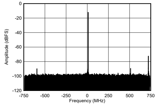
图 5-465. 9.61GHz 条件下 RX 单音输出 FFT
