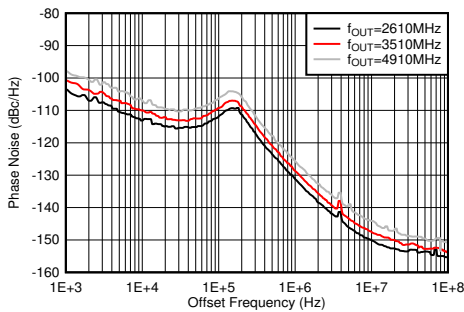
PLL 启用, f_{VCO} = 8847.36\text{MHz} , f_{REF} = 491.52\text{MSPS} , 在 TX 输出端测量 图 5-500. 25°C 条件下 9GHz VCO 相位噪声与偏移频率和 f_{OUT} 间的关系
