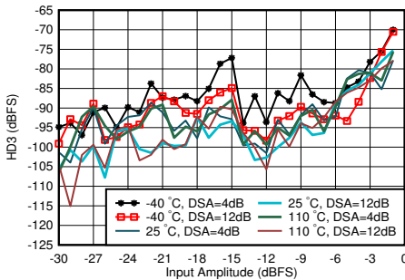
图 5-309. 0.8GHz 条件下 RX HD3 与 DSA 设置和温度间的关系
