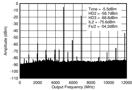
f_{\text{DAC}} = 11796.48\text{MSPS} ，交错模式，4.9GHz 匹配，包括 PCB 和电缆损耗。ILn = f_s/n \pm f_{\text{OUT}}
