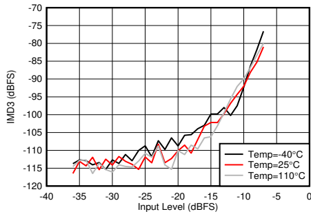
图 5-354. 2.6GHz 条件下 RX IMD3 与输入电平和温度间的关系
