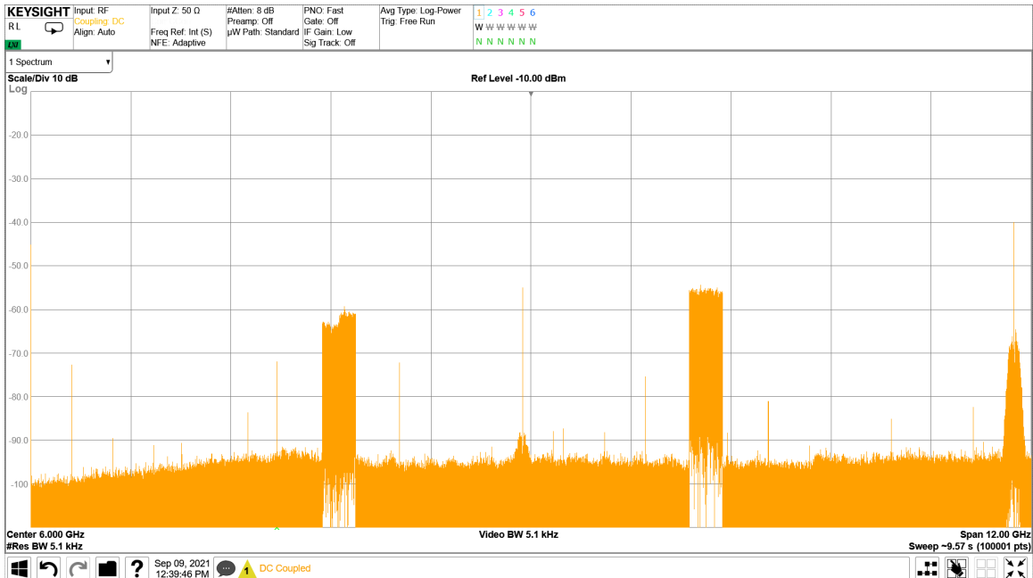
图 5-232. 8.1GHz 条件下 TX 4x100MHz NR 输出频谱
