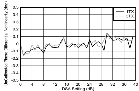
图 5-195. 8.11GHz 条件下 TX DSA 未校准相位微分非线性
