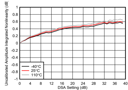
图 5-193. 8.11GHz 条件下 TX DSA 未校准振幅积分非线性
