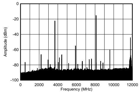
图 5-205. 8.11GHz 条件下 TX 单音输出频谱
