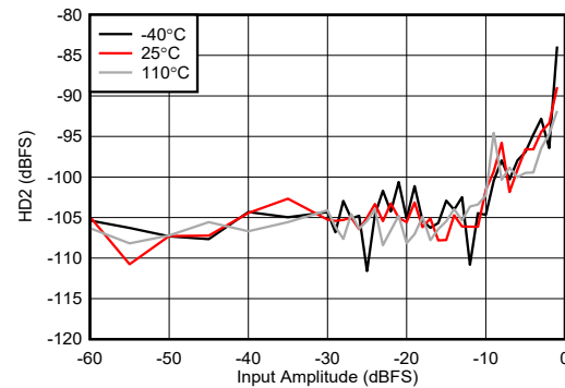
图 5-435. 8.11GHz 条件下 RX HD2 与数字振幅间的关系
