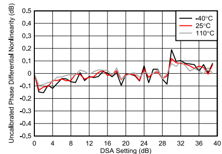
图 5-197. 8.11GHz 条件下 TX DSA 未校准相位微分非线性
