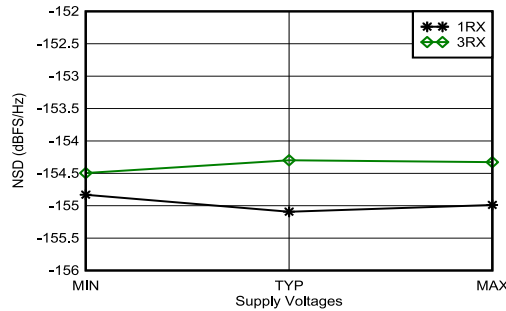
使用 3.6GHz 匹配时，单音幅度为 -20dBFS，偏移频率为 12.5MHz，所有电源均处于 MIN、TYP 或 MAX 推荐工作电压 图 5-392. 3.6GHz 条件下 RX 噪声频谱密度与电源电压和通道间的关系
