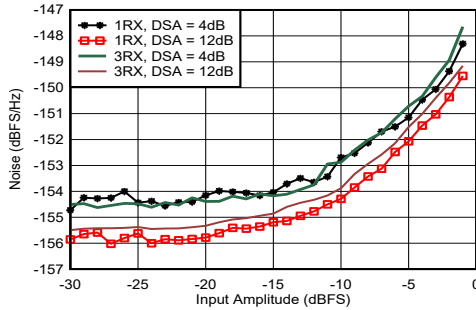
图 5-299. 0.8GHz 条件下 RX 噪声频谱密度与输入幅度和通道间的关系
