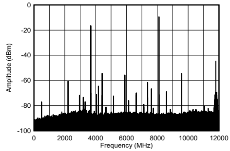
图 5-203. 8.11GHz 条件下 TX 单音输出频谱
