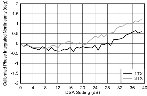
图 5-200. 8.11GHz 条件下 TX DSA 已校准相位积分非线性
