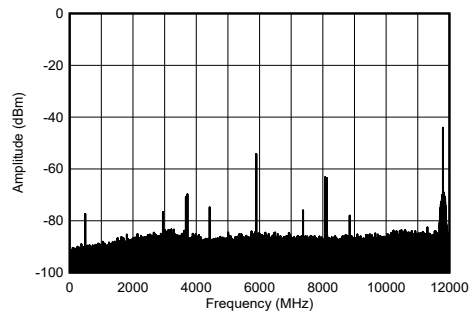
图 5-213. 8.1GHz 条件下 TX 双音输出频谱
