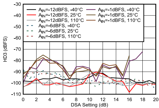
图 5-438. 8.11GHz 条件下 RX HD3 与 DSA 设置间的关系
