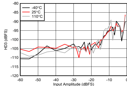
图 5-437. 8.11GHz 条件下 RX HD3 与数字振幅间的关系
