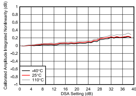
图 5-194. 8.11GHz 条件下 TX DSA 已校准振幅积分非线性
