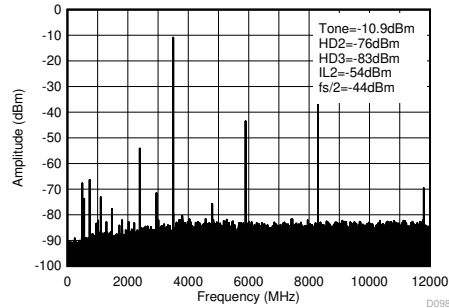
图 5-148. 3.5GHz (0 - f_{\text{DAC}} ) 条件下的 TX 单音 (-12dBFS) 输出频谱
