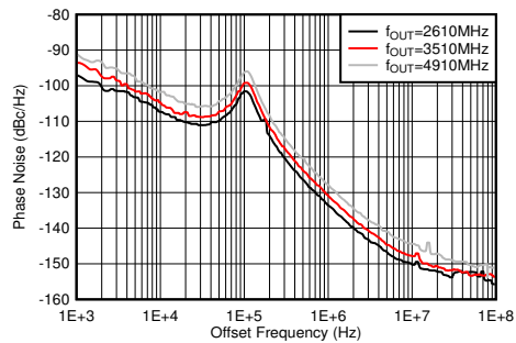
PLL 启用, f_{VCO} = 8847.36\text{MHz} , f_{REF} = 491.52\text{MSPS} , 在 TX 输出端测量 图 5-501. -40°C 条件下 9GHz VCO 相位噪声与偏移频率和 f_{OUT} 间的关系
