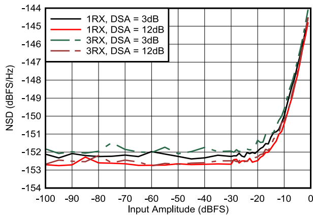
图 5-432. 8.11GHz 条件下 RX NSD 与数字振幅间的关系
