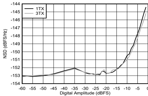
图 5-259. 9.61GHz 条件下 TX NSD 与数字振幅间的关系
