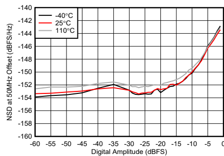
50MHz 偏移
