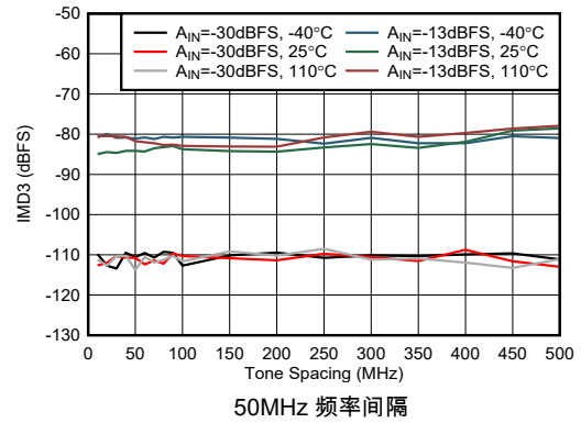
图 5-457. 9.6 GHz 条件下 RX IMD3 与频率间隔间的关系
