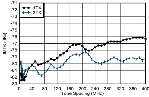
f_{\text{DAC}} = 8847.36\text{MSPS} ，直接模式， f_{\text{CENTER}} = 0.85\text{GHz} ，在 0.8GHz 条件下匹配，单音幅度为 -13\text{dBFS}
