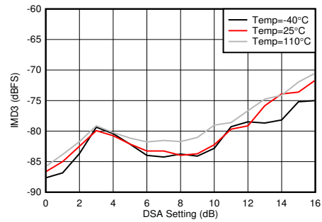
图 5-353. 2.6GHz 条件下 RX IMD3 与 DSA 设置和温度间的关系
