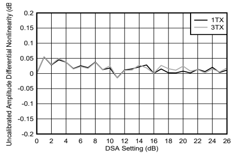
图 5-236. TX DSA 未校准振幅微分非线性
