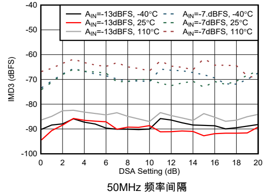
图 5-455. 9.6 GHz 条件下 RX IMD3 与 DSA 设置间的关系
