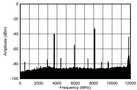
图 5-211. 8.1GHz 条件下 TX 双音输出频谱
