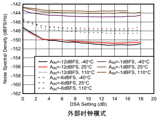
图 5-434. 8.11GHz 条件下 RX NSD 与 DSA 设置间的关系
