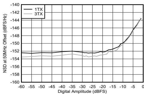
50MHz 偏移
