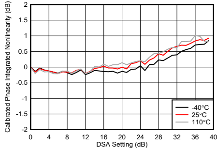
图 5-202. 8.11GHz 条件下 TX DSA 已校准相位积分非线性
