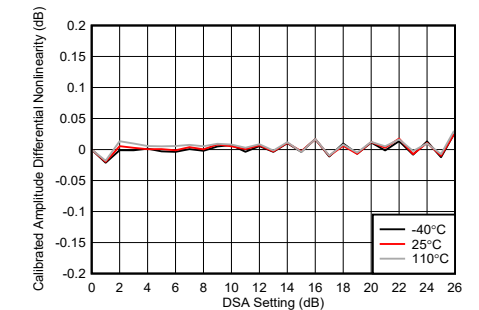
图 5-239. TX DSA 已校准振幅微分非线性
