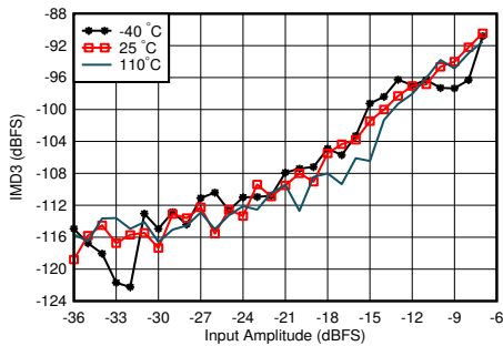
图 5-332. 1.75GHz 条件下 RX IMD3 与输入电平和温度间的关系
