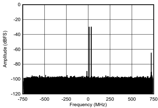
9.61GHz 和 9.635GHz，单频幅度为 -30dBFS
