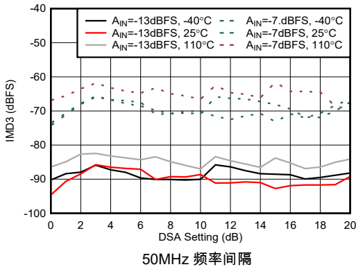
图 5-456. 9.6 GHz 条件下 RX IMD3 与 DSA 设置间的关系
