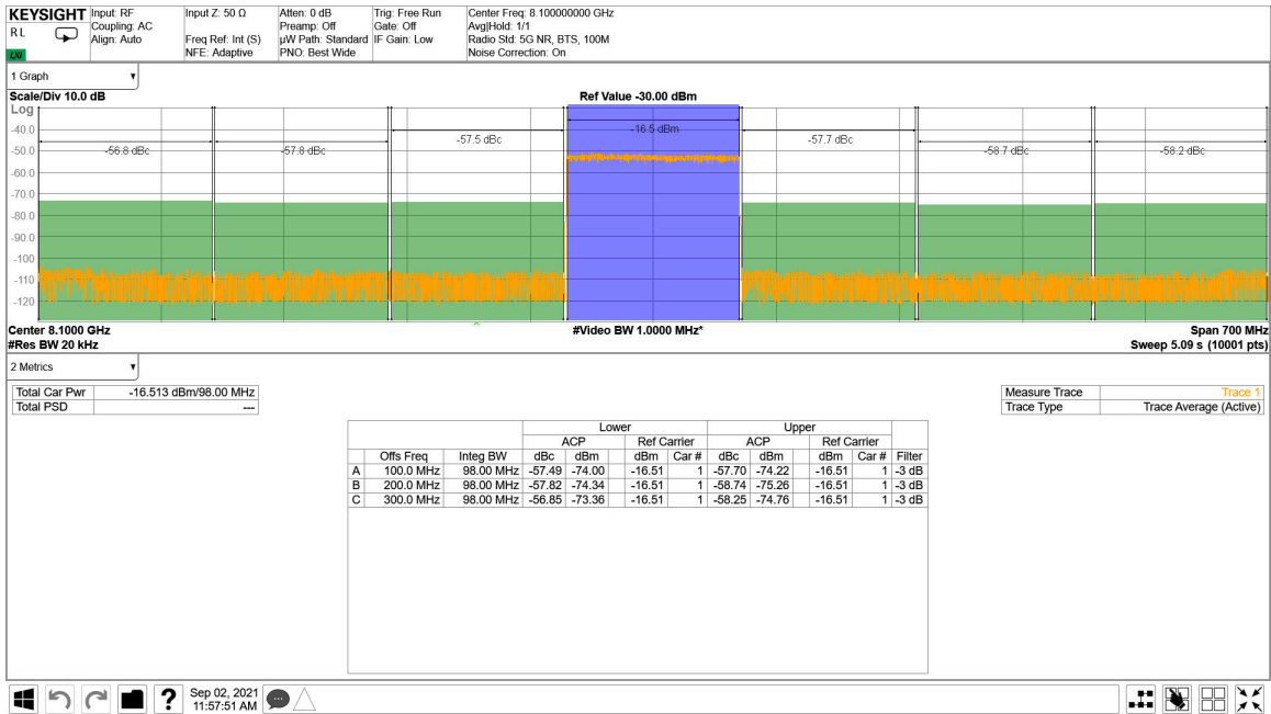
图 5-229. 8.11GHz 条件下 TX 100MHz NR 输出频谱
