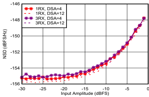
图 5-352. 2.6GHz 条件下 RX 噪声频谱密度与输入振幅和通道间的关系
