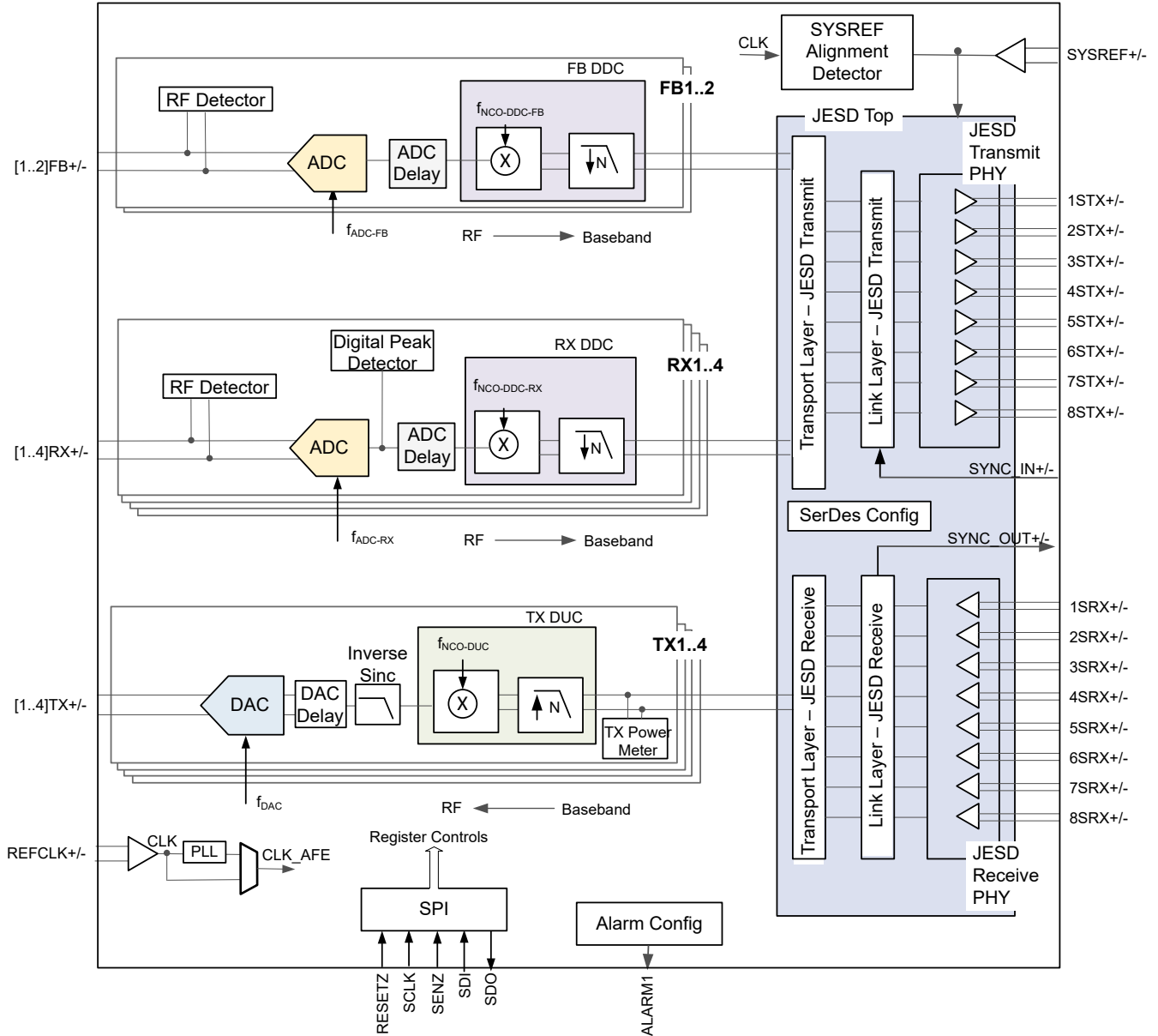
功能方框图
