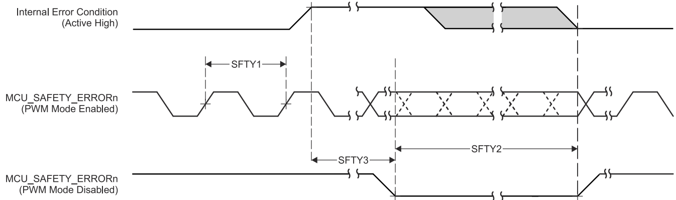
图 6-11. MCU_SAFETY_ERRORn 时序要求和开关特性
