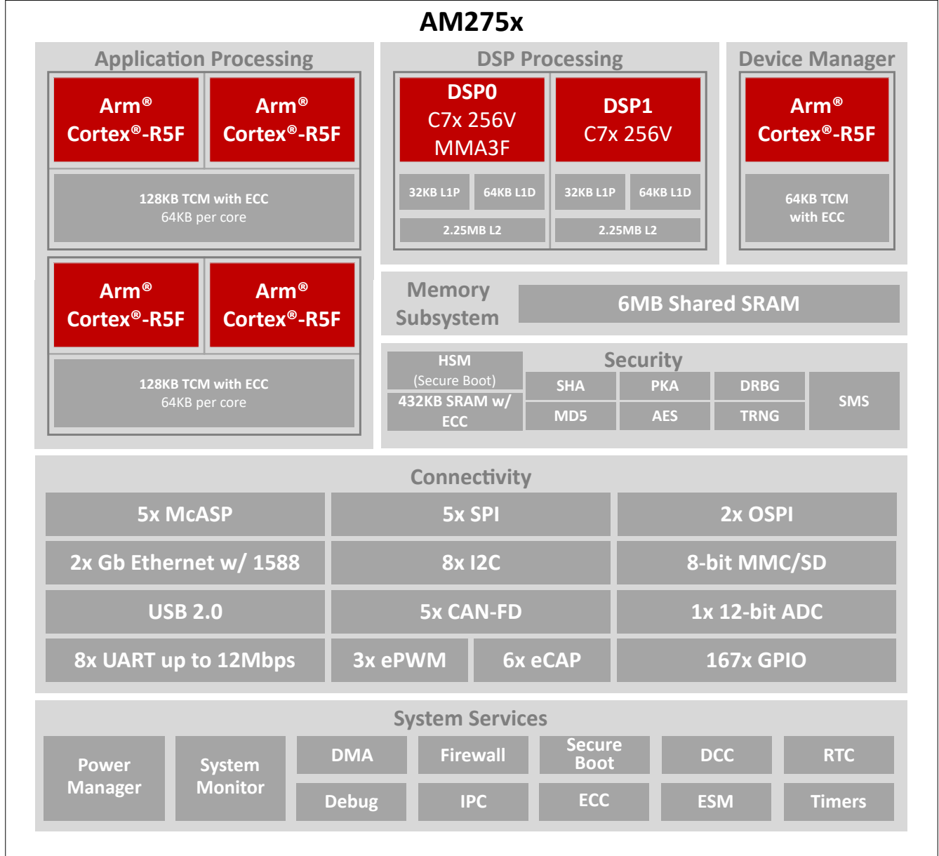
图 7-1. 功能方框图
