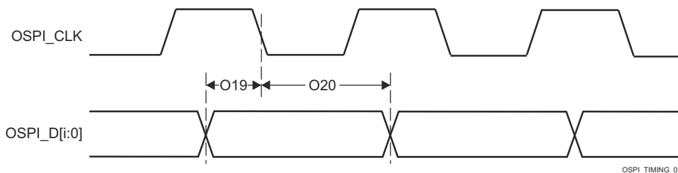
图 6-63. OSPI0 时序要求 - Tap SDR, 无环回
