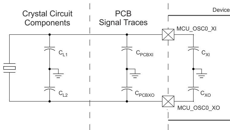
图 6-15. 负载电容
