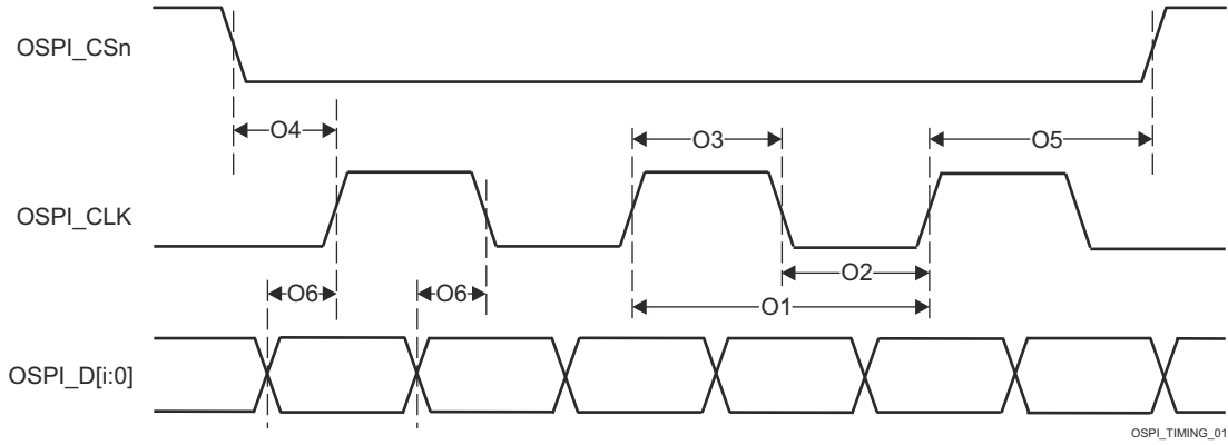
图 6-66. OSPI0 开关特性 - Tap DDR , 无环回
