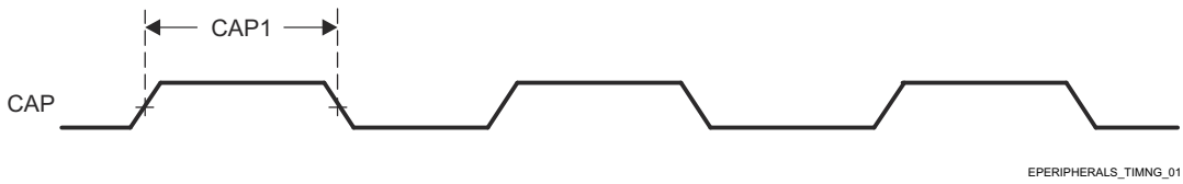
图 6-29. ECAP 时序要求
