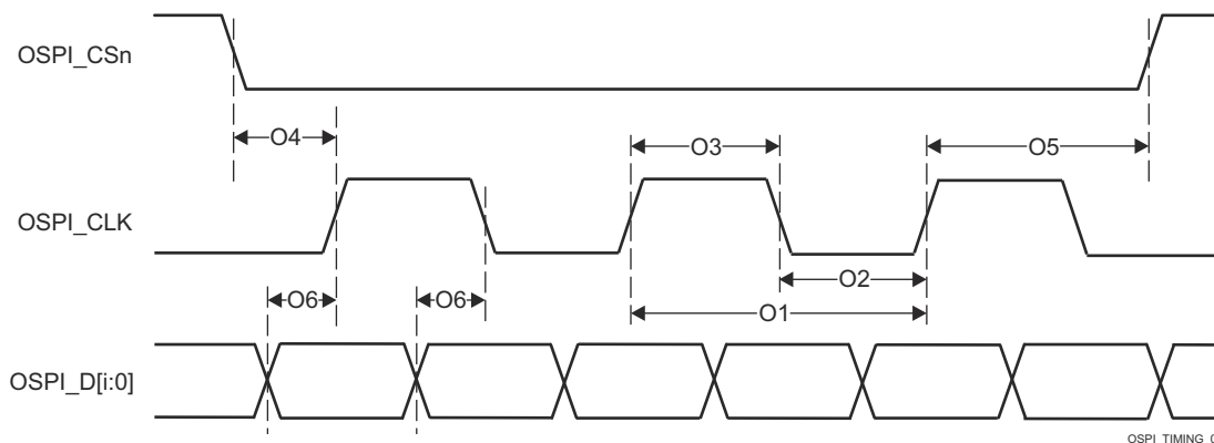
图 6-62. OSPI0 开关特性 - PHY DDR
