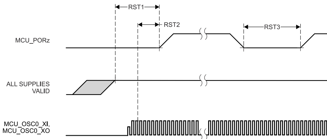
图 6-8. MCU_PORz 时序要求
