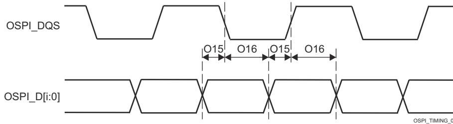
图 6-61. OSPI0 时序要求 - 具有外部电路板环回或 DQS 的 PHY DDR
