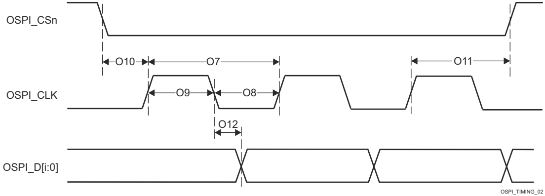
图 6-64. OSPI0 开关特性 - Tap SDR, 无环回
