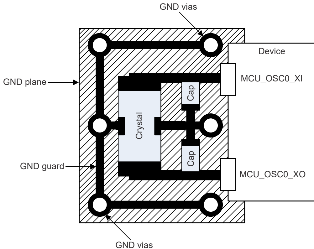
图 8-4. MCU_OSC0/OSC1/WKUP_LFOSC0 PCB 要求
