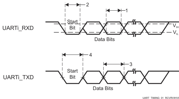
图 6-68. UART 时序要求和开关特性
