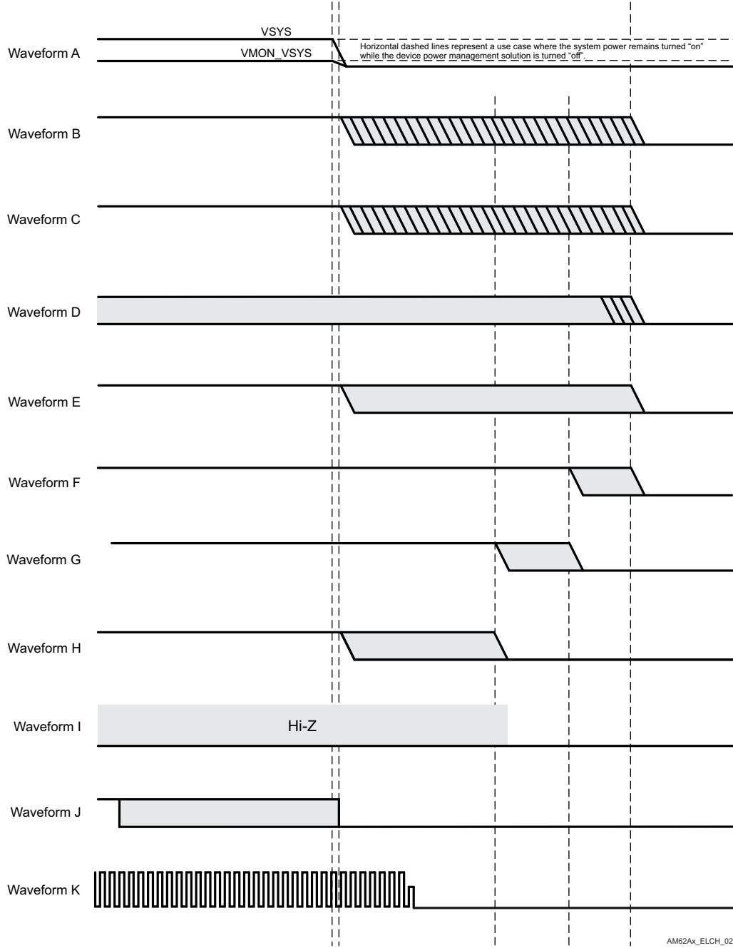
图 6-7. 下电时序
