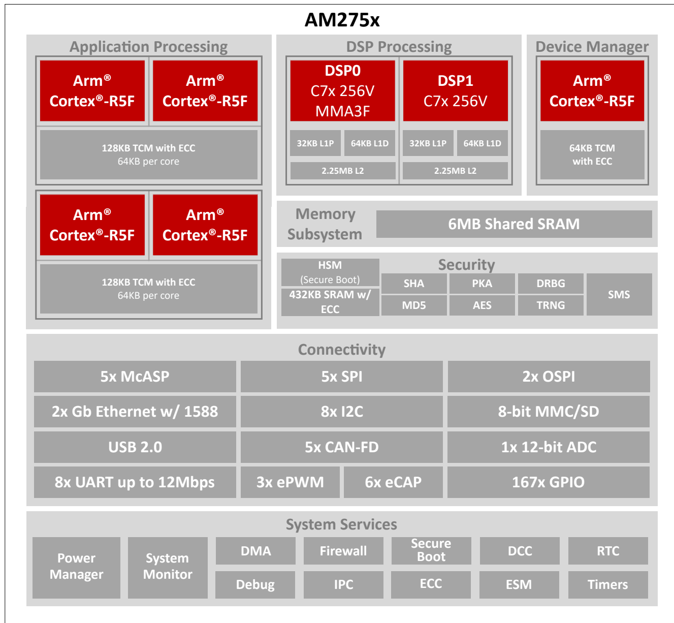
图 3-1. 功能方框图
