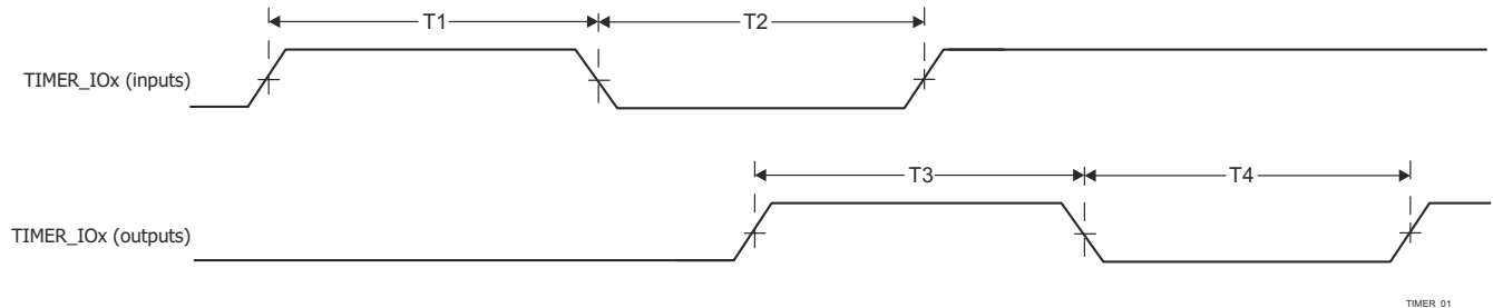
图 6-67. 计时器时序要求和开关特性
