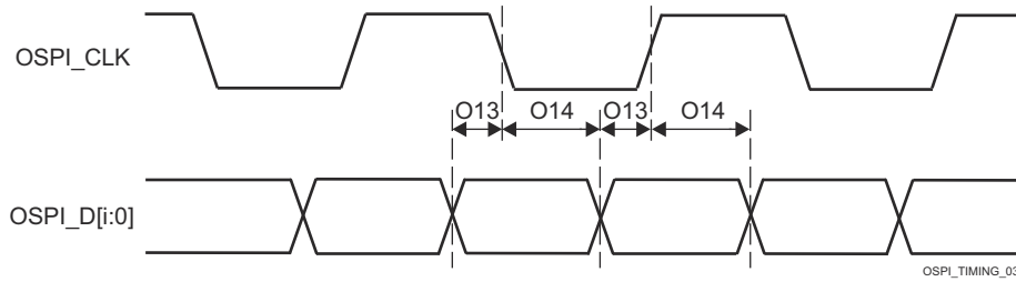
图 6-65. OSPI0 时序要求 - Tap DDR, 无环回
