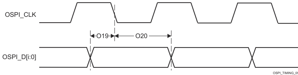
图 6-58. OSPI0 时序要求 - 具有内部 PHY 环回的 PHY SDR
