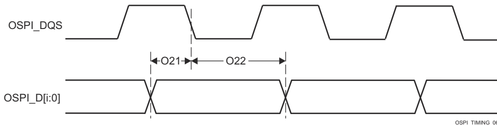
图 6-59. OSPI0 时序要求 - 具有外部电路板环回的 PHY SDR
