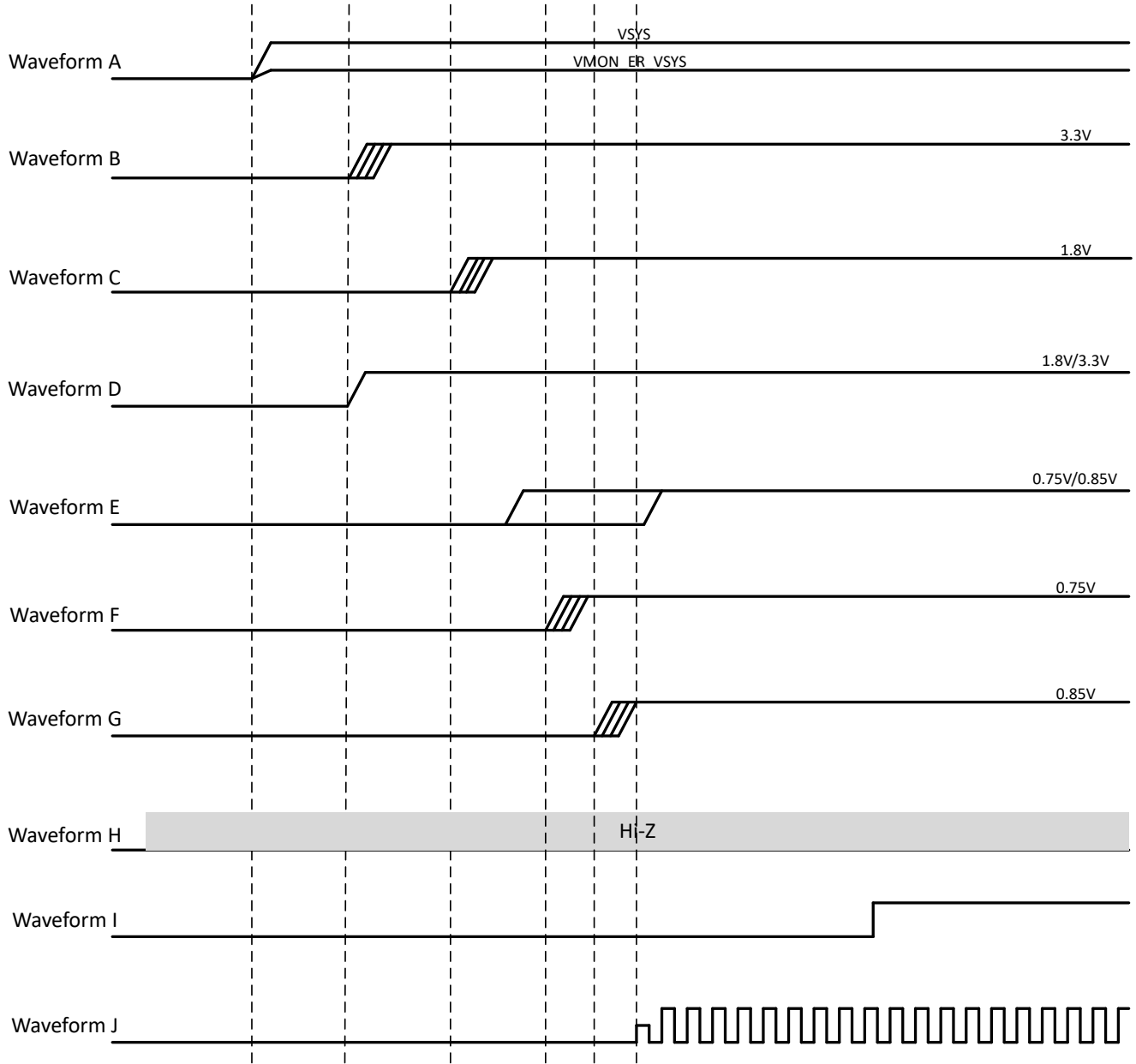
图 6-4. 上电时序
