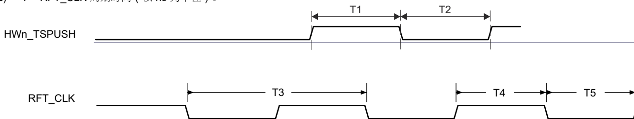
图 6-30. CPTS 时序要求
