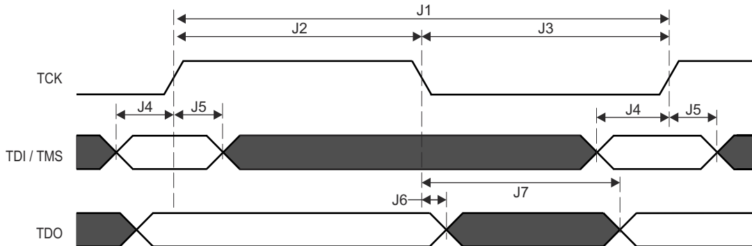
图 6-36. JTAG 时序要求和开关特性
