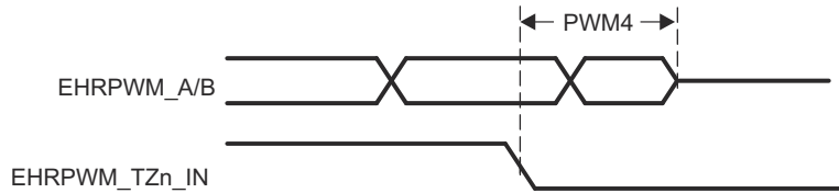
图 6-40. EHRPWM_TZn_IN 至 EHRPWM_A/B 高阻态开关特性
