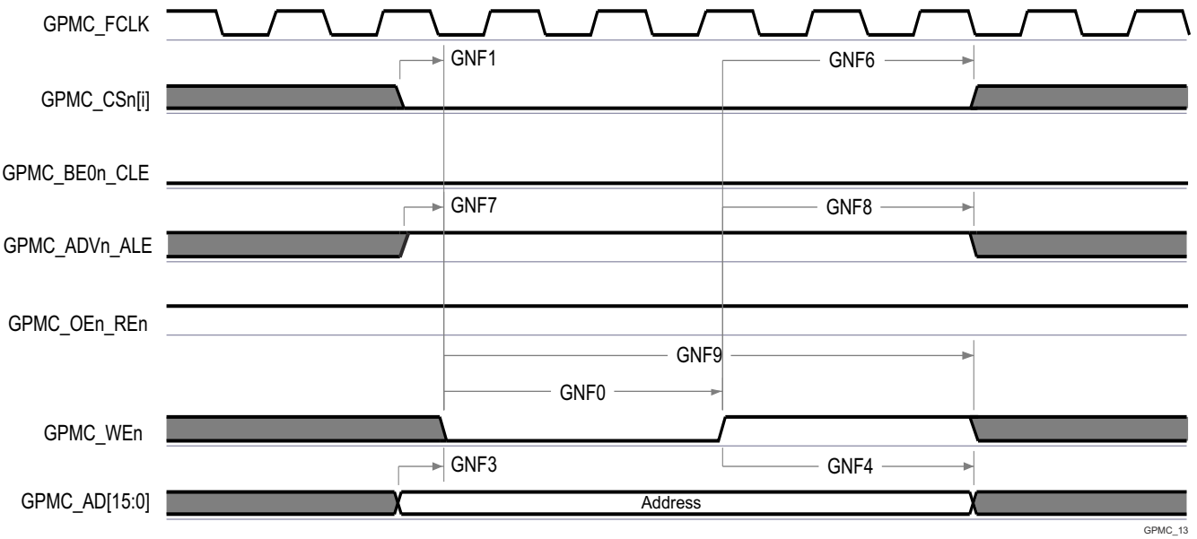
图 6-54. GPMC 和 NAND 闪存 - 地址锁存周期
