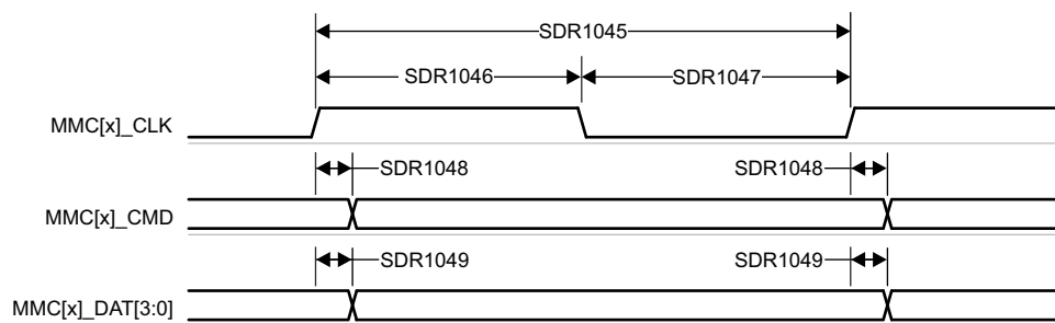
图 6-80. MMC0 - UHS-I SDR104 - 发送模式
