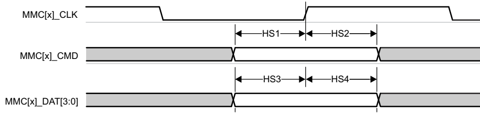
图 6-72. MMC0 - 高速 - 接收模式
