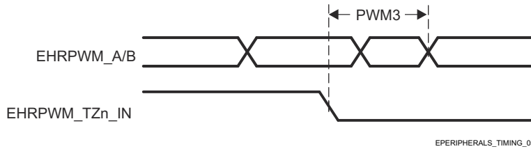
图 6-39. EHRPWM_TZn_IN 至 EHRPWM_A/B 强制开关特性
