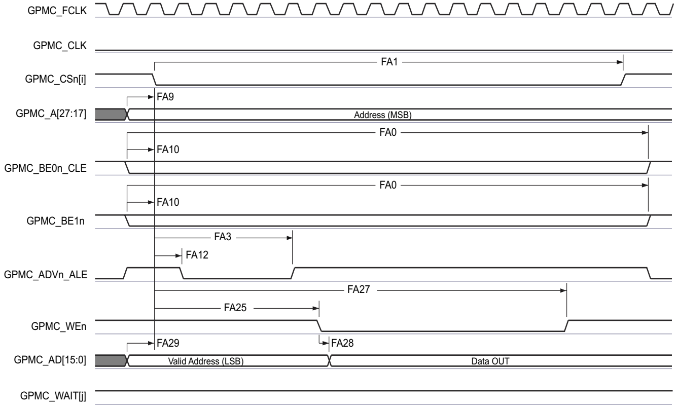
图 6-52. GPMC 和多路复用 NOR 闪存 - 异步写入 - 单字
