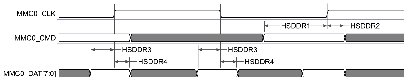
图 6-67. MMC0 - 高速 DDR 模式 - 接收模式
