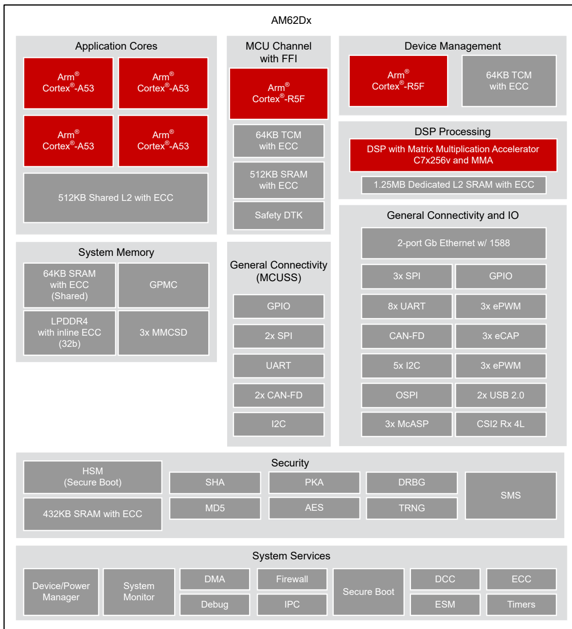
图 3-1. 功能方框图
