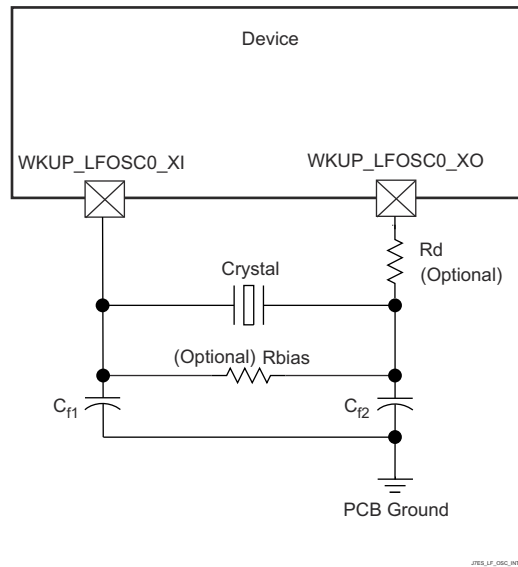
图 6-19. WKUP_LFOSC0 晶体实现
