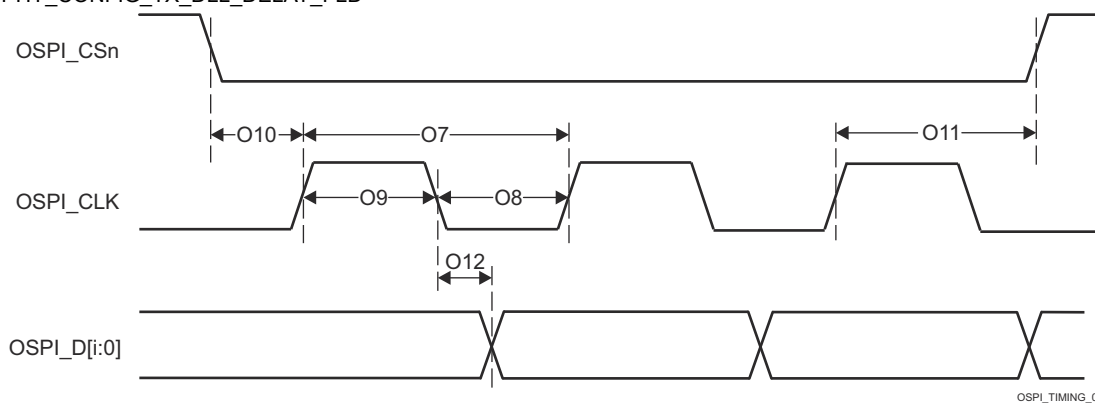
图 6-98. OSPI0 开关特性 - PHY SDR
