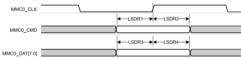
图 6-63. MMC0 - 旧 SDR - 接收模式
