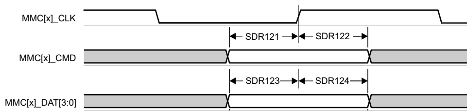
图 6-74. MMC0 - UHS-I SDR12 - 接收模式
