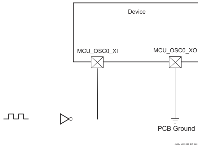
图 6-18. 与 1.8V LVCMOS 兼容的时钟输入
