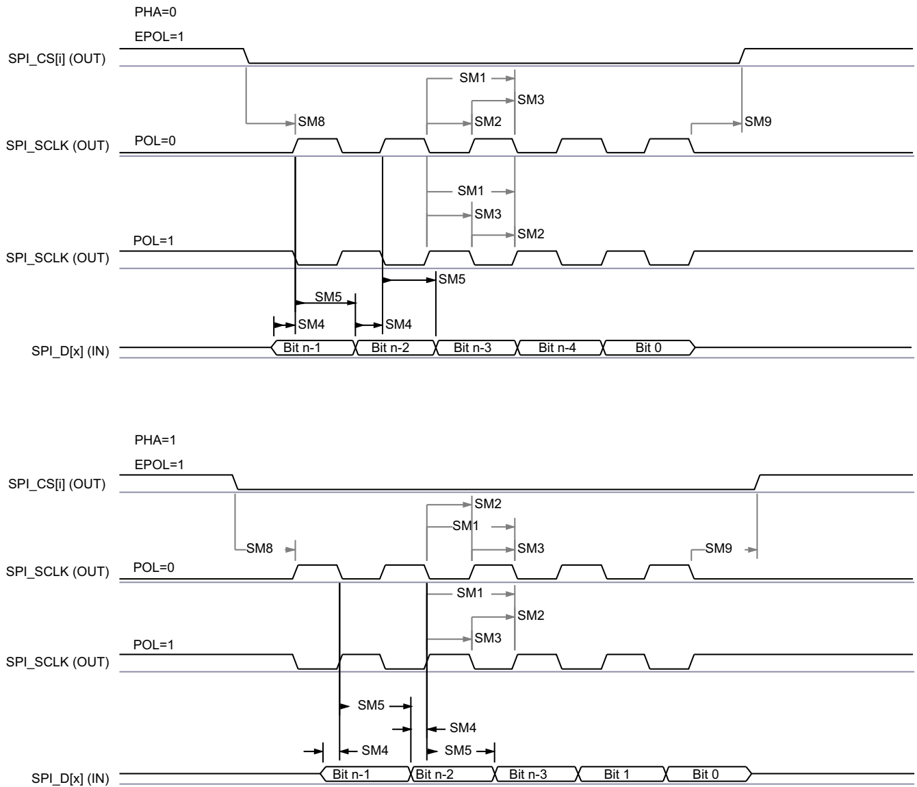
图 6-59. SPI 控制器模式接收时序
