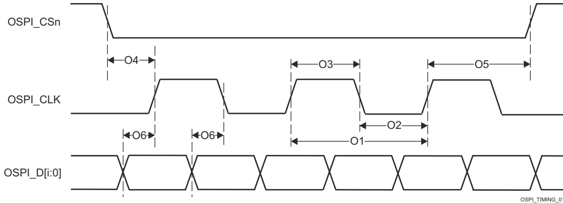
图 6-94. OSPI0 开关特性 - PHY DDR 数据训练
