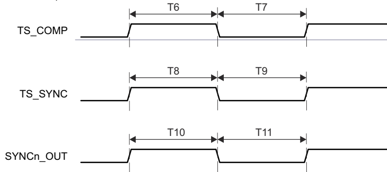
图 6-31. CPTS 开关特性
