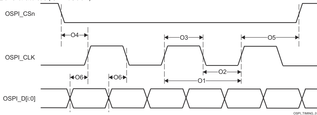
图 6-104. OSPI0 开关特性 - Tap DDR, 无环回
