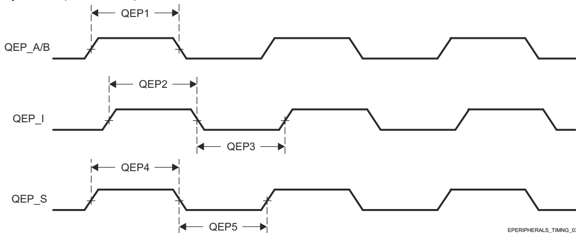
图 6-41. EQEP 时序要求
