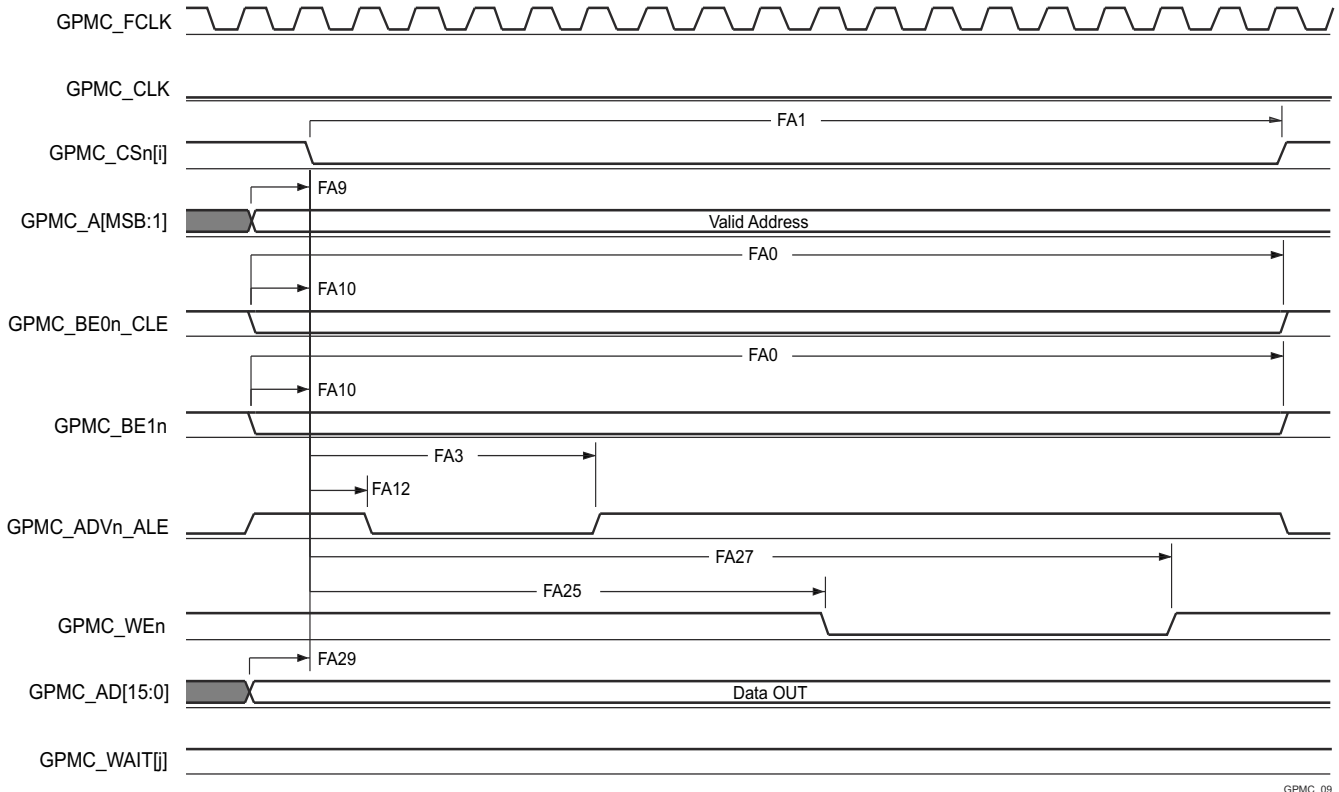
图 6-50. GPMC 和 NOR 闪存 - 异步写入 - 单字
