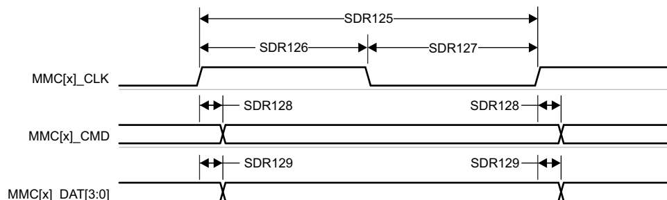
图 6-75. MMC0 - UHS-I SDR12 - 发送模式
