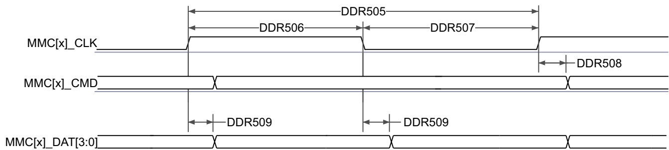
图 6-90. MMC1/MMC2 - UHS-I DDR50 - 发送模式
