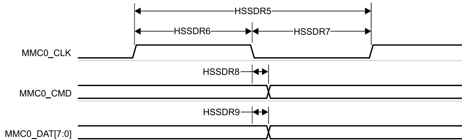
图 6-66. MMC0 - 高速 SDR 模式 - 发送模式
