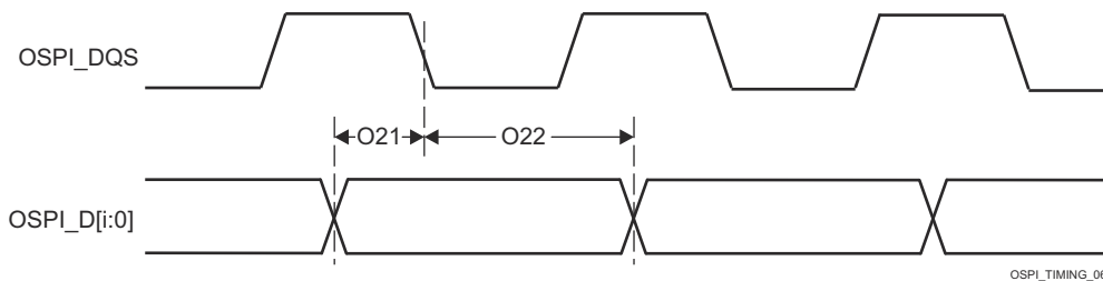
图 6-97. OSPI0 时序要求 - 具有外部电路板环回的 PHY SDR
