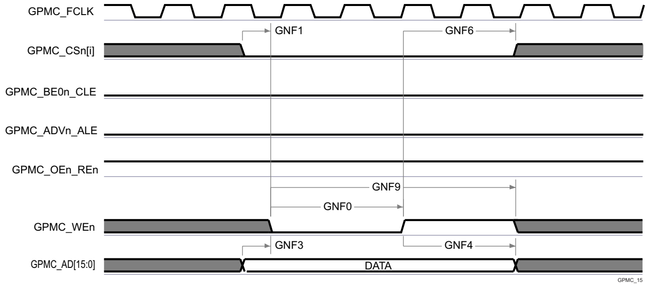
图 6-56. GPMC 和 NAND 闪存 - 数据写入周期
