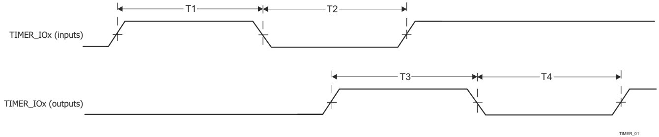
图 6-105. 计时器时序要求和开关特性
