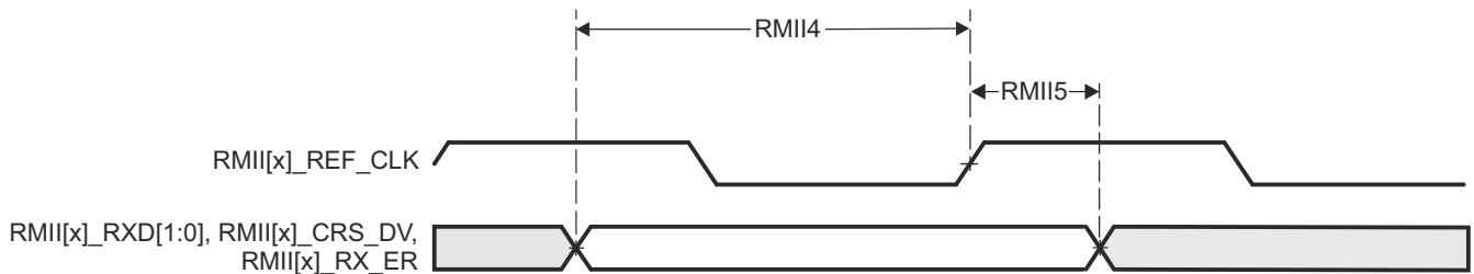
图 6-26. CPSW3G RMII[x]_RXD[1:0]、RMII[x]_CRS_DV、RMII[x]_RX_ER 时序要求 - RMII 模式
