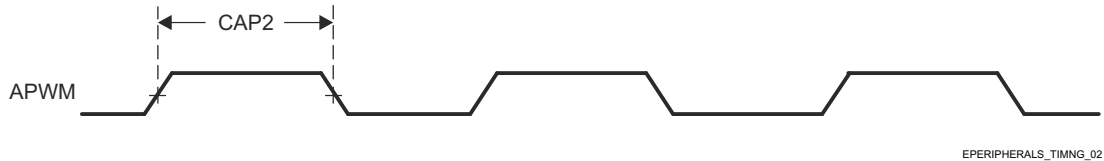
图 6-34. ECAP 开关特性
