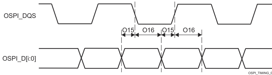
图 6-99. OSPI0 时序要求 - 具有外部电路板环回或 DQS 的 PHY DDR
