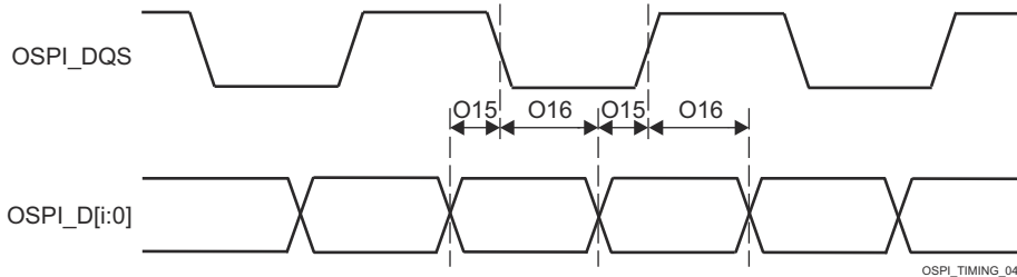
图 6-92. OSPI0 时序要求 - PHY 数据训练，带 DQS 的 DDR
