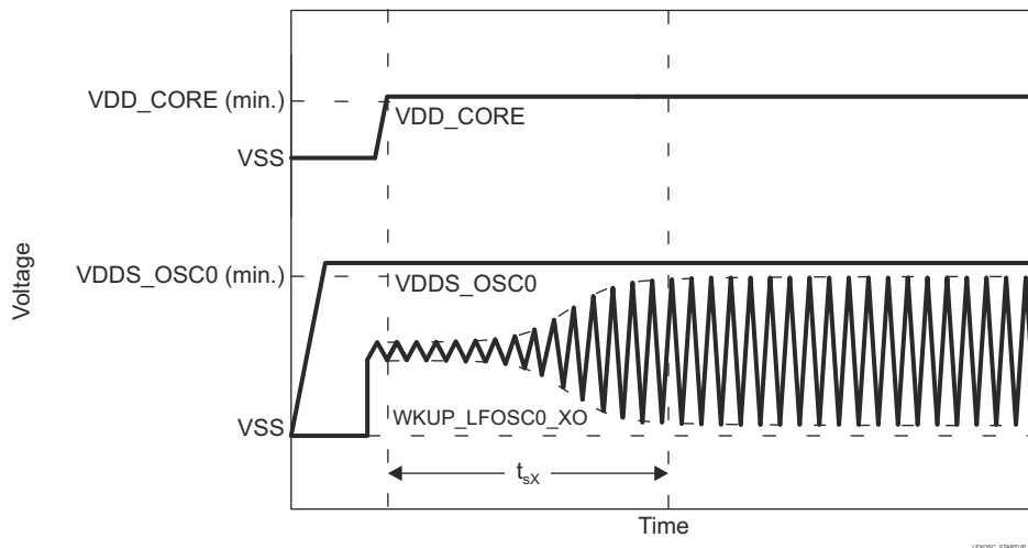
图 6-21. WKUP_LFOSC0 启动时间
