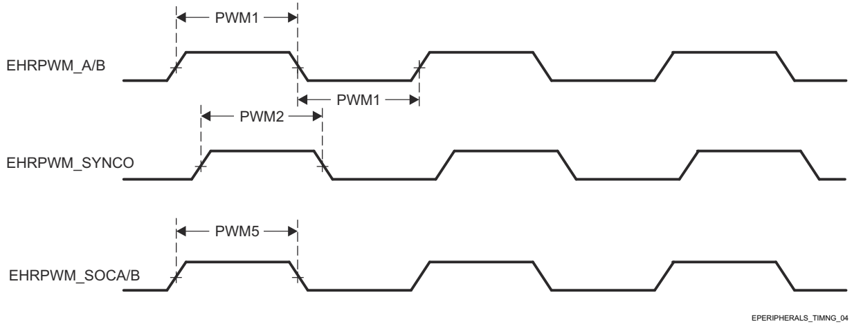
图 6-38. EHRPWM 开关特性
