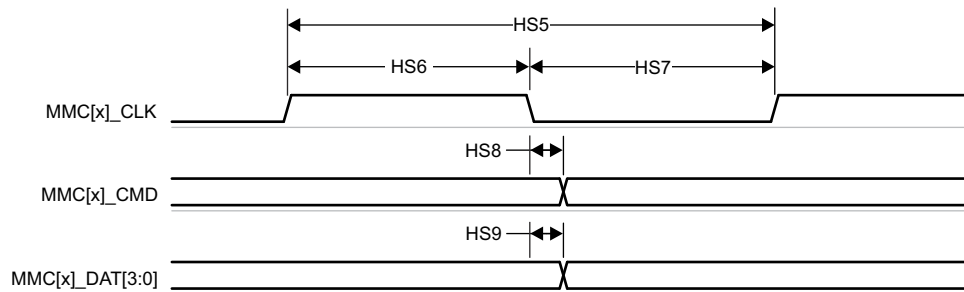
图 6-73. MMC0 - 高速 - 发送模式
