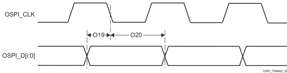
图 6-96. OSPI0 时序要求 - 具有内部 PHY 环回的 PHY SDR
