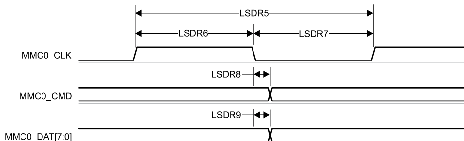
图 6-64. MMC0 - 旧 SDR - 发送模式
