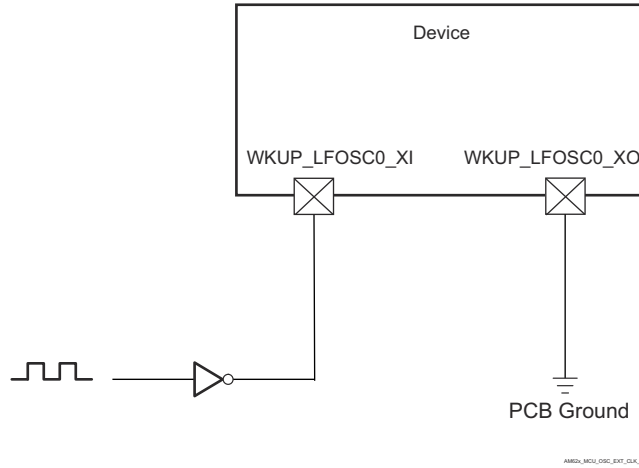
图 6-22. 与 1.8V LVCMOS 兼容的时钟输入
