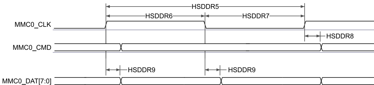
图 6-68. MMC0 - 高速 DDR 模式 - 发送模式
