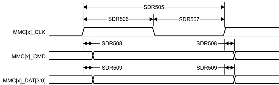
图 6-89. MMC1/MMC2 - UHS-I SDR50 - 发送模式
