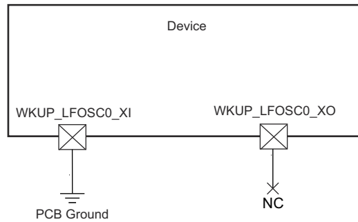
图 6-23. 未使用 WKUP_LFOSC0
