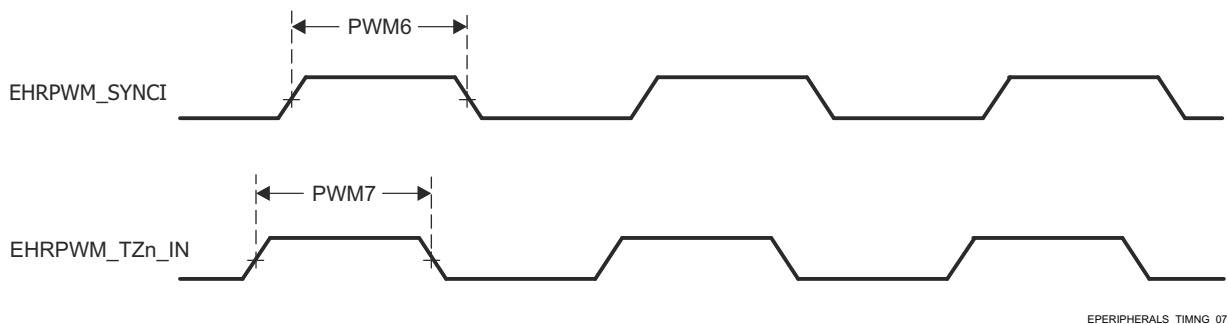
图 6-37. EPWM 时序要求
