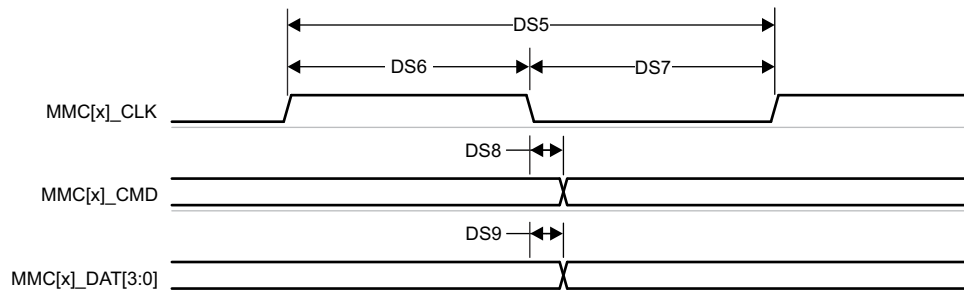
图 6-82. MMC1/MMC2 - 默认速度 - 发送模式
