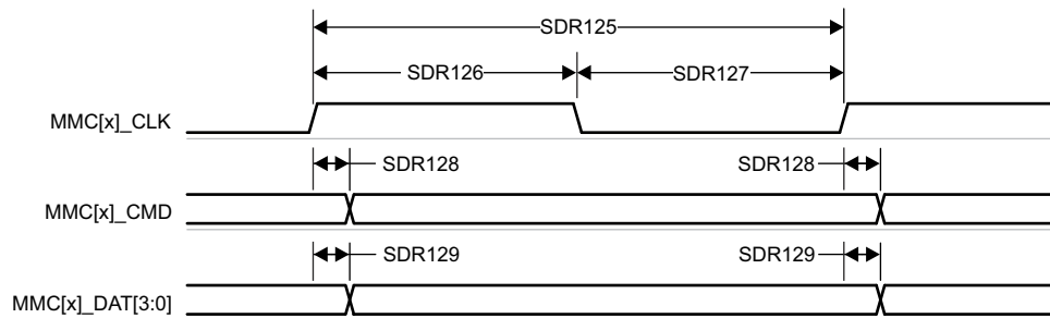
图 6-86. MMC1/MMC2 - UHS-I SDR12 - 发送模式
