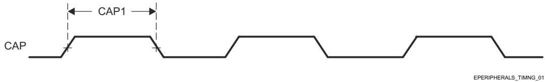
图 6-33. ECAP 时序要求
