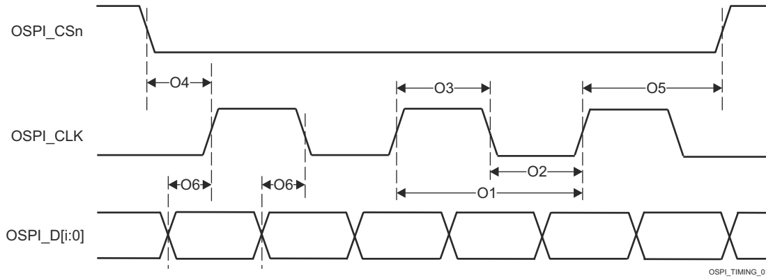
图 6-100. OSPI0 开关特性 - PHY DDR
