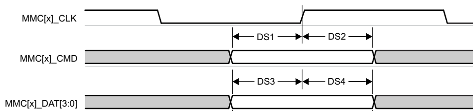
图 6-70. MMC0 - 默认速度 - 接收模式
