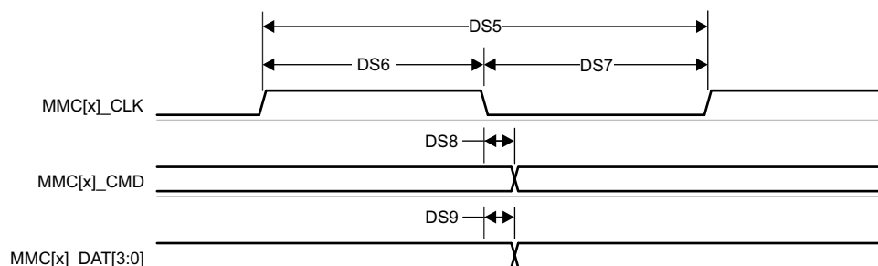
图 6-71. MMC0 - 默认速度 - 发送模式
