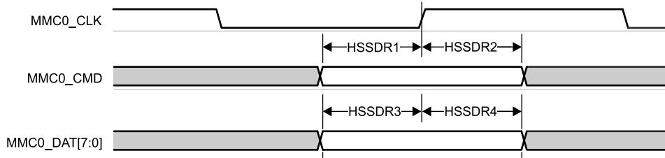
图 6-65. MMC0 - 高速 SDR 模式 - 接收模式
