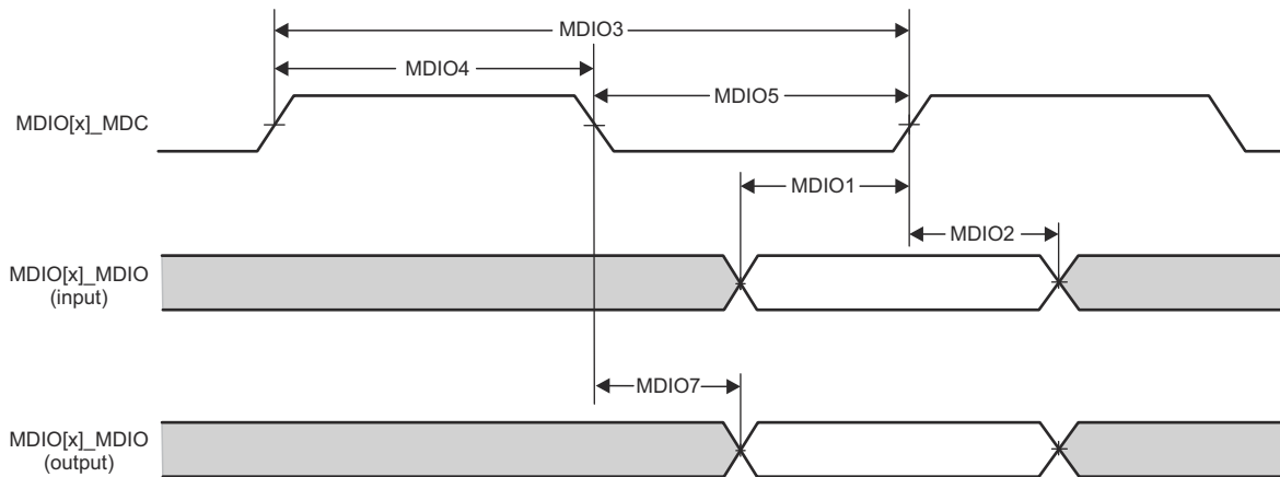
图 6-24. CPSW3G MDIO 时序要求和开关特性
