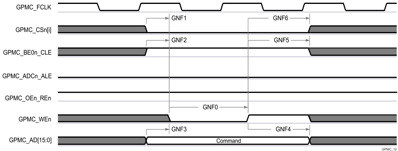
图 6-53. GPMC 和 NAND 闪存 - 命令锁存周期
