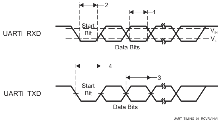
图 6-106. UART 时序要求和开关特性
