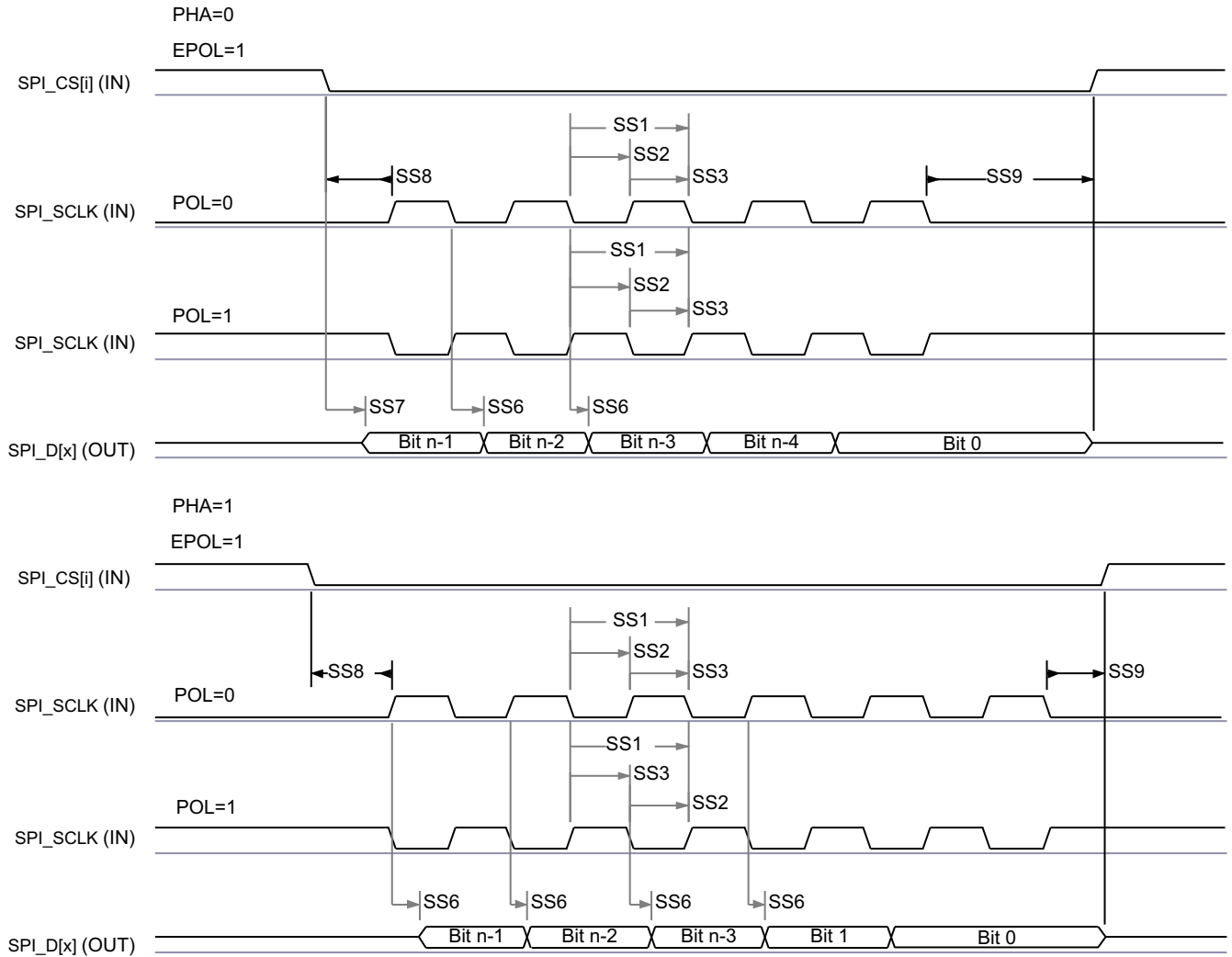
图 6-62. SPI 外设模式发送时序
