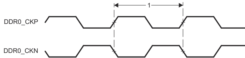
图 6-32. DDRSS 开关特性
