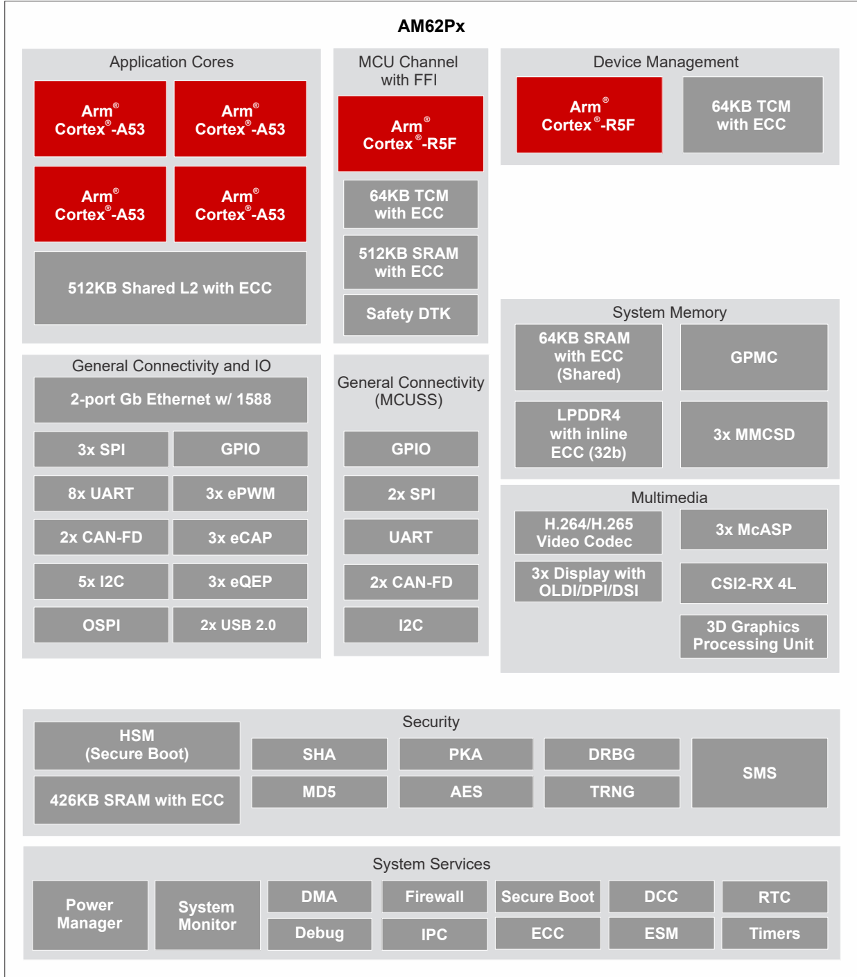
图 3-1. 功能方框图
