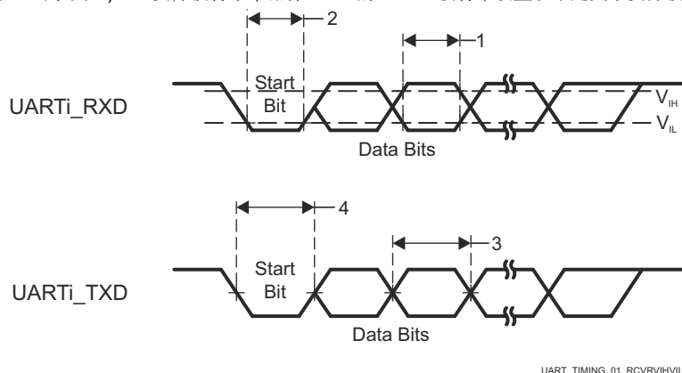
图 6-102. UART 时序要求和开关特性
