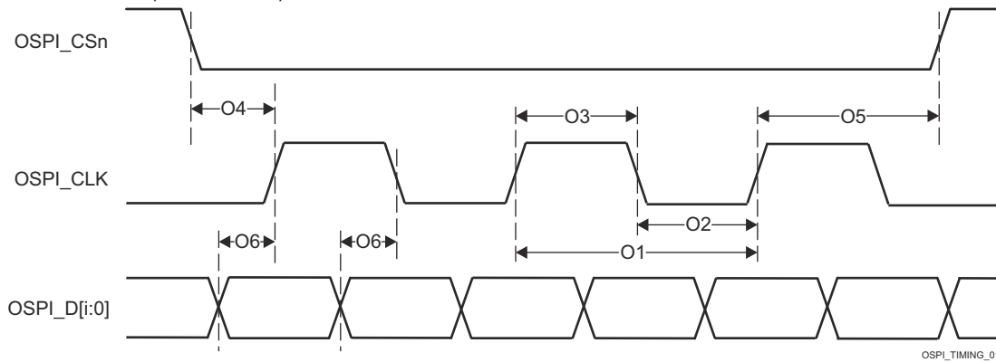
图 6-100. OSPI0 开关特性 - Tap DDR, 无环回
