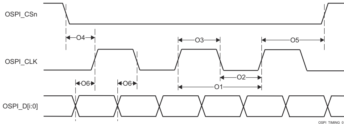
图 6-90. OSPI0 开关特性 - PHY DDR 数据训练
