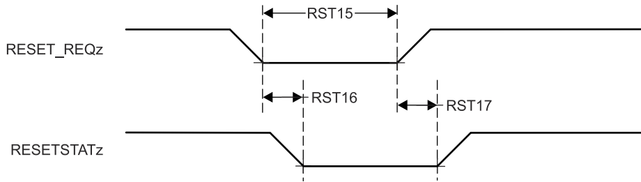
图 6-10. RESET_REQz 和 RESETSTATz 时序要求和开关特性
