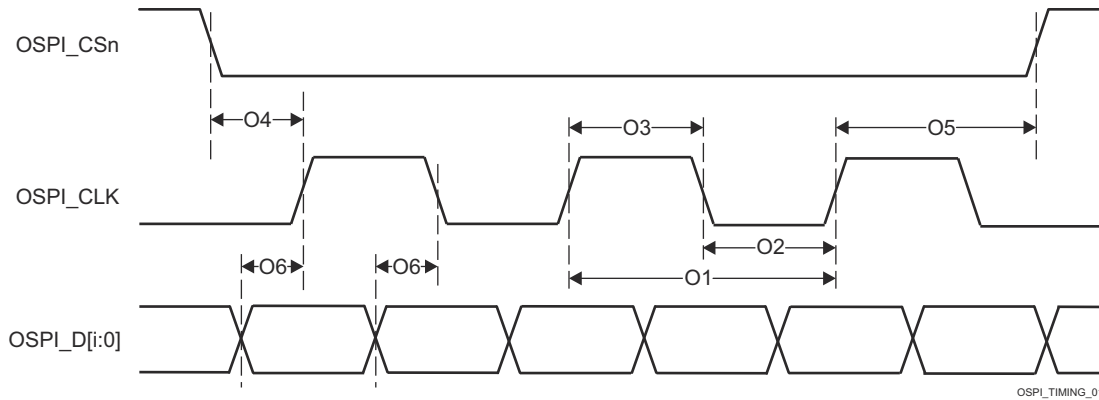
图 6-90. OSPI 开关特性 - PHY DDR 数据训练
