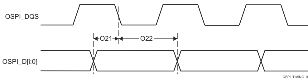
图 6-93. OSPI0 时序要求 - 具有外部电路板环回的 PHY SDR
