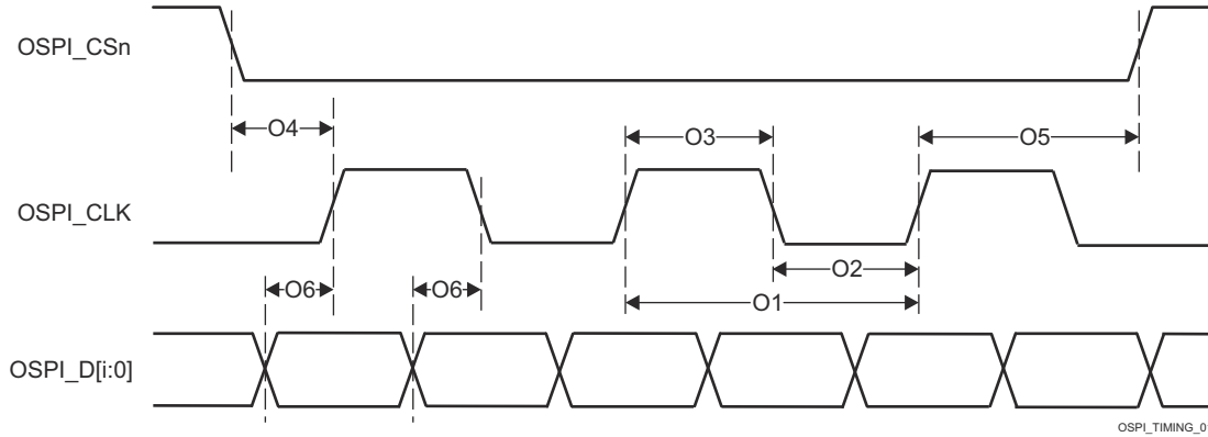
图 6-96. OSPI0 开关特性 - PHY DDR
