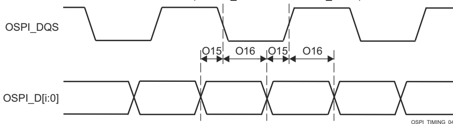
图 6-95. OSPI0 时序要求 - 具有外部电路板环回或 DQS 的 PHY DDR
