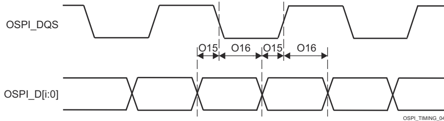
图 6-88. OSPI0 时序要求 – PHY 数据训练，带 DQS 的 DDR
