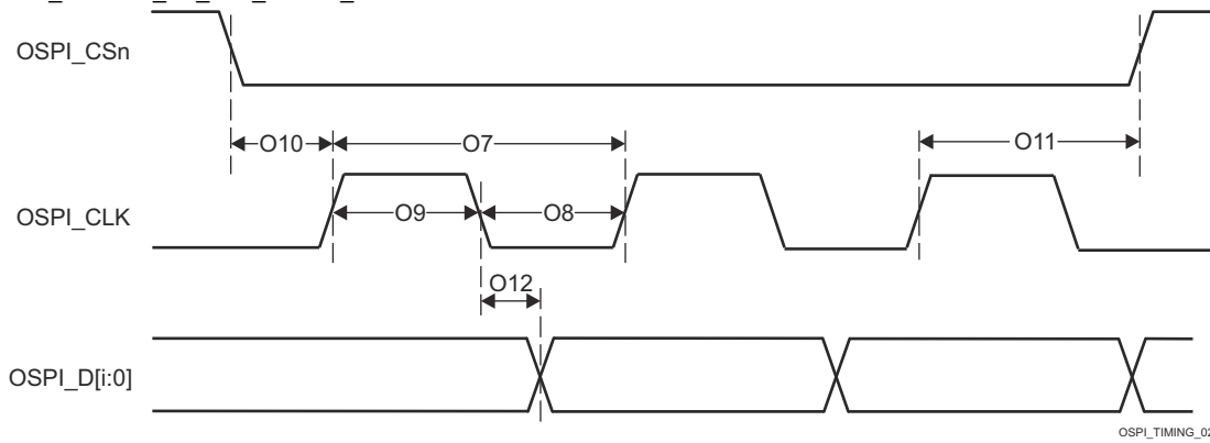
图 6-94. OSPI0 开关特性 - PHY SDR
