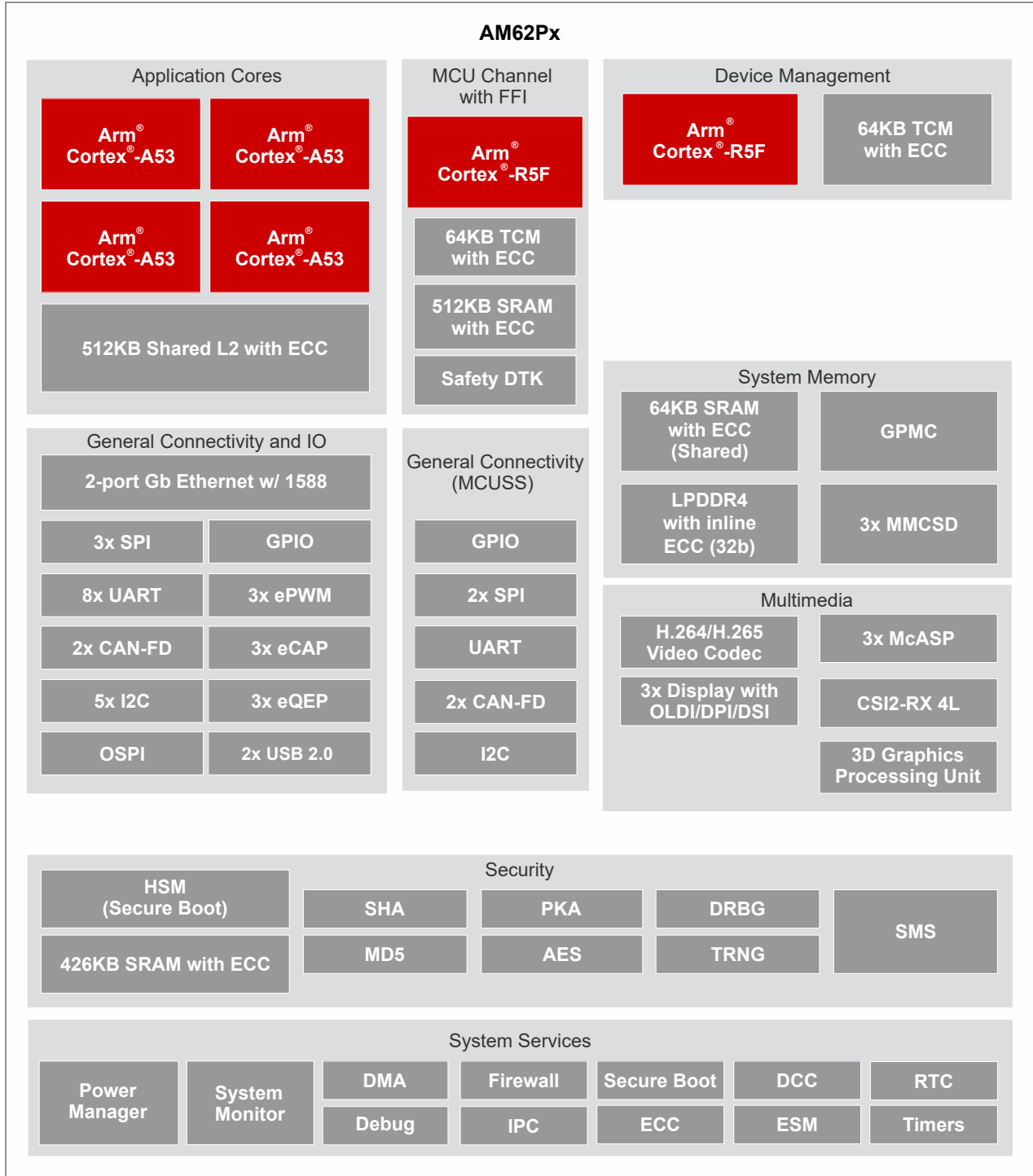
图 3-1. 功能方框图
