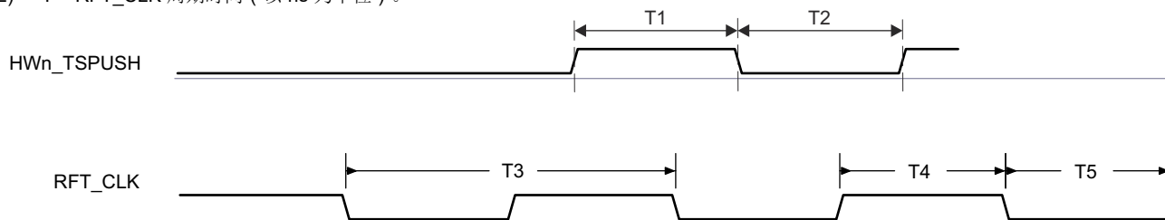
图 6-32. CPTS 时序要求
