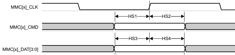
图 6-78. MMC1/MMC2 - 高速 - 接收模式
