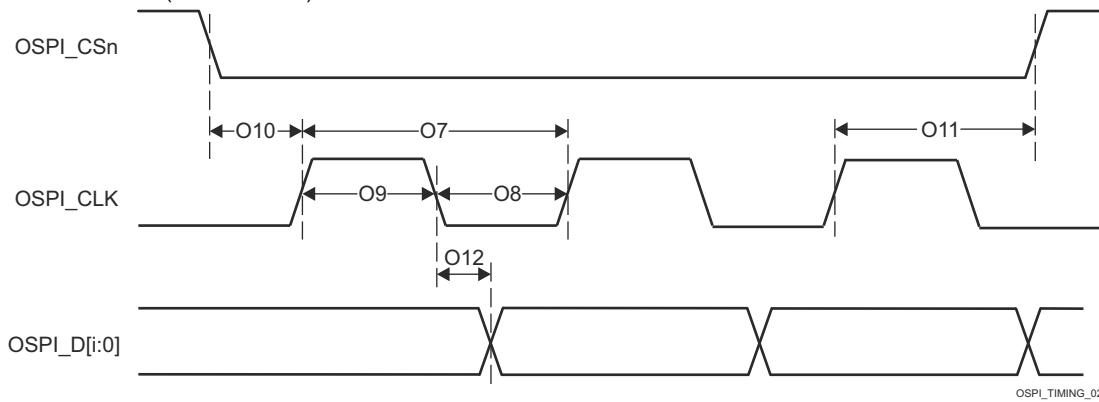
图 6-98. OSPI0 开关特性 - Tap SDR, 无环回
