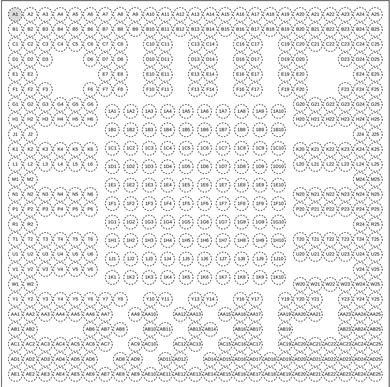
图 5-1. AMH FCBGA 封装 (顶视图)
