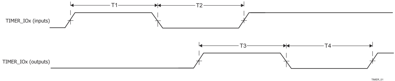
图 6-101. 计时器时序要求和开关特性
