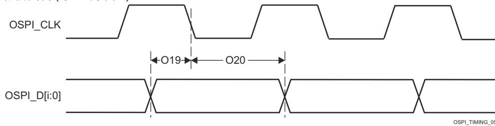
图 6-97. OSPI0 时序要求 - Tap SDR，无环回
