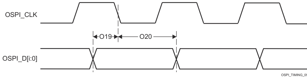
图 6-92. OSPI0 时序要求 - 具有内部 PHY 环回的 PHY SDR
