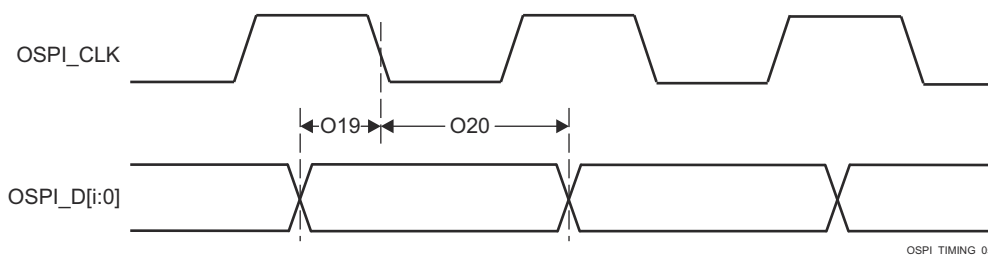
图 6-92. OSPI0 时序要求 - 具有内部 PHY 环回的 PHY SDR
