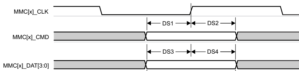
图 6-76. MMC1/MMC2 - 默认速度 - 接收模式
