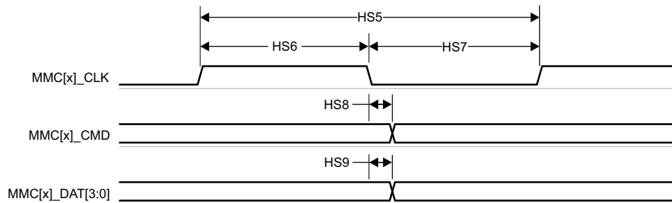
图 6-79. MMC1/MMC2 - 高速 - 发送模式
