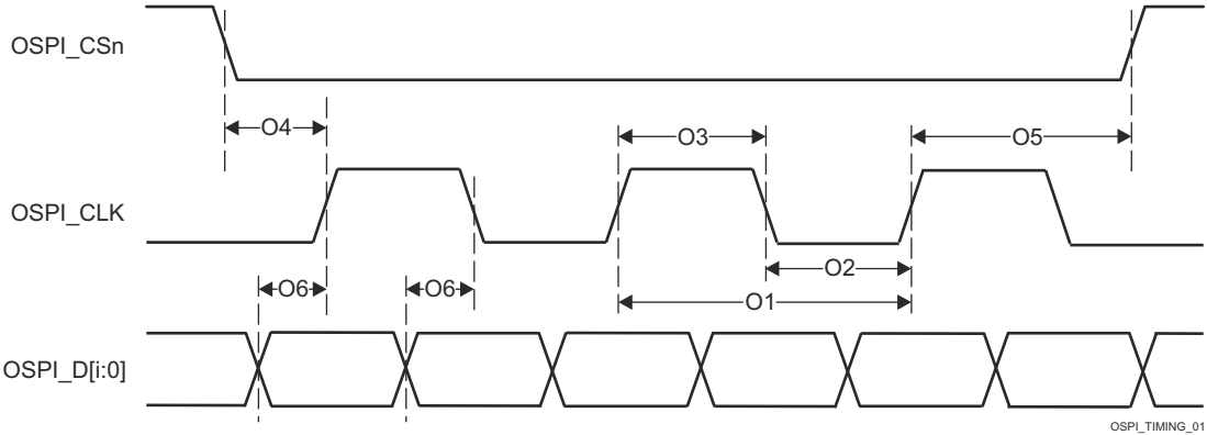
图 6-80. OSPI0 开关特性 - PHY DDR 数据训练
