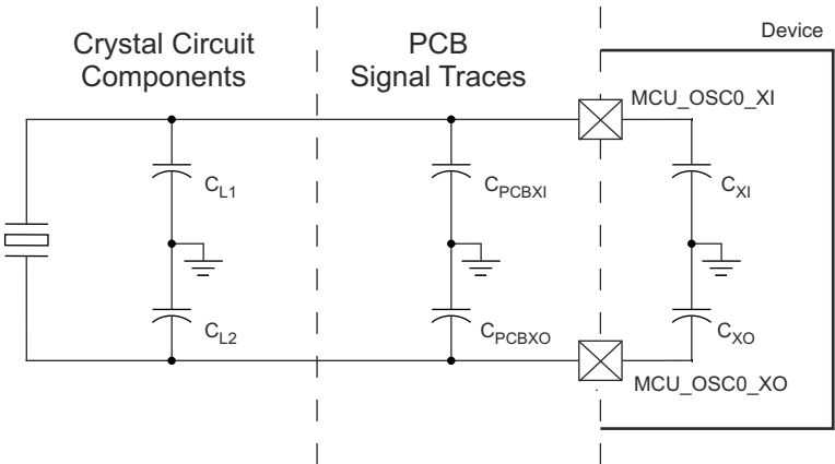
图 6-19. 负载电容
