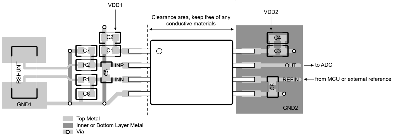
图 8-7. AMC0x00R-Q1 的建议布局
