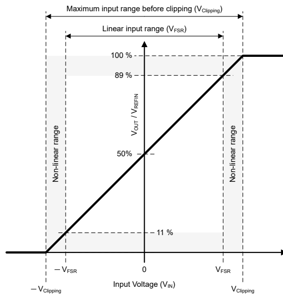
图 7-3. AMC0x00R-Q1 的输入到输出传送曲线
