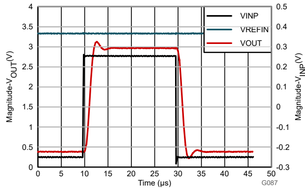
图 8-4. AMC0x00R-Q1 的输出阶跃响应
