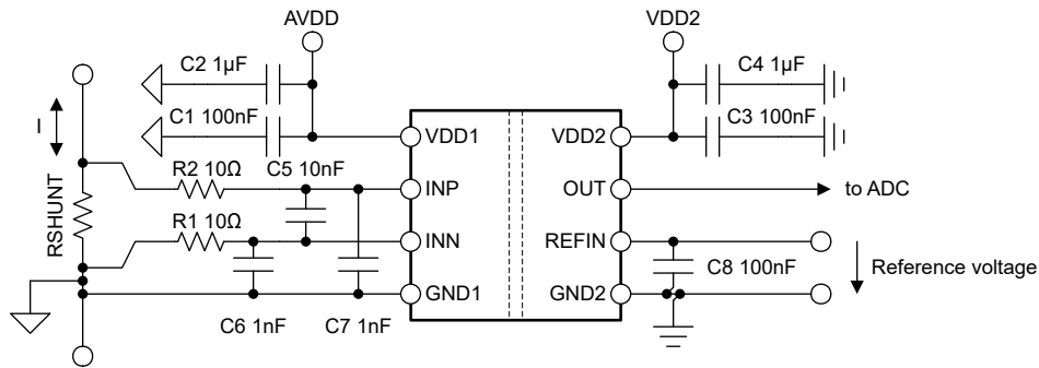
图 8-6. AMC0x00R-Q1 去耦
