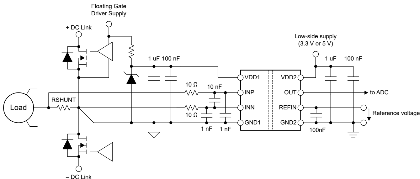
图 8-1. 在典型应用中使用 AMC0x00R-Q1 进行电流检测
