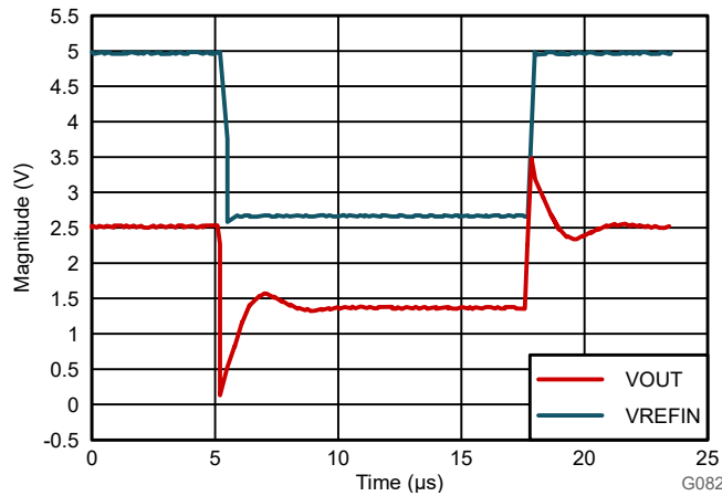
图 8-5. AMC0x00R-Q1 的参考输入阶跃响应
