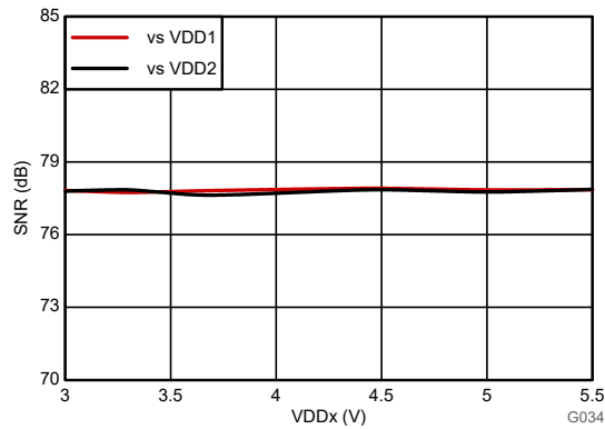
图 6-30. 信噪比与电源电压间的关系
