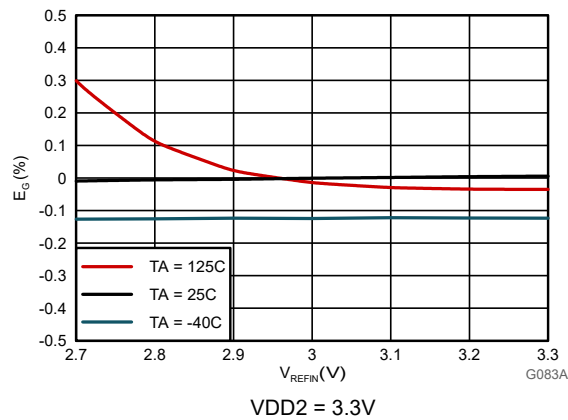
图 6-12. 增益误差与 VREFIN 间的关系
