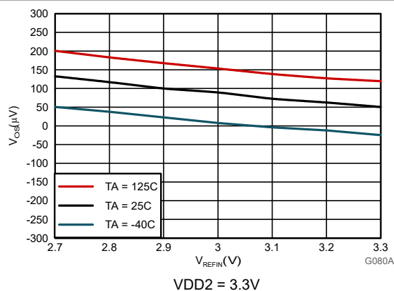
图 6-10. 输入偏移电压与 VREFIN 间的关系
