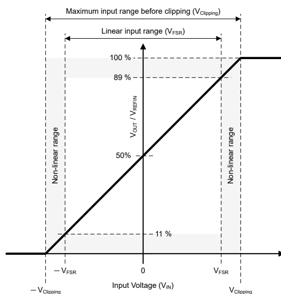
图 7-3. AMC0x02R-Q1 的输入到输出传送曲线
