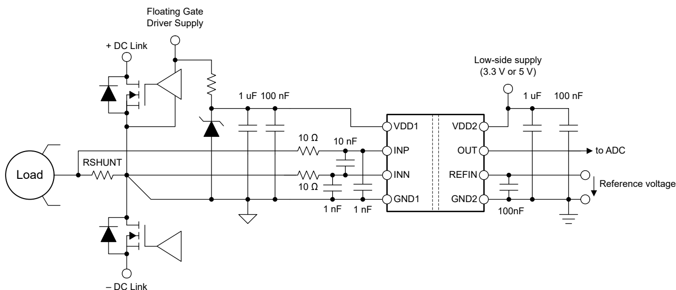
图 8-1. 在典型应用中使用 AMC0x02R-Q1 进行电流检测
