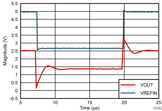
图 8-5. AMC0x02R-Q1 的参考输入阶跃响应
