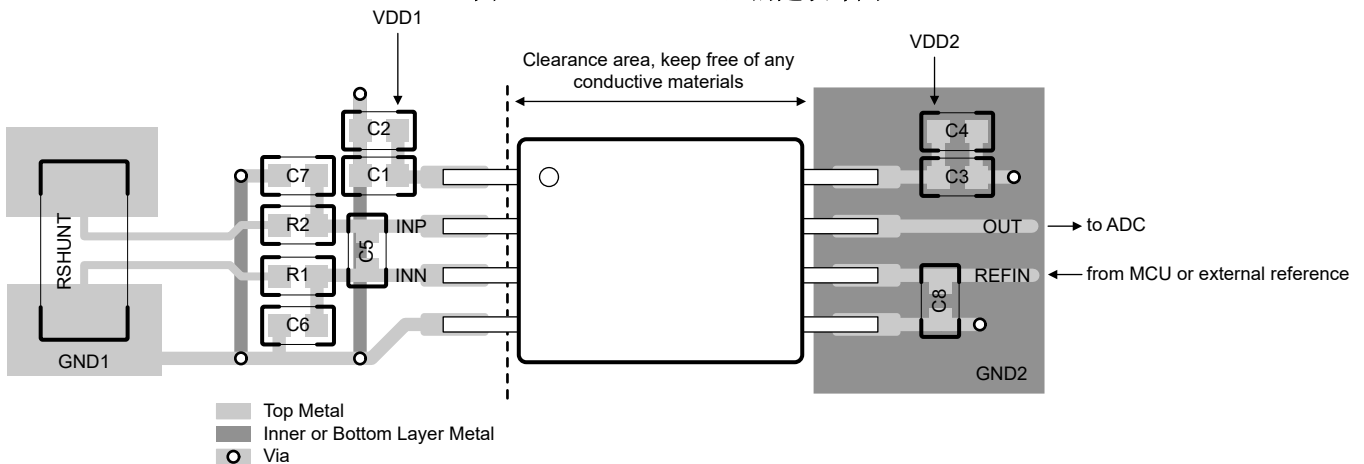
图 8-7. AMC0x02R-Q1 的建议布局
