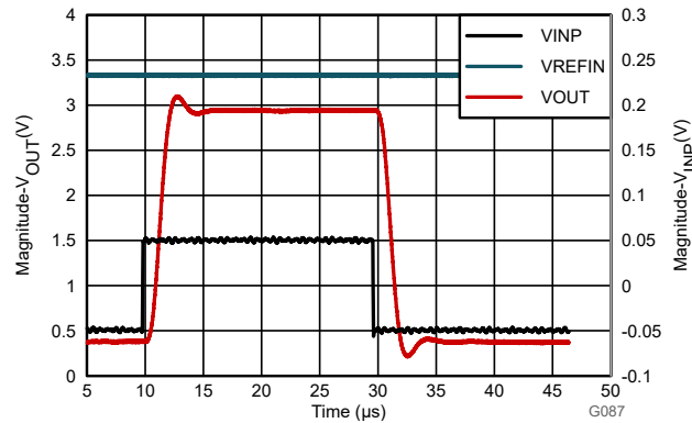
图 8-4. AMC0x02R-Q1 的输出阶跃响应
