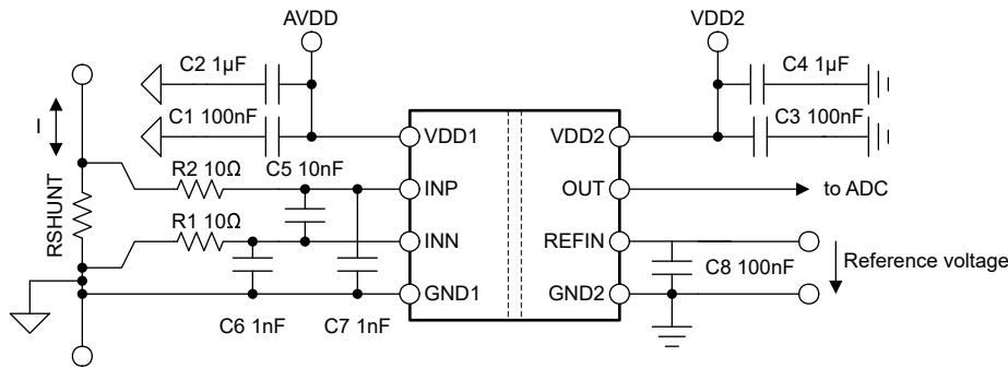
图 8-6. AMC0x02R-Q1 去耦
