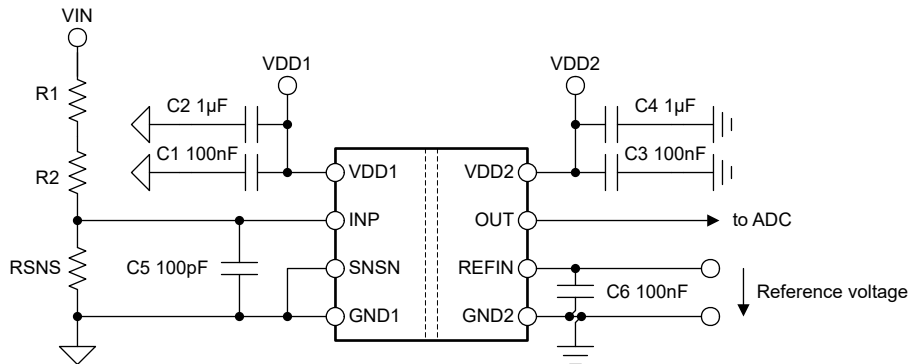
图 8-5. AMC0x11S 去耦
